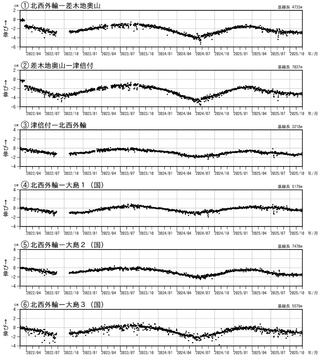
図 3-2 伊豆大島 GNSS 連続観測による基線長変化 (2022 年 3 月～2025 年 11 月)
