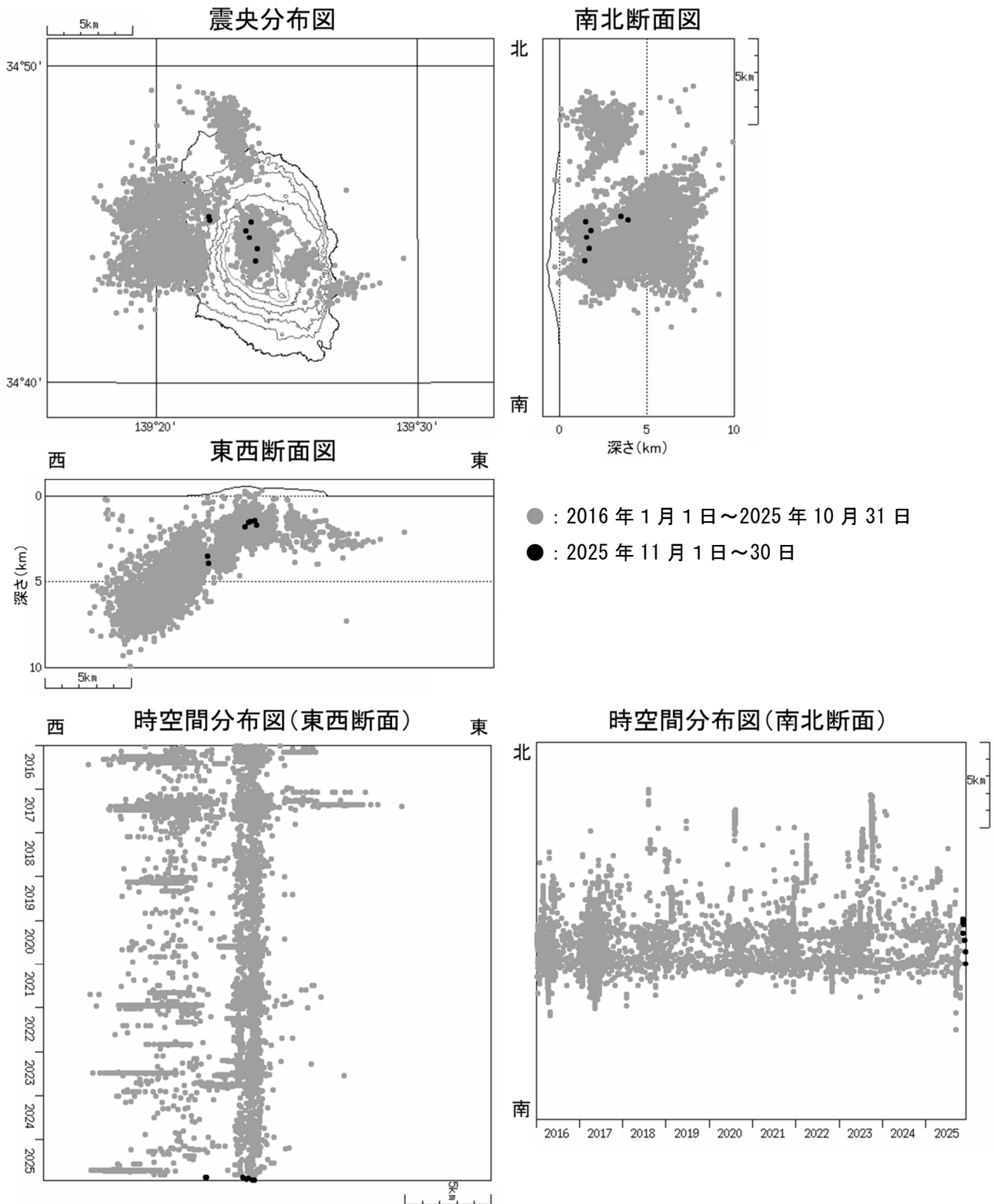
図4 伊豆大島 震源分布図（2016 年 1 月 1 日～2025 年 11 月 30 日）
