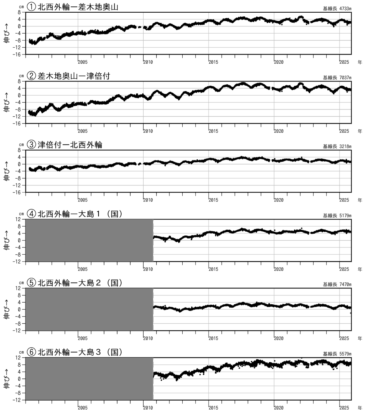
図3-1 伊豆大島 GNSS 連続観測による基線長変化(2001年1月～2025年11月)
