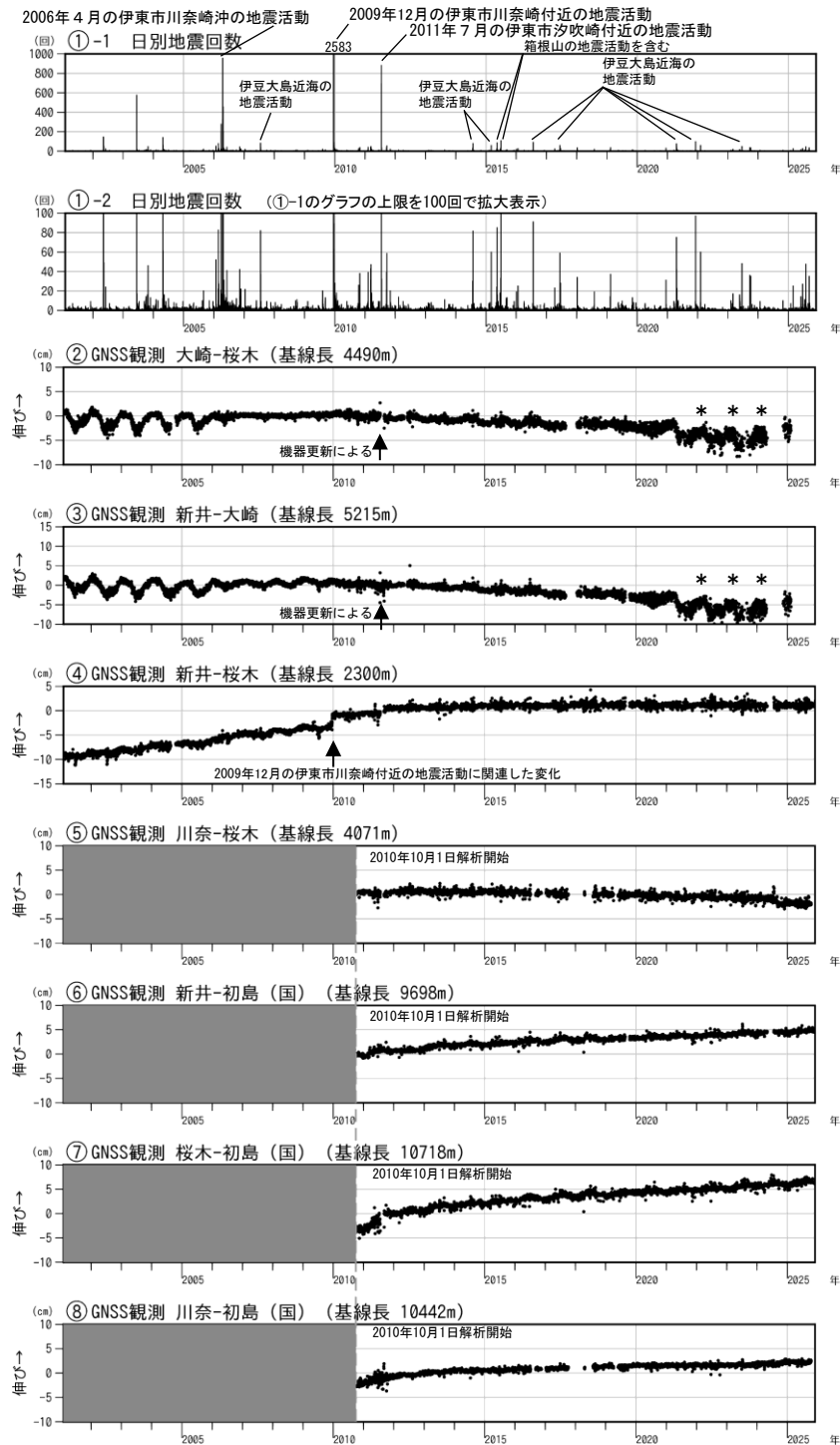
図3 伊豆東部火山群 火山活動経過図（2001年2月1日～2025年11月30日）
