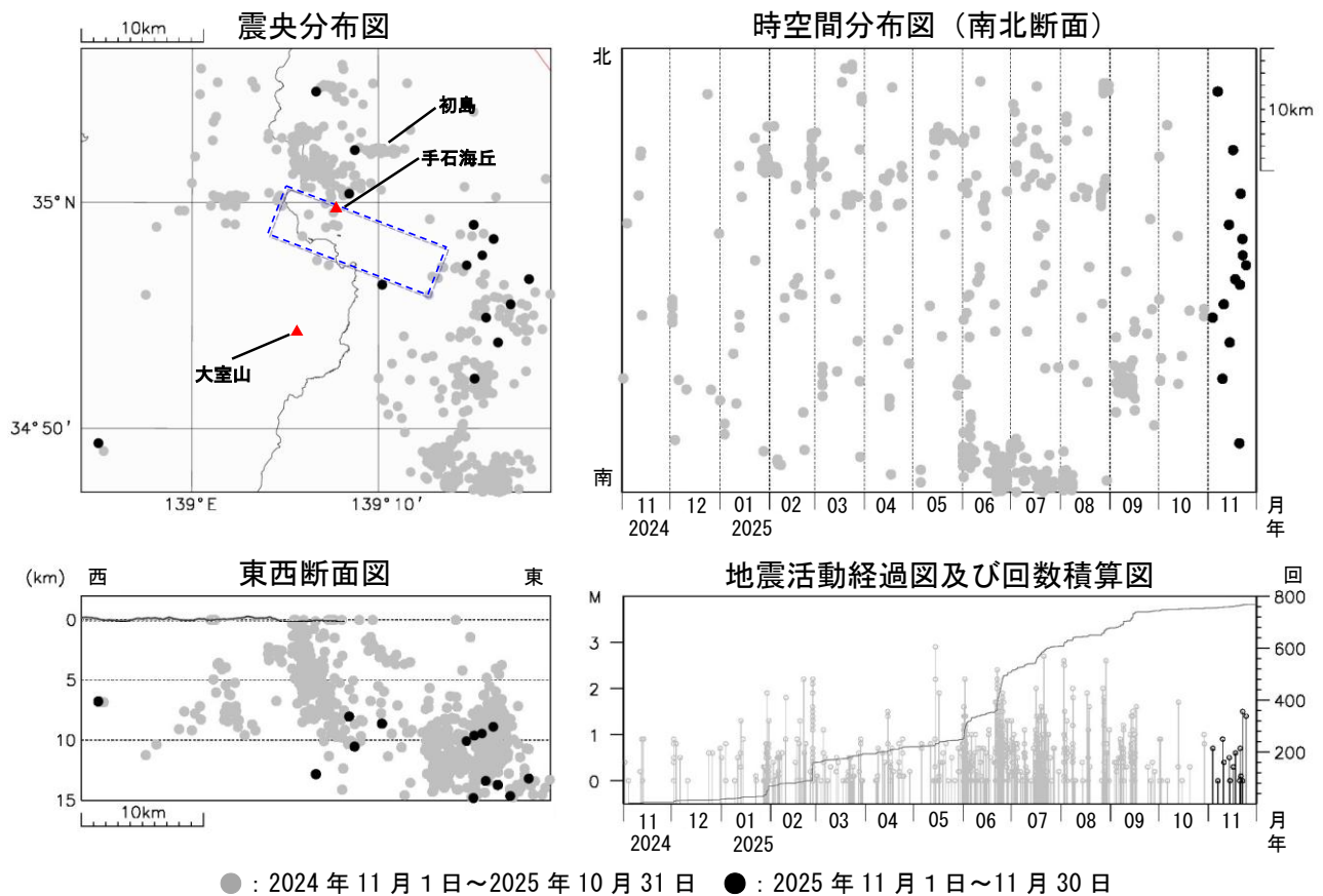
図2 伊豆東部火山群 広域地震観測網による震源分布図（2024 年 11 月 1 日～2025 年 11 月 30 日） □ の領域は群発地震活動の発生する可能性がある範囲（火口が出現する可能性のある範囲）を示しています。 https://www.data.jma.go.jp/vois/data/filing/level/PDF/level_316.pdf 広域地震観測網により震源決定したもので、深さは全て海面以下として決定しています。 M（マグニチュード）は地震の規模を表し、M0.0 以上を表示しています。 図中の震源要素は一部暫定値が含まれており、後日変更することがあります。 この図では、関係機関の地震波形を一元的に処理し、地震観測点の標高を考慮する等した手法で得られた震源を用いています。
