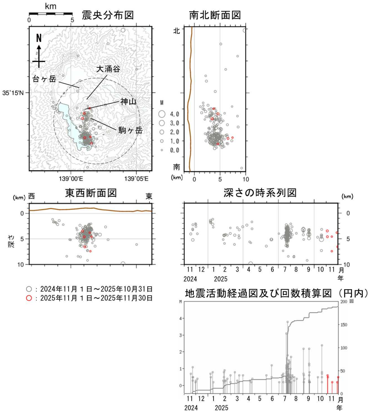
図4 箱根山 広域地震観測網による山体周辺の震源分布図（2024年11月1日～2025年11月30日）
