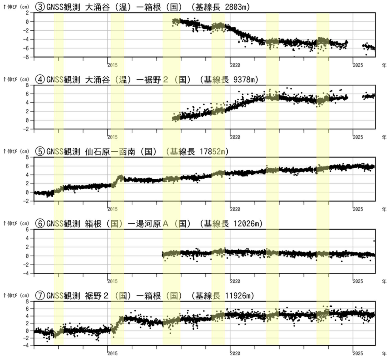
図3-2 箱根山 GNSS連続観測による 基線長変化及び観測点配置図 (2012年1月1日～2025年11月30日) (国)：国土地理院 (温)：神奈川県温泉地学研究所 空白部分は欠測を示します。 システム更新に伴う調整中のため、一部の 過去データにステップ状の変化がみ られています。
