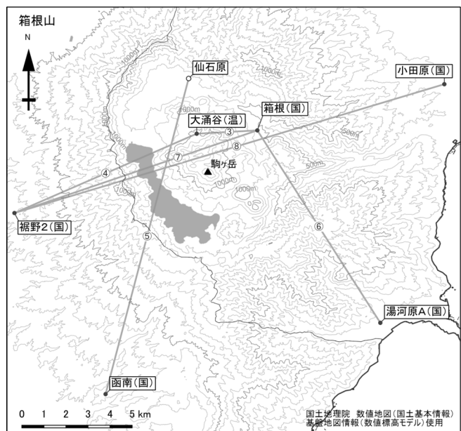
図3-2 箱根山 GNSS連続観測による 基線長変化及び観測点配置図 (2012年1月1日～2025年11月30日) (国)：国土地理院 (温)：神奈川県温泉地学研究所 空白部分は欠測を示します。 システム更新に伴う調整中のため、一部の 過去データにステップ状の変化がみ られています。
