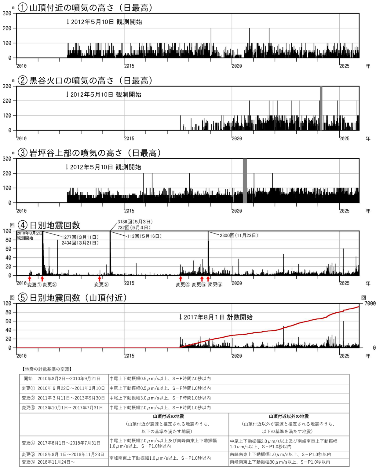
図5 焼岳 噴気の高さと地震回数の推移(2010年8月2日～2025年11月30日) ②黒谷火口の噴気の高さは、2024年2月5日から3月14日にかけて、障害のため欠測（灰色の期間）。 ③岩坪谷上部の噴気の高さは、2020年7月7日から9月10日にかけて、障害のため欠測（灰色の期間）。 ④2017年8月1日以降、山頂付近の地震と山頂付近以外の地震を分けて計数していますが、④ではこれらを合計した回数を示しています。図中の赤矢印は計数基準の変更を示しています。 ⑤山頂付近の日別地震回数（左軸）と日別地震回数の積算（右軸）を示しています。 ・黒谷火口では、2017年夏頃から噴気が時々観測されるようになり、2019年夏頃から噴気を観測する日が増えました。
