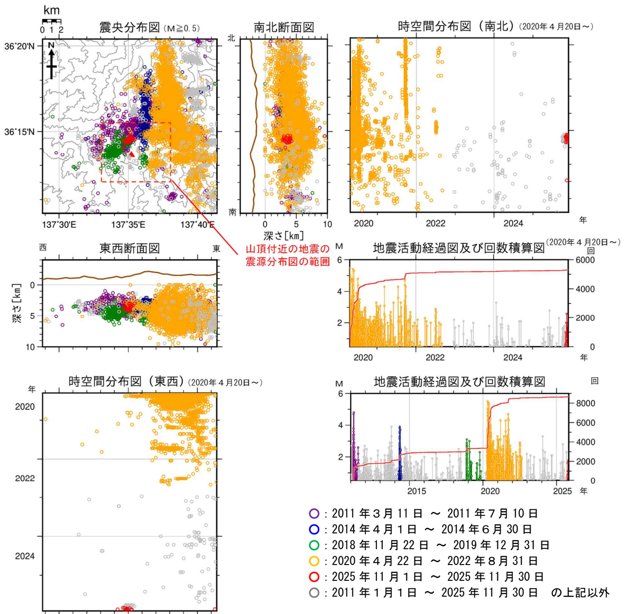
図9 焼岳 広域地震観測網による山体及び周辺の地震活動(2011年1月1日~2025年11月30日)
