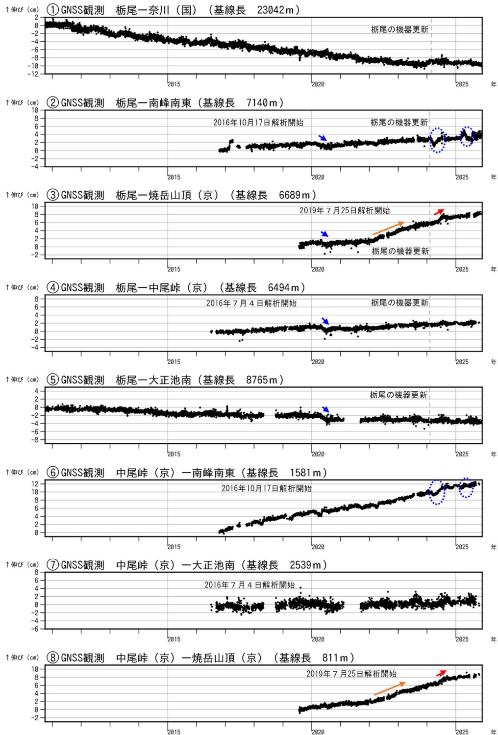
図6 焼岳 GNSS 連続観測による基線長変化（2010年10月1日～2025年11月30日）
