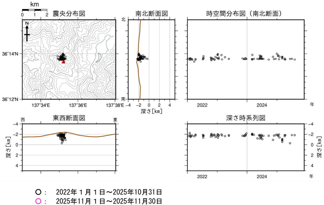
図2 焼岳 山頂付近の地震の震源分布図（2022年1月1日～2025年11月30日）
