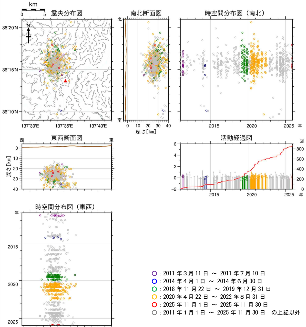
図10 焼岳 広域地震観測網による深部低周波地震の震源分布図（2011年1月1日～2025年11月30日）
