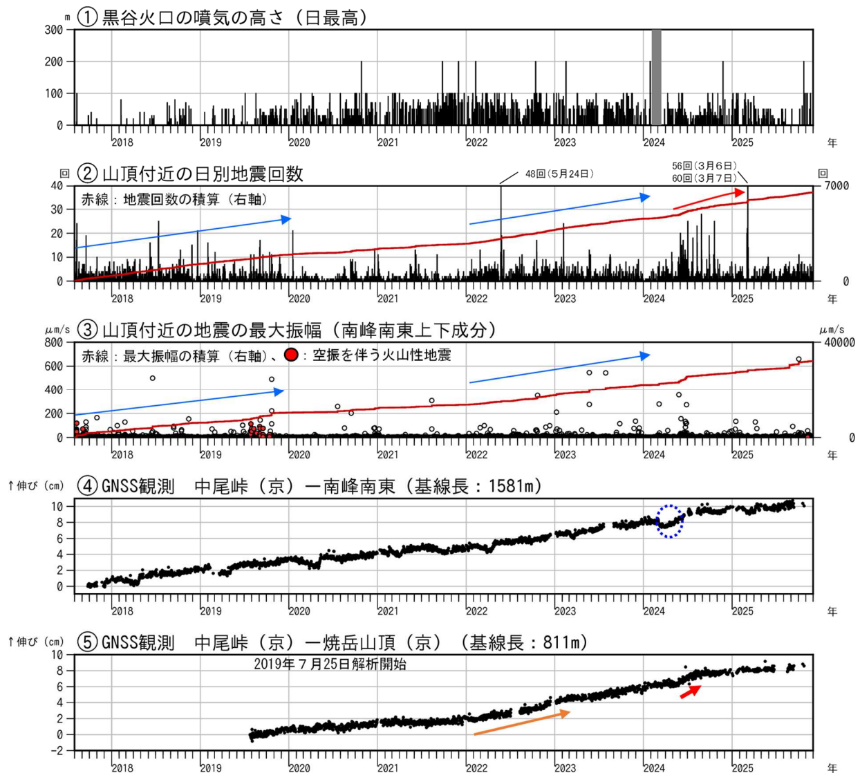
図1 焼岳 火山活動経過図（2017年8月1日～2025年11月30日）
