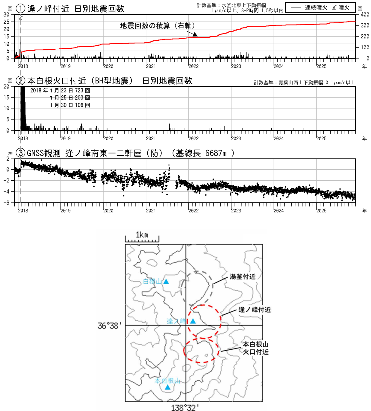
図 15 草津白根山（本白根山） 火山活動経過図（2017年12月1日～2025年11月30日）
