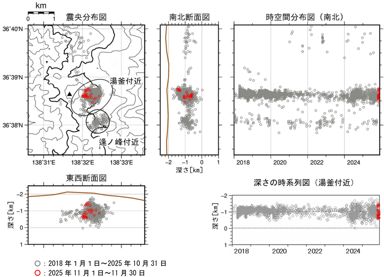
図4 草津白根山 震源分布図（2018年1月1日～2025年11月30日）
