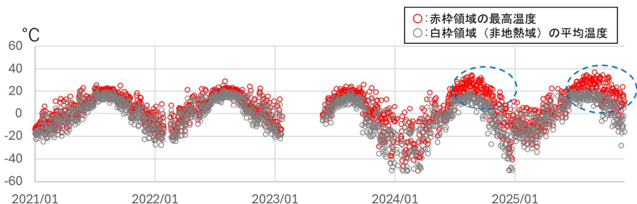
図 1－6 草津白根山（白根山（湯釜付近）） 水釜北東の地熱域の状況 (2021 年 1 月 1 日～2025 年 11 月 30 日)
