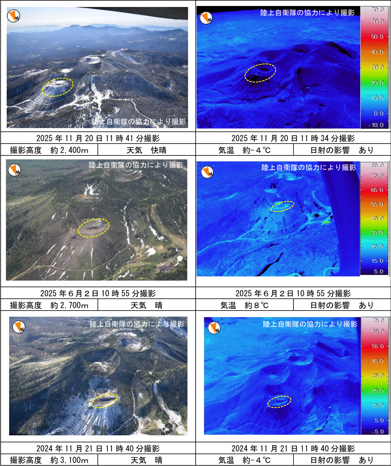
図 14－2 草津白根山（本白根山） 本白根山周辺付近の状況
