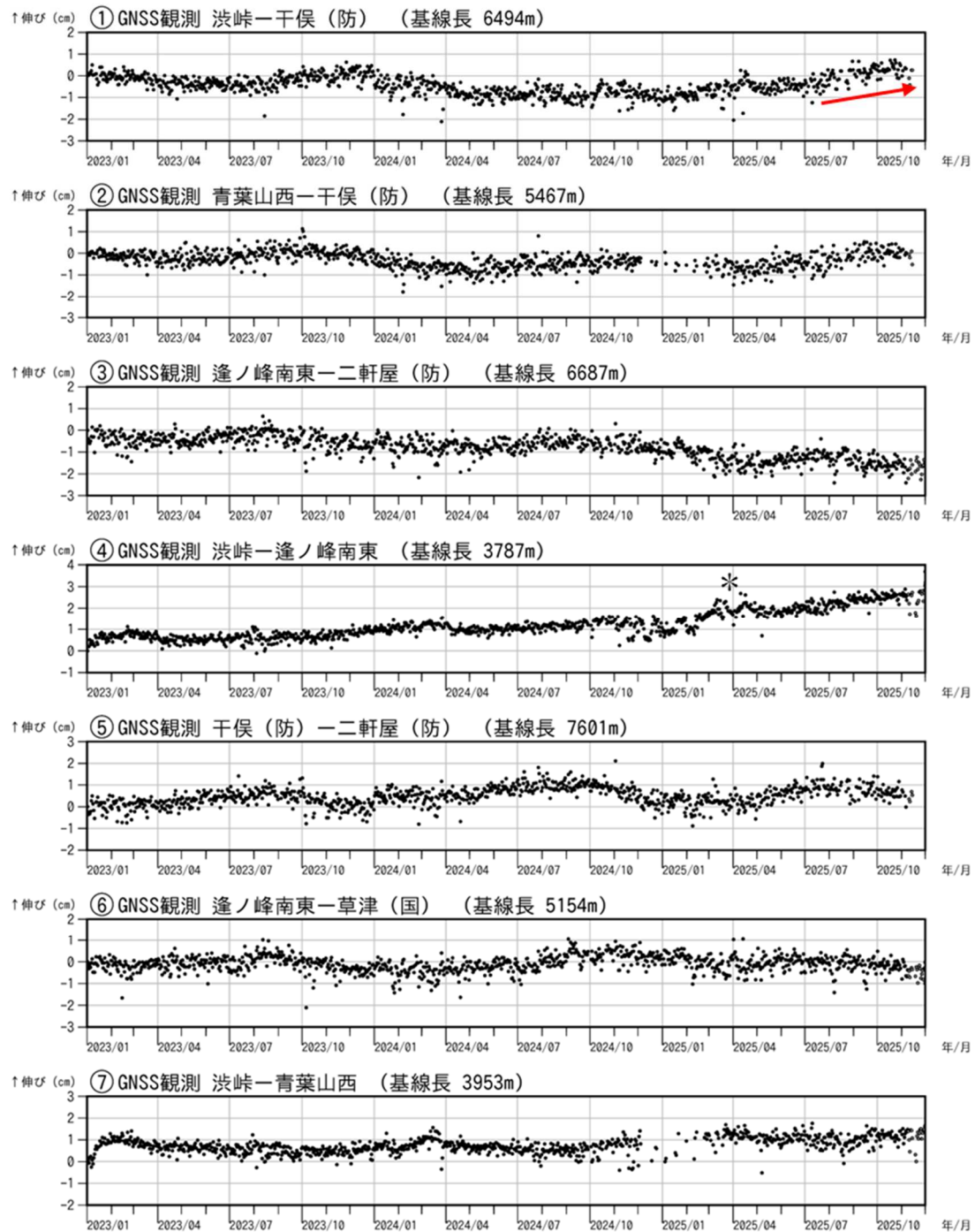
図7-2 草津白根山 GNSS 連続観測結果（2023年1月1日～2025年11月30日）
