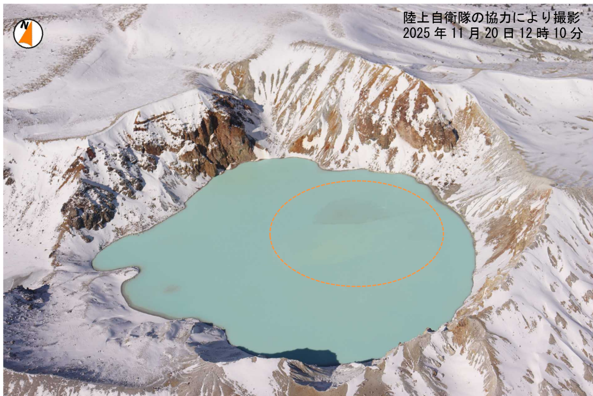
図1－3 草津白根山（白根山（湯釜付近）） 湯釜火口内の状況
