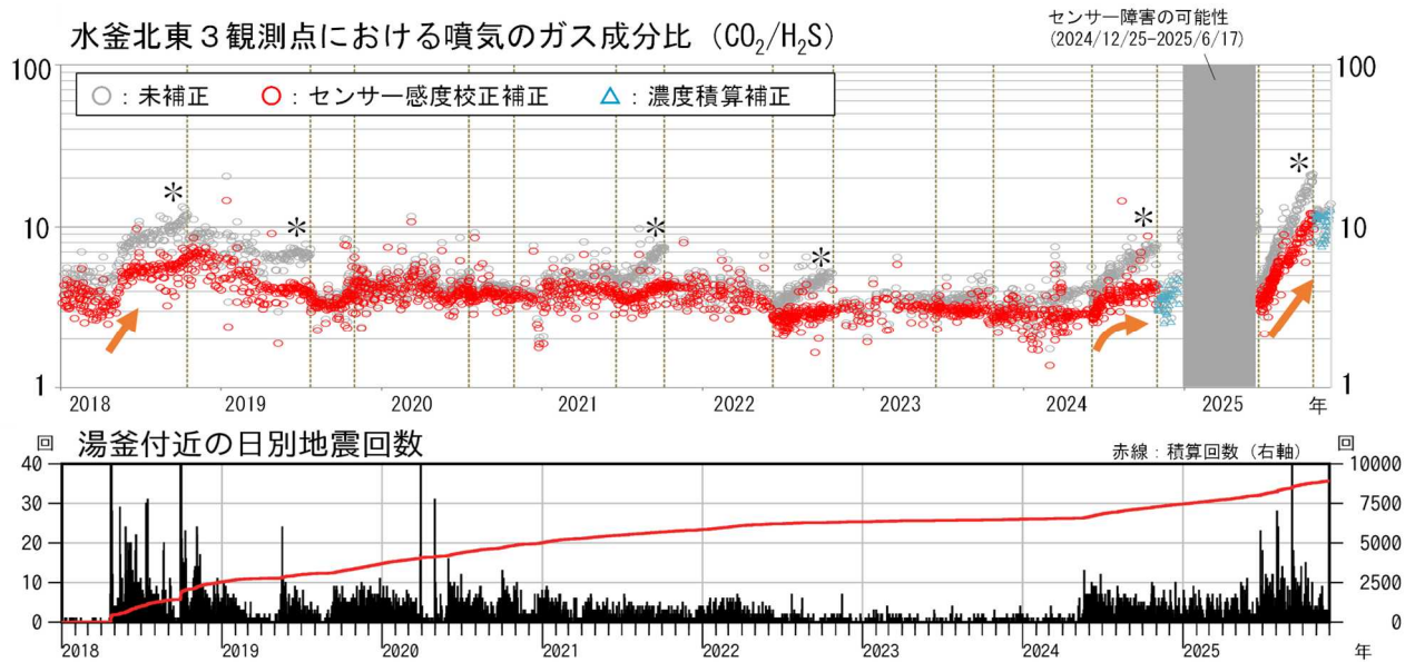
図2 草津白根山（白根山（湯釜付近）） 火山ガス観測結果（2018年1月～2025年11月30日）
