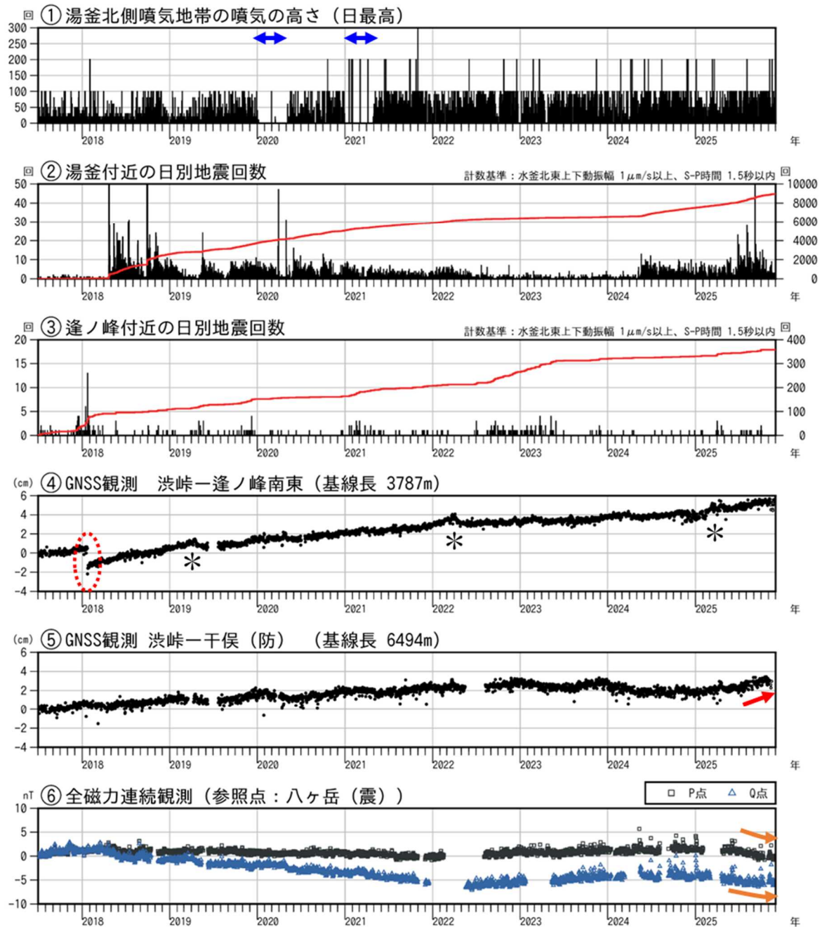
図9 草津白根山（白根山（湯釜付近）） 火山活動経過図（2017年7月1日～2025年11月30日）
