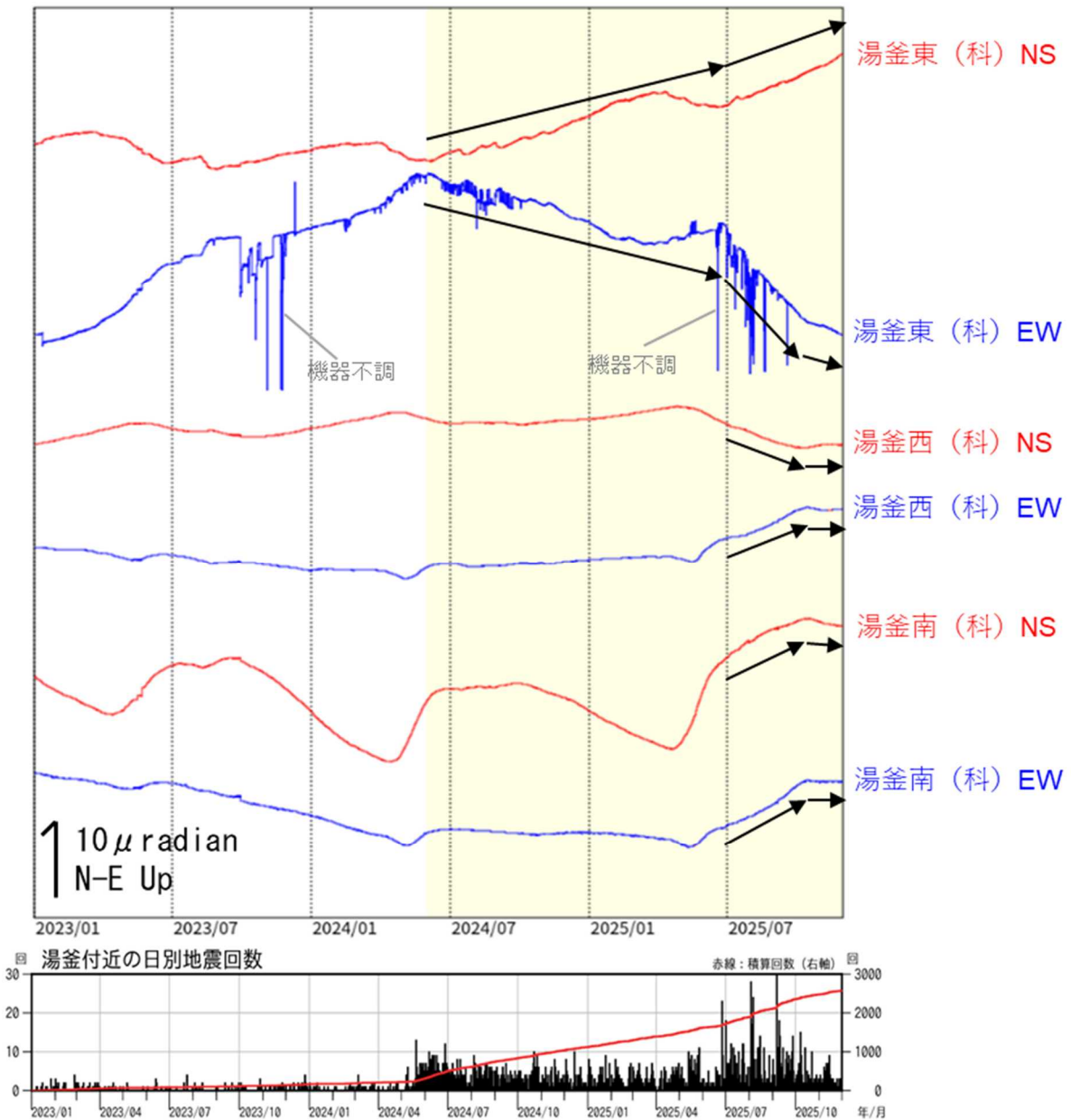
図6 草津白根山（白根山（湯釜付近）） 傾斜変動（2023年1月～2025年11月30日） データは時間平均値を使用しています。（科）：東京科学大学
