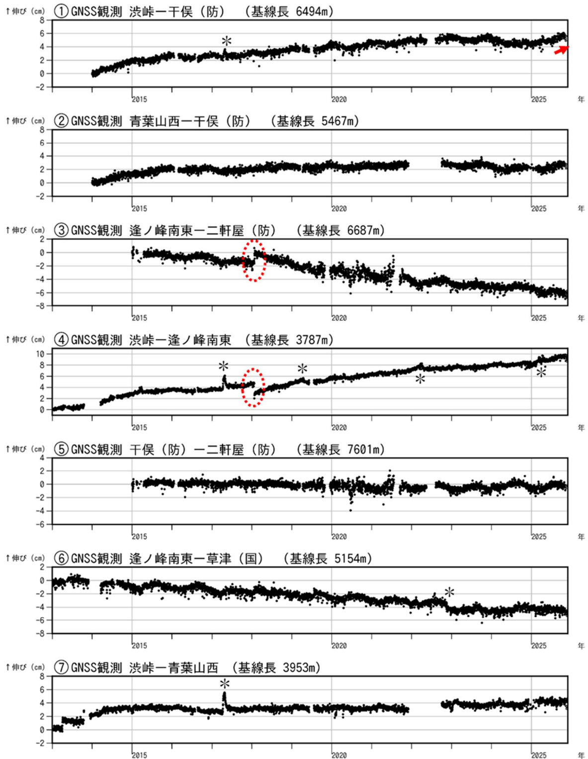
図 7-1 草津白根山 GNSS 連続観測結果（2013 年 1 月 1 日～2025 年 11 月 30 日）
