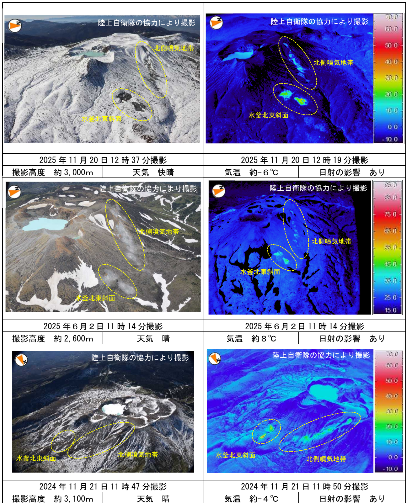
図 1-5 草津白根山（白根山（湯釜付近）） 湯釜火口北側噴気地帯及び水釜北東斜面の状況
