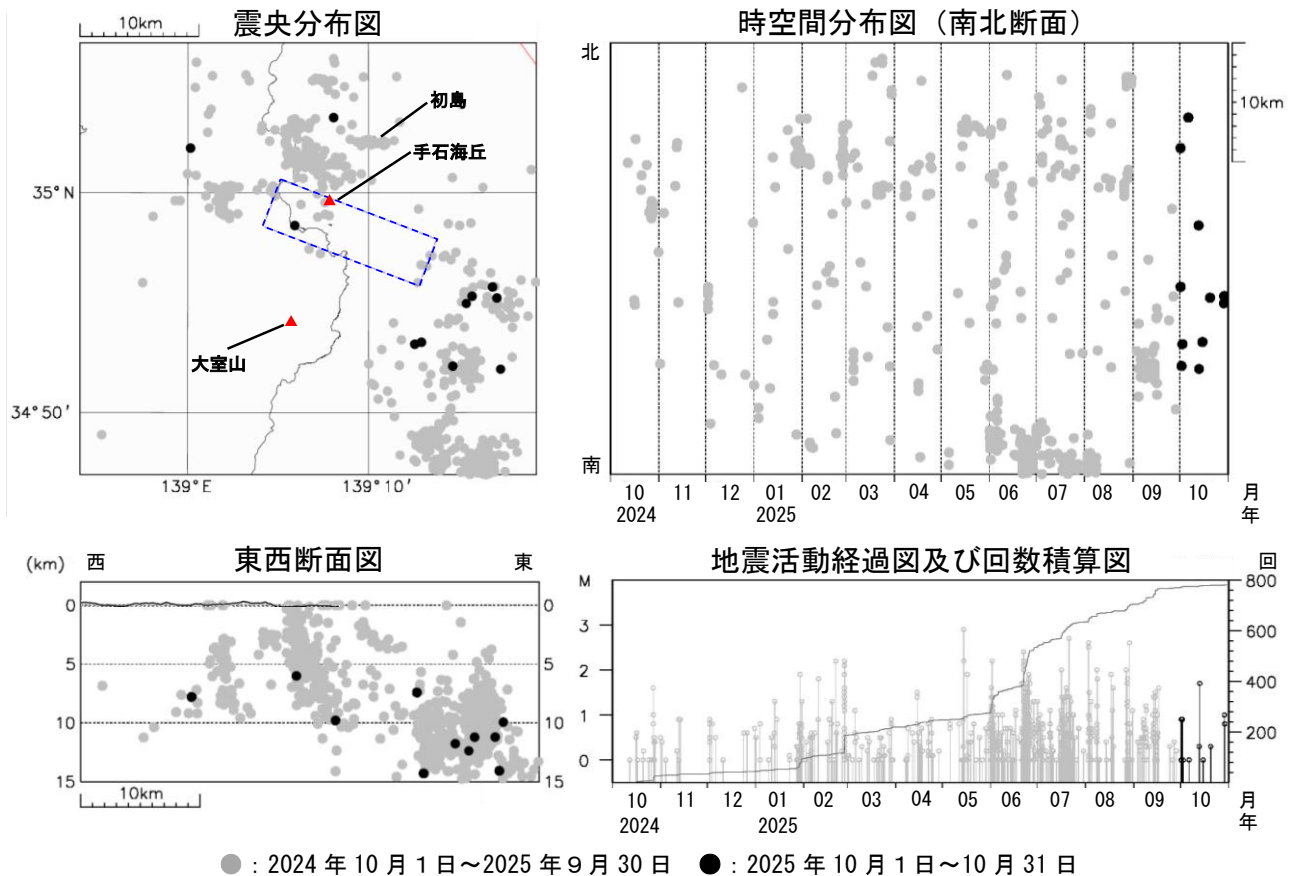
図2 伊豆東部火山群 広域地震観測網による震源分布図（2024 年 10 月 1 日～2025 年 10 月 31 日） □ の領域は群発地震活動の発生する可能性がある範囲（火口が出現する可能性のある範囲）を示しています。 https://www.data.jma.go.jp/vois/data/filing/level/PDF/level_316.pdf 広域地震観測網により震源決定したもので、深さは全て海面以下として決定しています。 M（マグニチュード）は地震の規模を表し、M0.0 以上を表示しています。 図中の震源要素は一部暫定値が含まれており、後日変更することがあります。 この図では、関係機関の地震波形を一元的に処理し、地震観測点の標高を考慮する等した手法で得られた震源を用いています。
