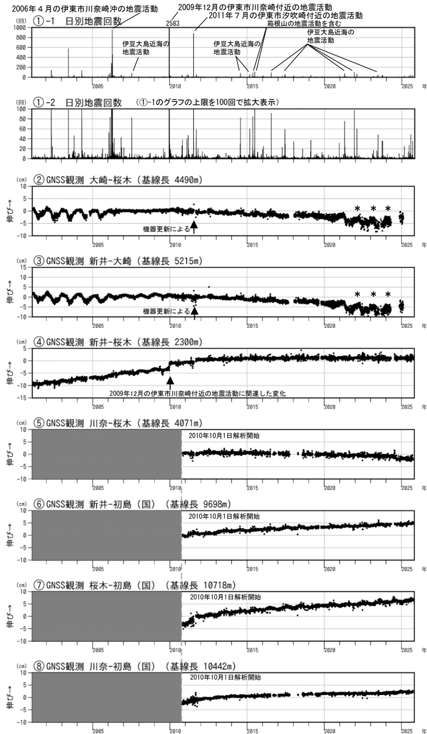
図3 伊豆東部火山群 火山活動経過図（2001年2月1日～2025年10月31日）
