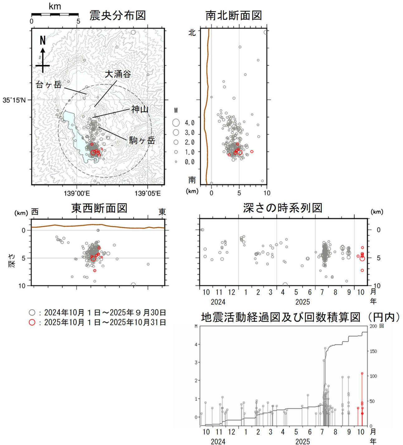
図4 箱根山 広域地震観測網による山体周辺の震源分布図（2024年10月1日～2025年10月31日）
