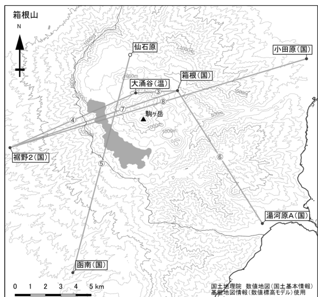
図3-2 箱根山 GNSS連続観測による 基線長変化及び観測点配置図 (2012年1月1日~2025年10月31日)
