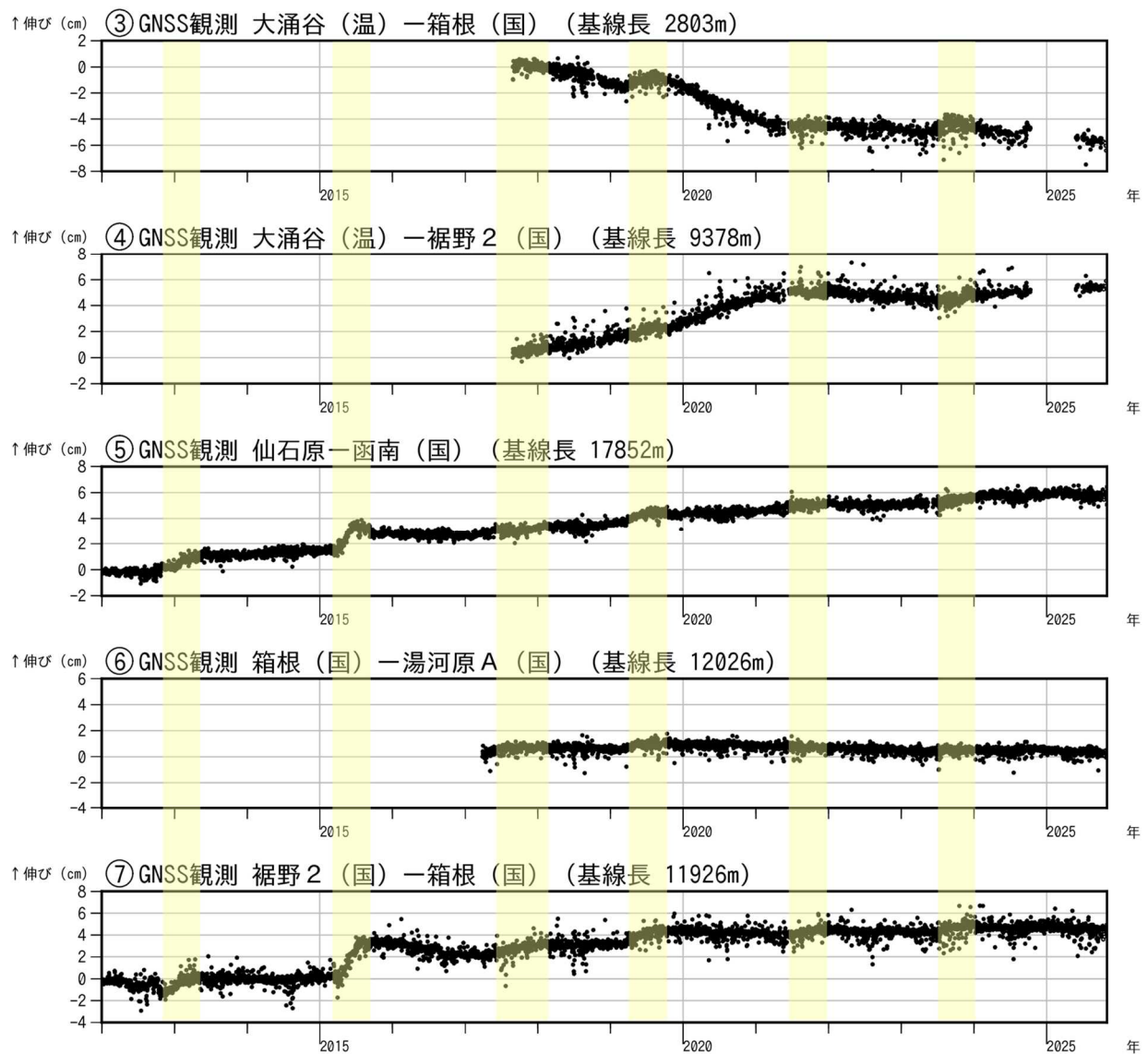
図3-2 箱根山 GNSS連続観測による 基線長変化及び観測点配置図 (2012年1月1日~2025年10月31日)
