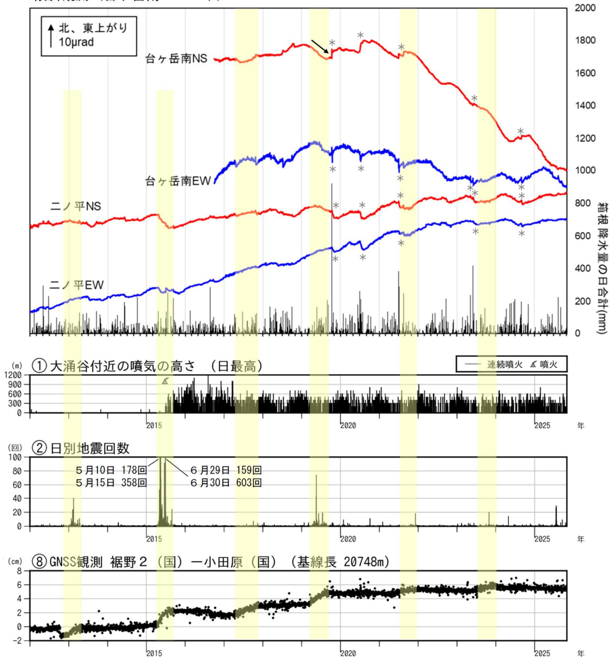
図3-1 箱根山 火山活動経過図（2012年1月1日～2025年10月31日）
