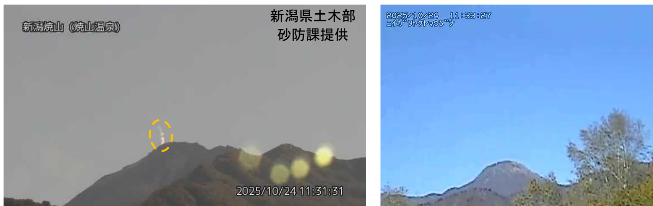
図 1 新潟焼山 山頂部の噴煙（橙色枠）の状況
