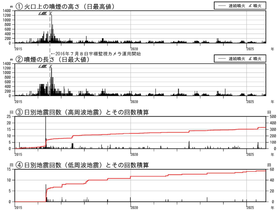
図7 新潟焼山 火山活動経過図（短期）（2015年1月1日～2025年10月31日）
