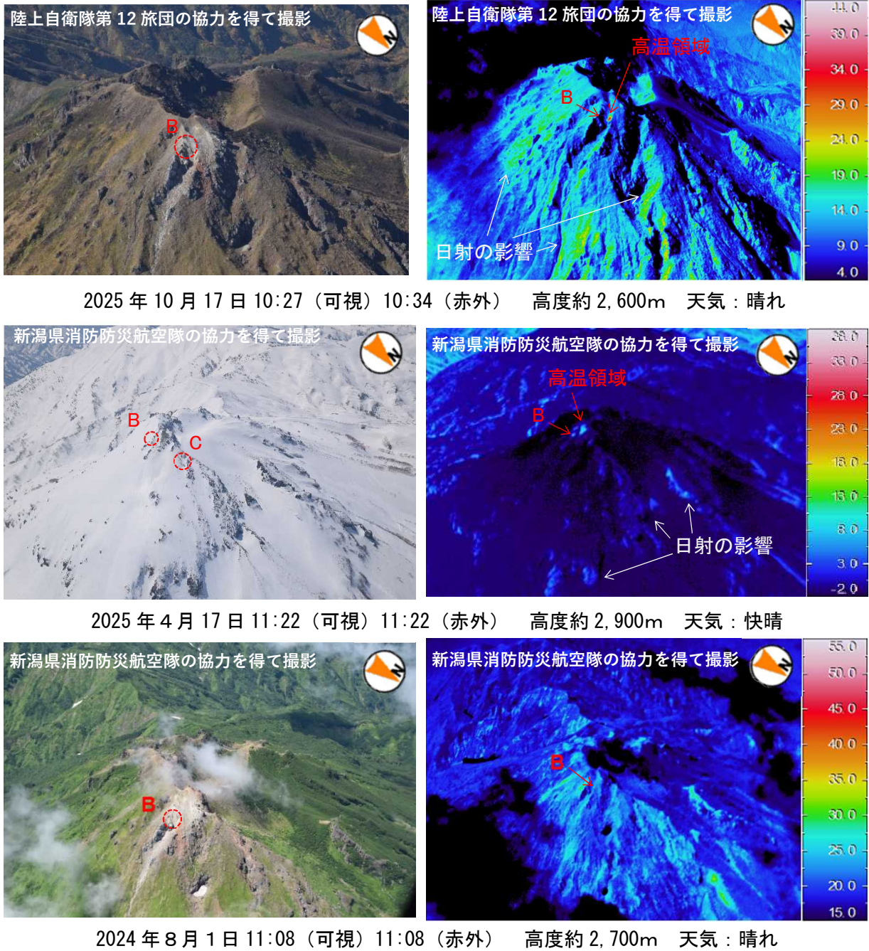
図2 新潟焼山 北東斜面の地熱域の推移
