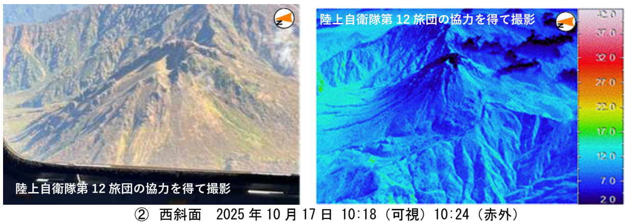
図4－1 新潟焼山 可視画像及び赤外熱映像装置による地表面温度分布 ・南及び西斜面では日射の影響を超えるような目立った高温領域は認められませんでした。
