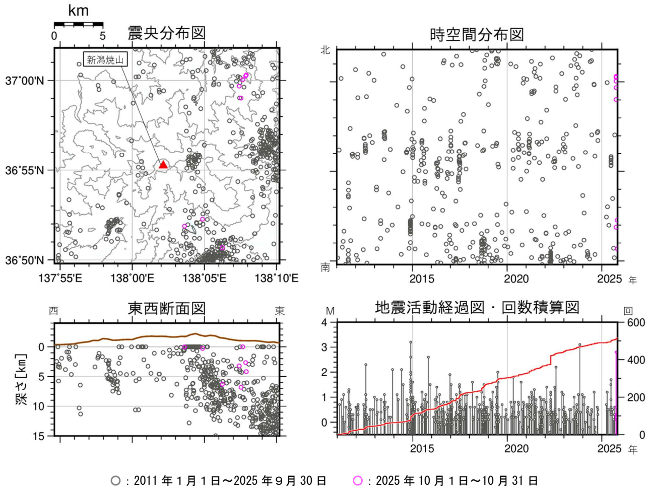
図8 新潟焼山 広域地震観測網による山体・周辺の地震活動（2011年1月1日～2025年10月31日） 広域地震観測網により震源決定したもので、深さは全て海面以下として決定しています。なお、2020年9月以降については、地震観測点の標高を考慮する等、震源決定の手法を変更しています。 図中の震源要素は一部暫定値が含まれており、後日変更することがあります。 ・新潟焼山周辺を震源とする地震活動は低調に経過しました。
