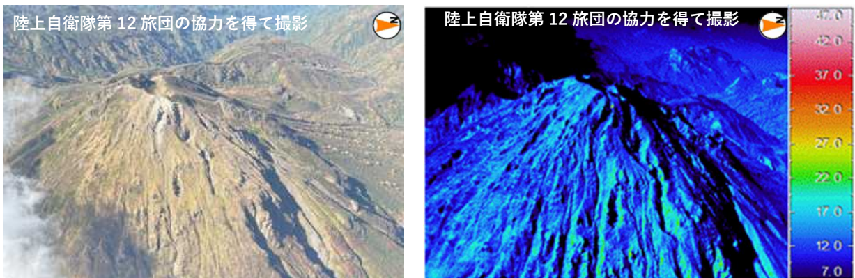
図4－2 新潟焼山 可視画像及び赤外熱映像装置による地表面温度分布
