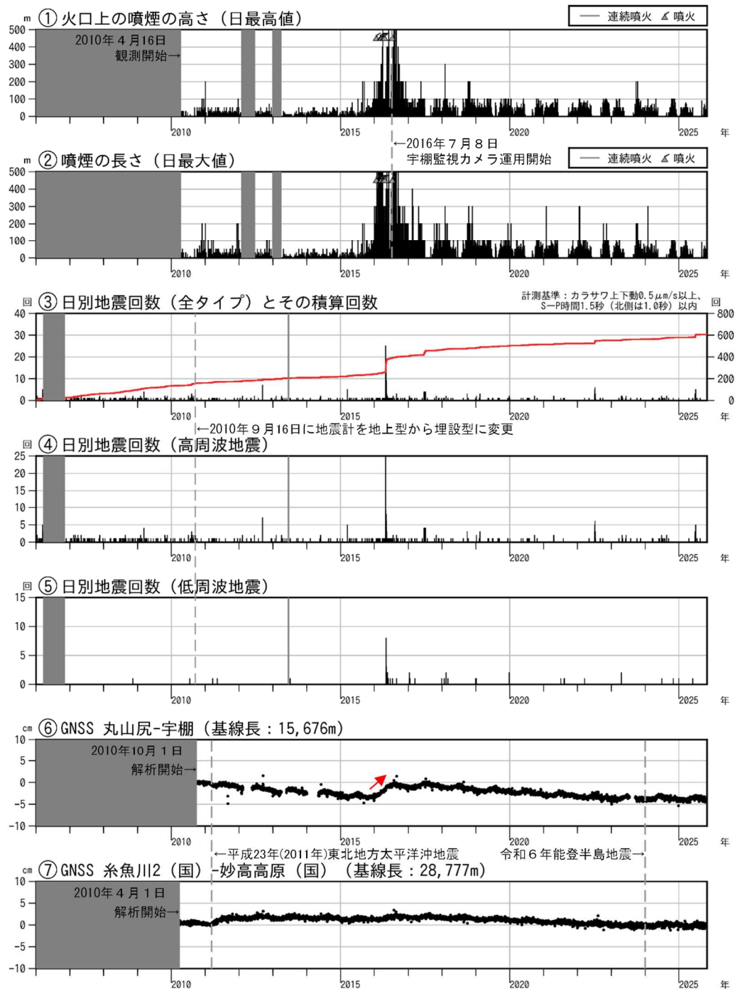
図6 新潟焼山 火山活動経過図（2006年1月1日～2025年10月31日）
