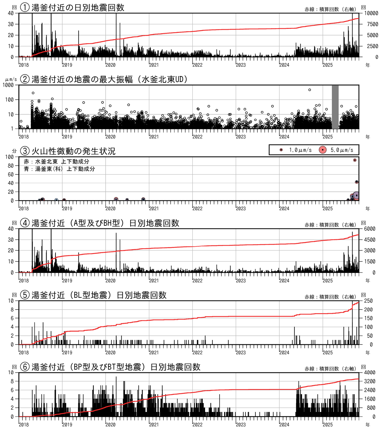
図6 草津白根山（白根山（湯釜付近）） 湯釜付近の地震活動の状況
