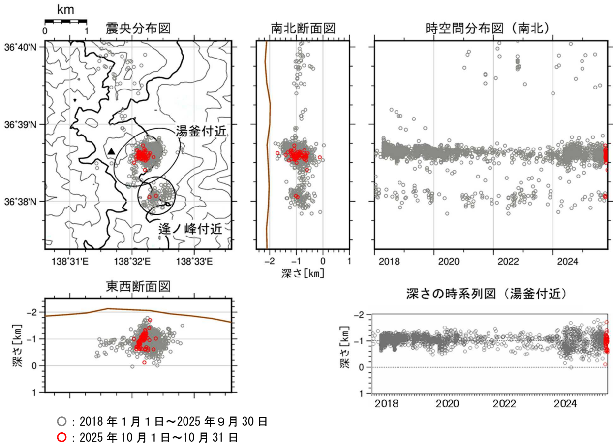
図5 草津白根山 震源分布図（2018 年 1 月 1 日～2025 年 10 月 31 日）
