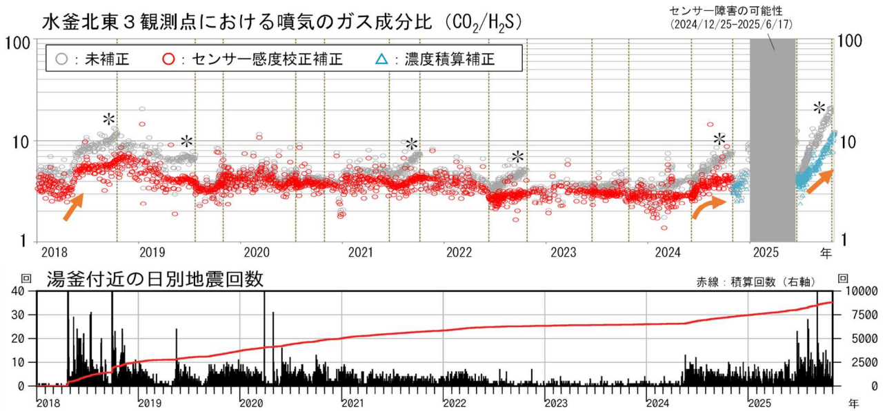
図2 草津白根山（白根山（湯釜付近）） 火山ガス観測結果（2018年1月～2025年10月31日）
