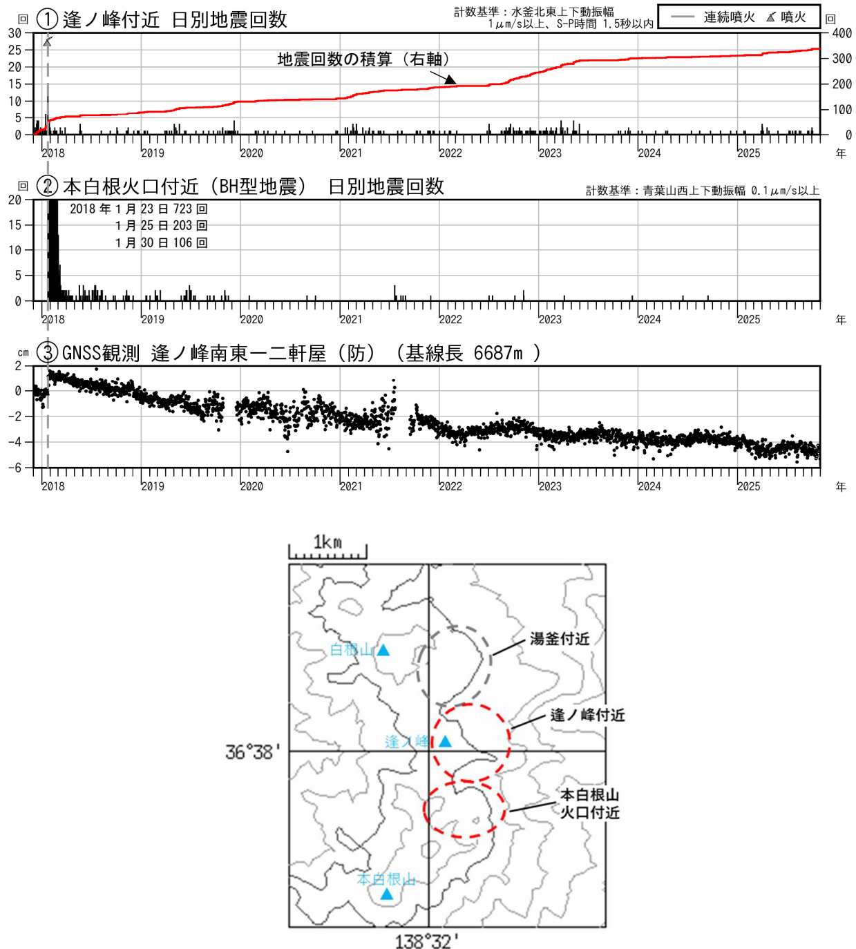
図 17 草津白根山（本白根山） 火山活動経過図（2017年12月1日～2025年10月31日）
