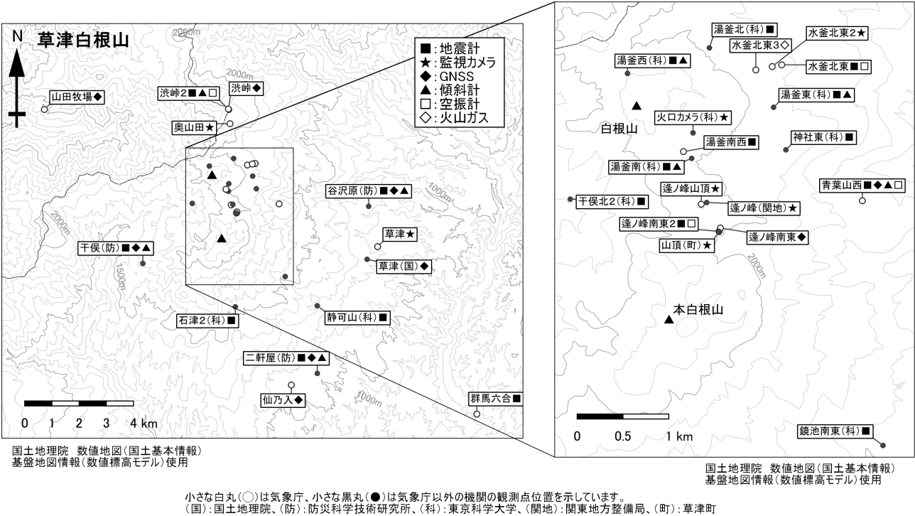
図 19 草津白根山 観測点配置図
