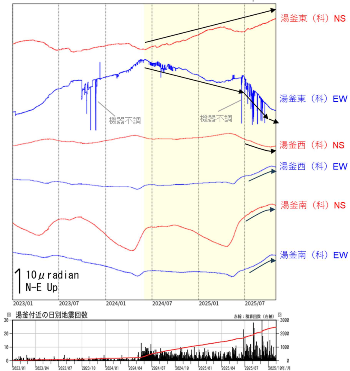
図7 草津白根山（白根山（湯釜付近）） 傾斜変動（2023年1月～2025年10月31日） データは時間平均値を使用しています。（科）：東京科学大学
