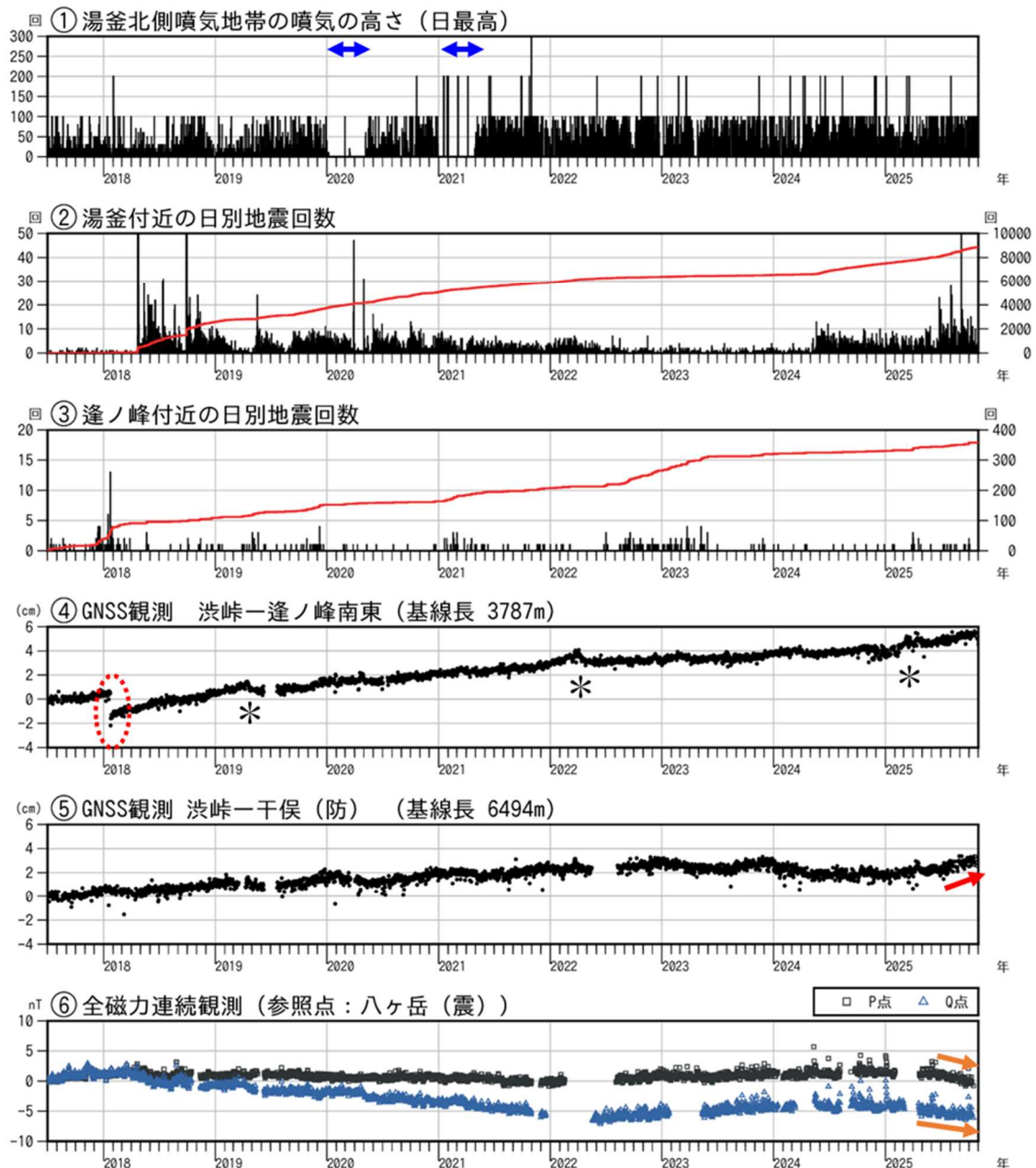
図 11 草津白根山（白根山（湯釜付近）） 火山活動経過図（2017 年 7 月 1 日～2025 年 10 月 31 日）
