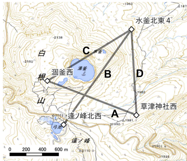
図9-1 草津白根山 緊急設置 GNSS 観測点配置図
