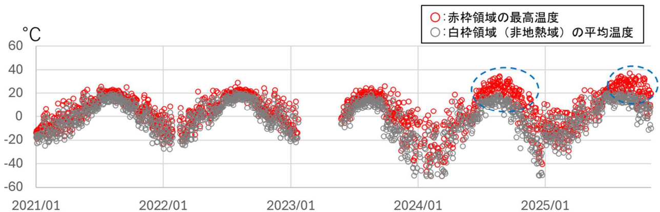
図1-4 草津白根山（白根山（湯釜付近）） 水釜北東の地熱域の状況 (2021年1月1日～2025年10月31日)
