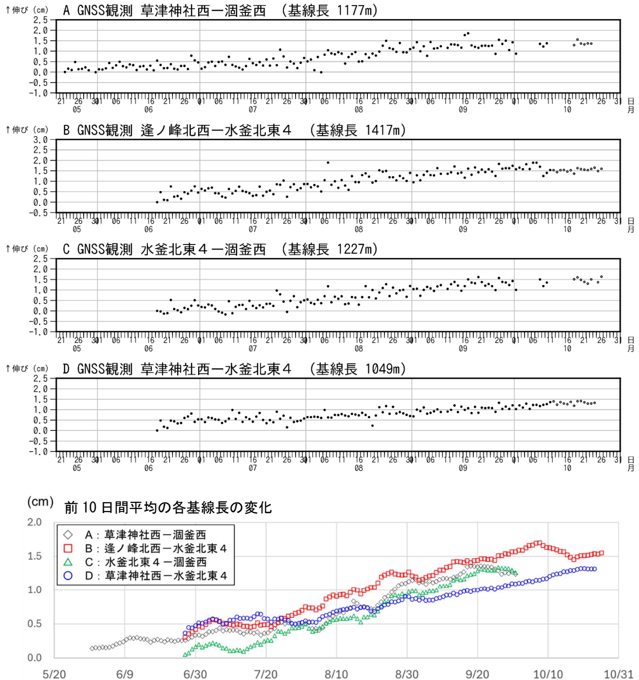
図 8 草津白根山 湯釜近傍での臨時の GNSS 連続観測結果（2025 年 5 月 20 日～2025 年 10 月 31 日） 図中の GNSS 基線番号 A～D は図 9－1 に対応しています。
