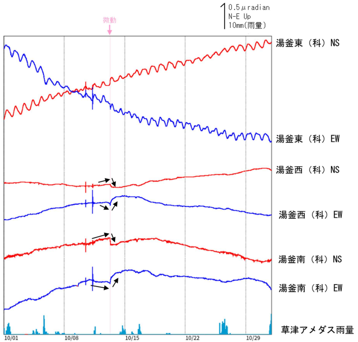
図4 草津白根山（白根山（湯釜付近）） 火山性微動の発生前後に観測された傾斜変動 データは10月1日から31日までの分値を使用しています。（科）：東京科学大学
