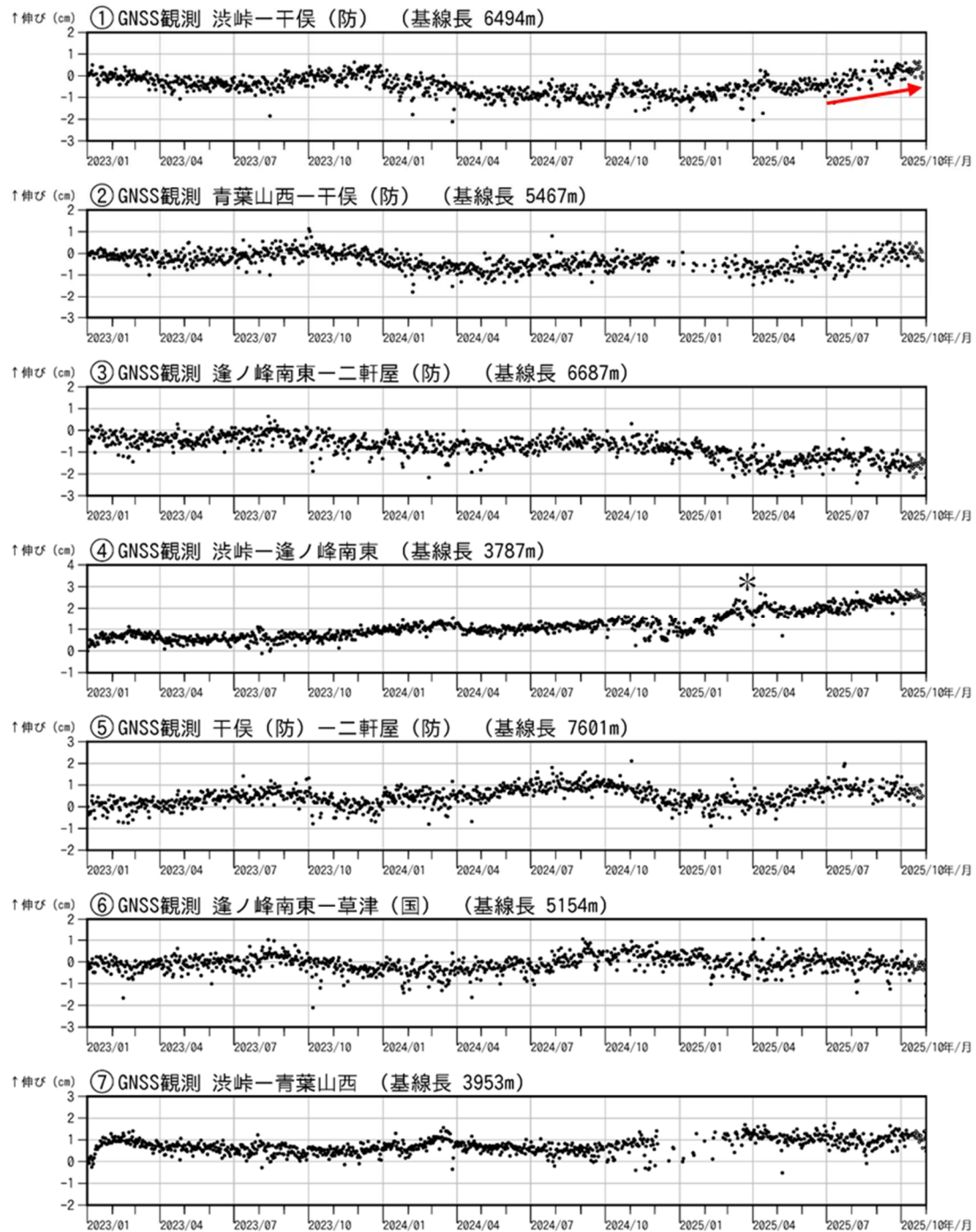
図 10-2 草津白根山 GNSS 連続観測結果（2023 年 1 月 1 日～2025 年 10 月 31 日）
