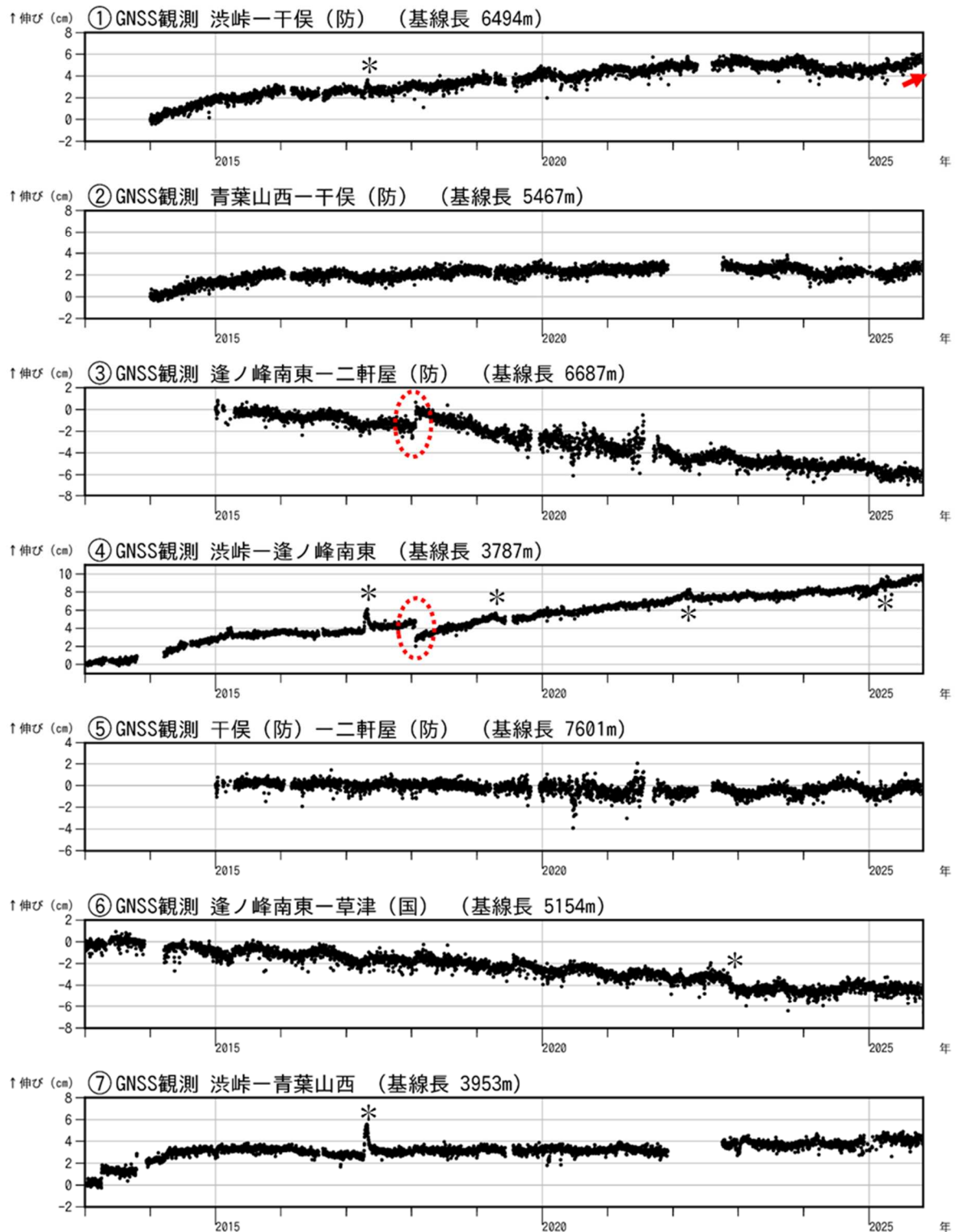
図 10-1 草津白根山 GNSS 連続観測結果（2013 年 1 月 1 日～2025 年 10 月 31 日）
