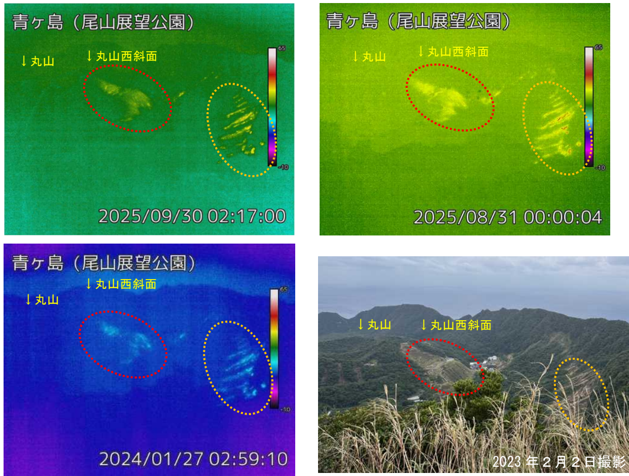
図2 青ヶ島 カルデラ内の地表面温度の状況（左上、右上、左下：尾山展望公園監視カメラによる、右下：2023年2月2日に撮影した同場所からの写真） ・地熱活動（赤点線及び黄色点線で示した範囲）に変化は認められません。
