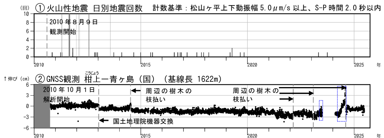
図3 青ヶ島 火山活動経過図（2010年8月9日～2025年9月30日） ① グラフの灰色部分は機器障害による欠測を示す。 ② （国）：国土地理院、図4のGNSS基線②に対応。グラフの空白部分は柑上の障害による欠測を示す。 ・青破線で囲んだ変化は柑上観測点周囲の樹木による影響と考えています。
