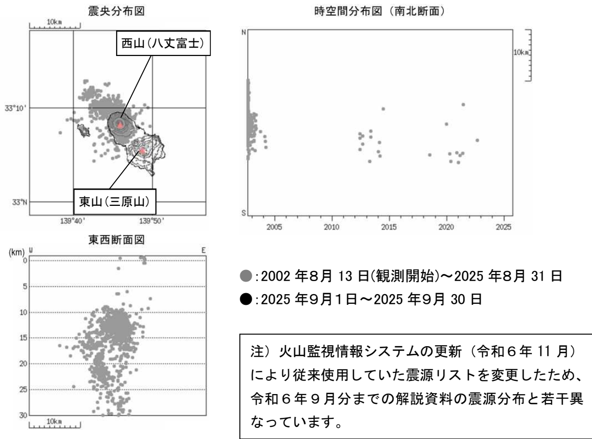
図3 八丈島 震源分布図 (2002年8月13日~2025年9月30日)
