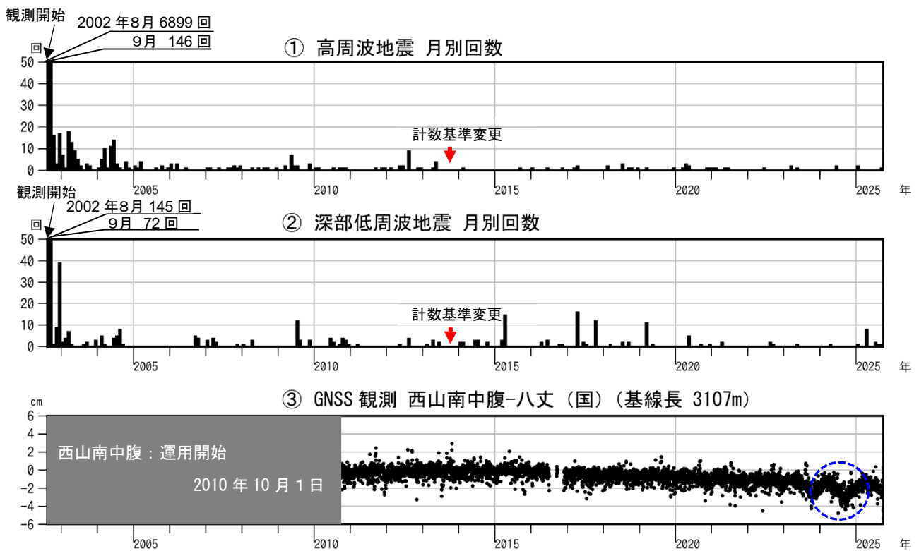
図 2 八丈島 火山活動経過図（2002 年 8 月 13 日～2025 年 9 月 30 日）
