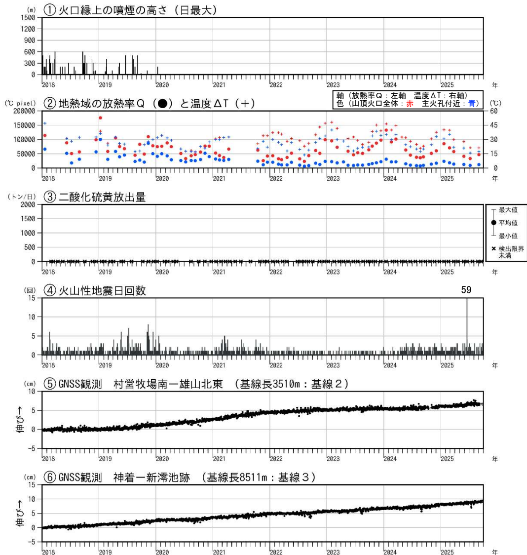
図5 三宅島 火山活動経過図（2018年1月1日～2025年9月30日）
