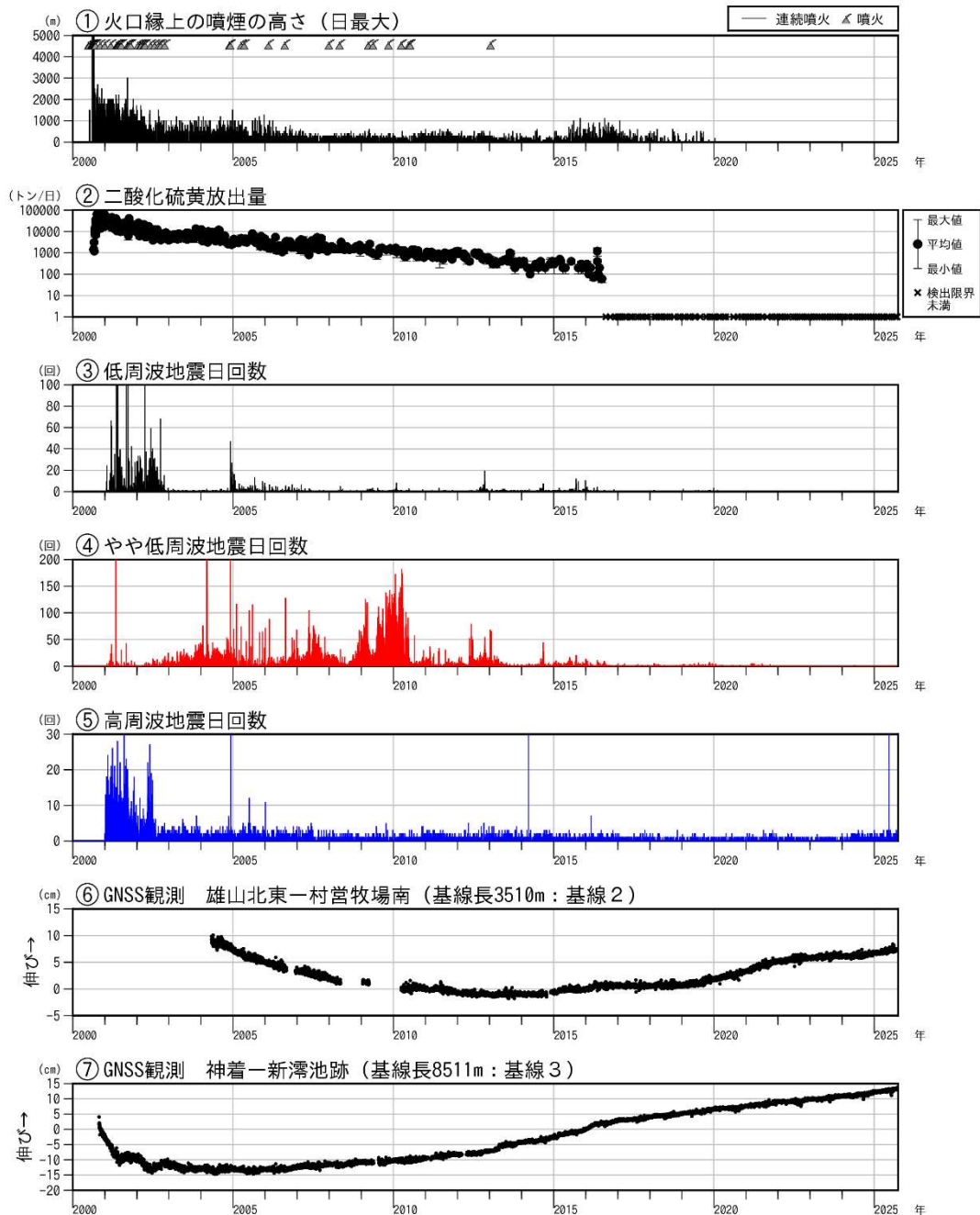
図6 三宅島 長期の火山活動経過図（2000年1月1日～2025年9月30日）
