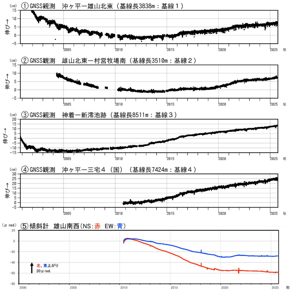
図7 三宅島 GNSS 連続観測及び傾斜計観測結果（2000年10月26日～2025年9月30日）
