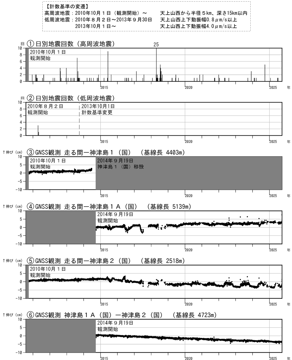
図2 神津島 火山活動経過図(2010年8月2日～2025年9月30日)
