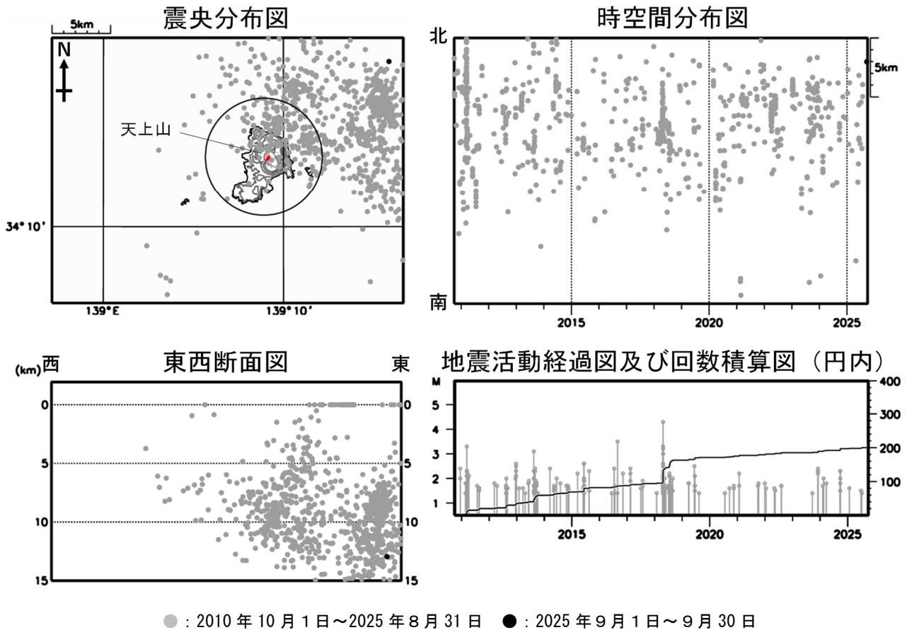
図 3 神津島 広域地震観測網による山体・周辺の地震活動（2010年10月1日～2025年9月30日） 広域地震観測網により震源決定したもので、深さは全て海面以下として決定しています。なお、2020年9月以降については、地震観測点の標高を考慮する等、震源決定の手法を変更しています。 M（マグニチュード）は地震の規模を表し、M1.4以上の地震を示しています。 図中の震源要素は一部暫定値が含まれており、後日変更することがあります。 計数対象（天上山西から半径約5km、深さ約15km以内）以外の地震が含まれるため、図2－①の日別地震回数（高周波地震）とは異なります。 震央分布図中の円は火山性地震の回数の計数対象（天上山西から半径5km、深さ15km以内）の範囲を示しています。 ・地震活動は低調に経過しました。
