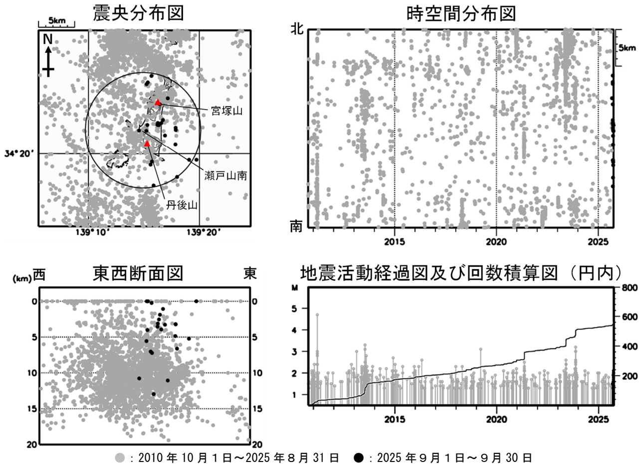
図3 新島 広域地震観測網による山体・周辺の地震活動（2010年10月1日～2025年9月30日） 広域地震観測網により震源決定したもので、深さは全て海面以下として決定しています。なお、2020年9月以降については、地震観測点の標高を考慮する等、震源決定の手法を変更しています。 M（マグニチュード）は地震の規模を表し、M1.3以上の地震を示しています。 図中の震源要素は一部暫定値が含まれており、後日変更することがあります。 計数対象（瀬戸山南から半径約8km、深さ約20km以内）以外の地震が含まれるため、図2-①の日別地震回数（高周波地震）とは異なります。 震央分布図中の円は火山性地震の回数の計数対象（瀬戸山南から半径8km、深さ20km以内）の範囲を示しています。 ・地震活動は低調に経過しました。
