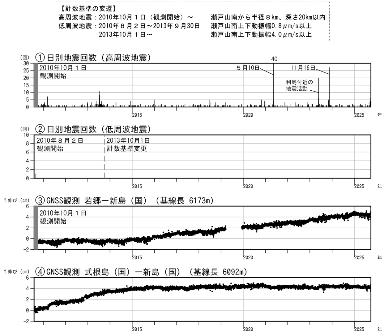
図2 新島 火山活動経過図(2010年8月2日～2025年9月30日)
