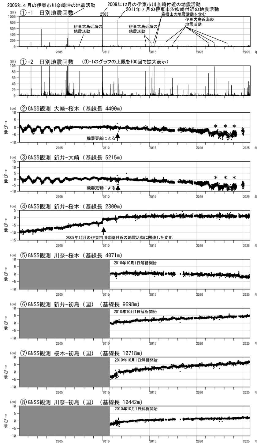
図3 伊豆東部火山群 火山活動経過図（2001年2月1日～2025年9月30日）
