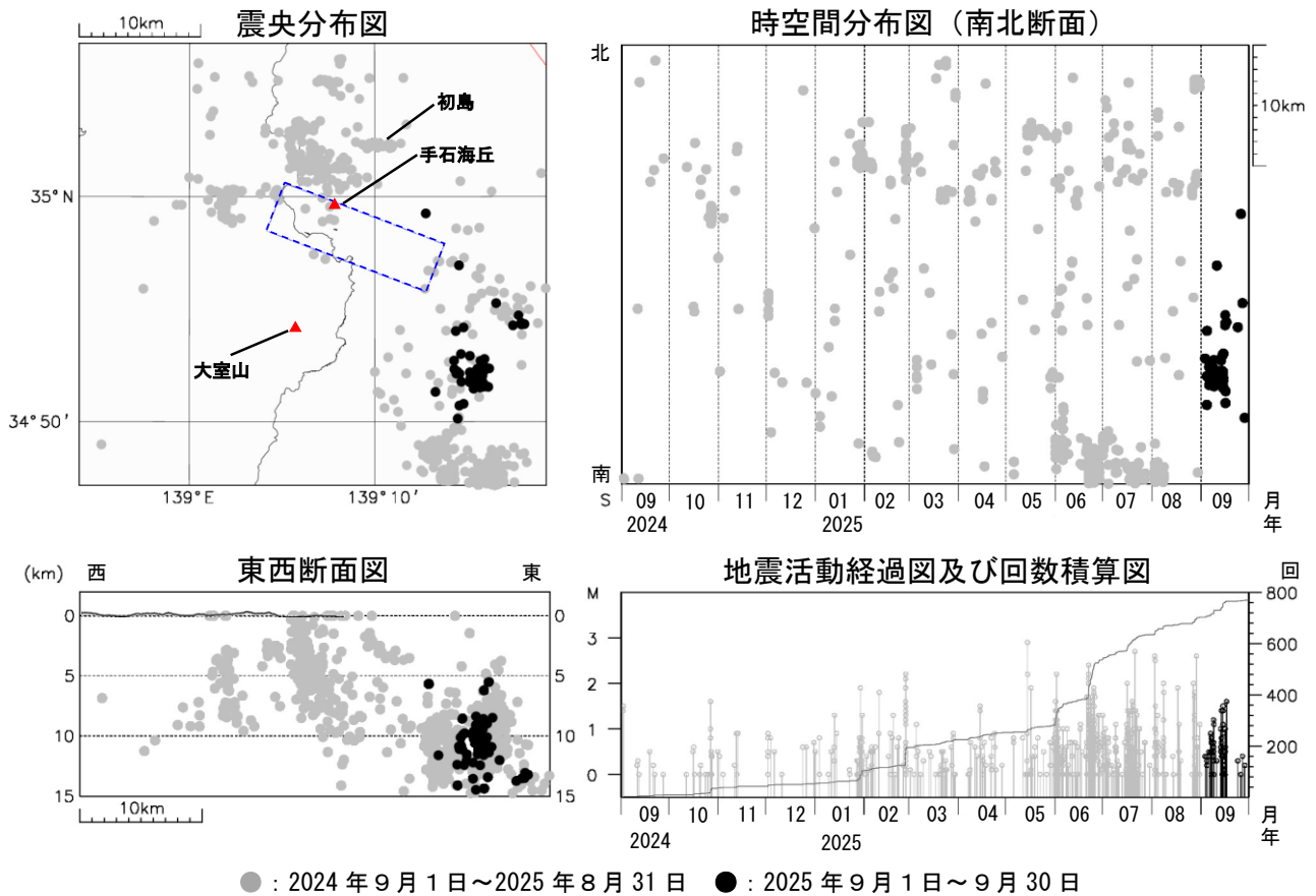
図2 伊豆東部火山群 広域地震観測網による震源分布図（2024 年 9 月 1 日～2025 年 9 月 30 日） □ の領域は群発地震活動の発生する可能性がある範囲（火口が出現する可能性のある範囲）を示しています。 https://www.data.jma.go.jp/vois/data/filing/level/PDF/level_316.pdf 広域地震観測網により震源決定したもので、深さは全て海面以下として決定しています。 M（マグニチュード）は地震の規模を表し、M0.0 以上を表示しています。 図中の震源要素は一部暫定値が含まれており、後日変更することがあります。 この図では、関係機関の地震波形を一元的に処理し、地震観測点の標高を考慮する等した手法で得られた震源を用いています。
