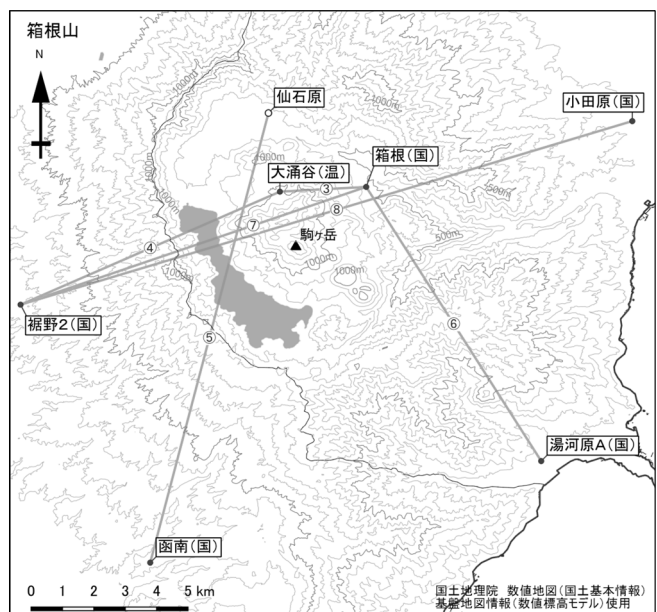
図3-2 箱根山 GNSS連続観測による 基線長変化及び観測点配置図 (2012年1月1日～2025年9月30日)
