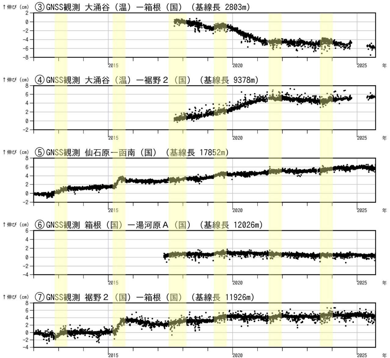
図3-2 箱根山 GNSS連続観測による 基線長変化及び観測点配置図 (2012年1月1日～2025年9月30日)
