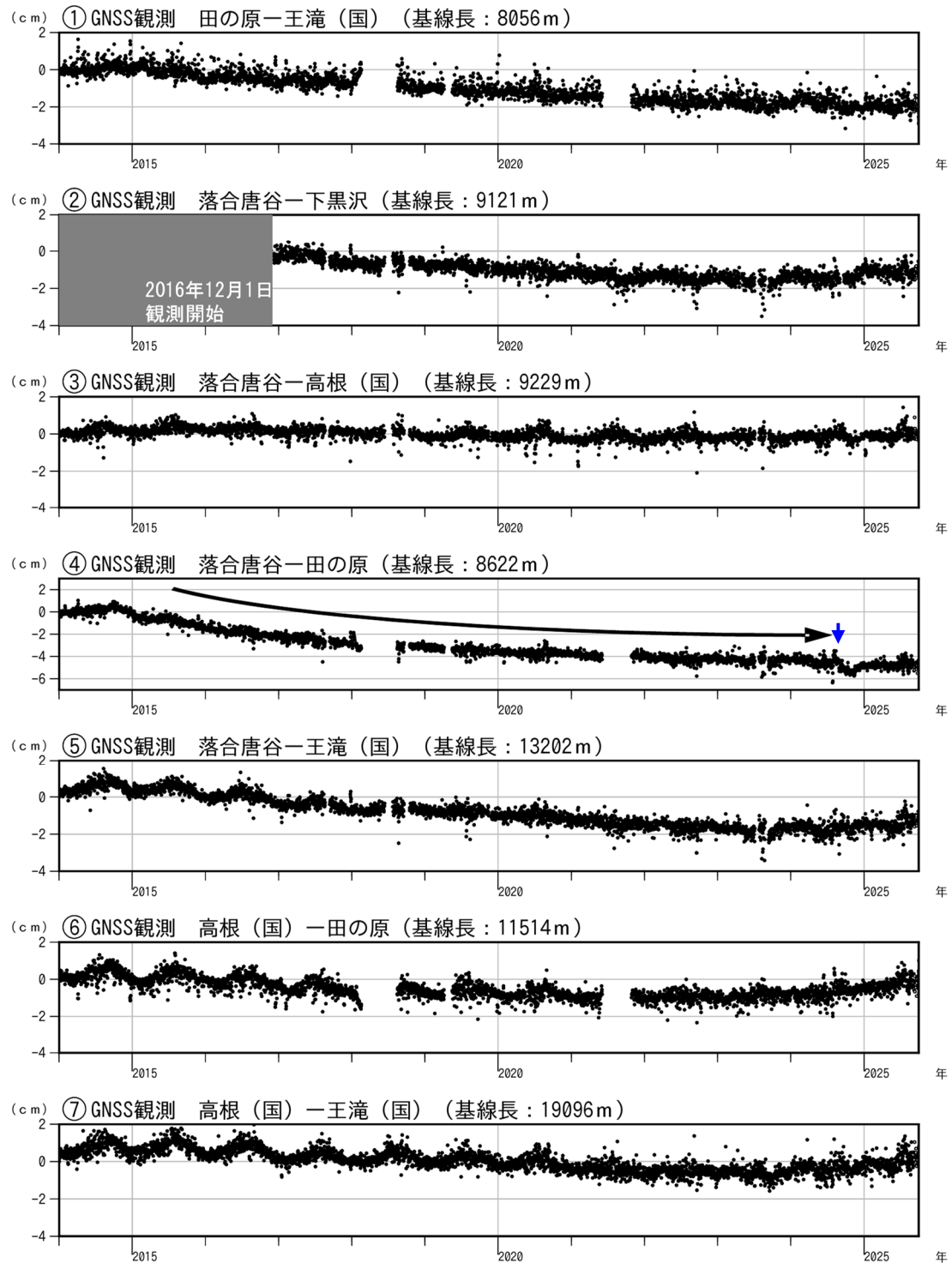
図5 御嶽山 GNSS 連続観測結果（2014 年 1 月 1 日～2025 年 9 月 30 日）
