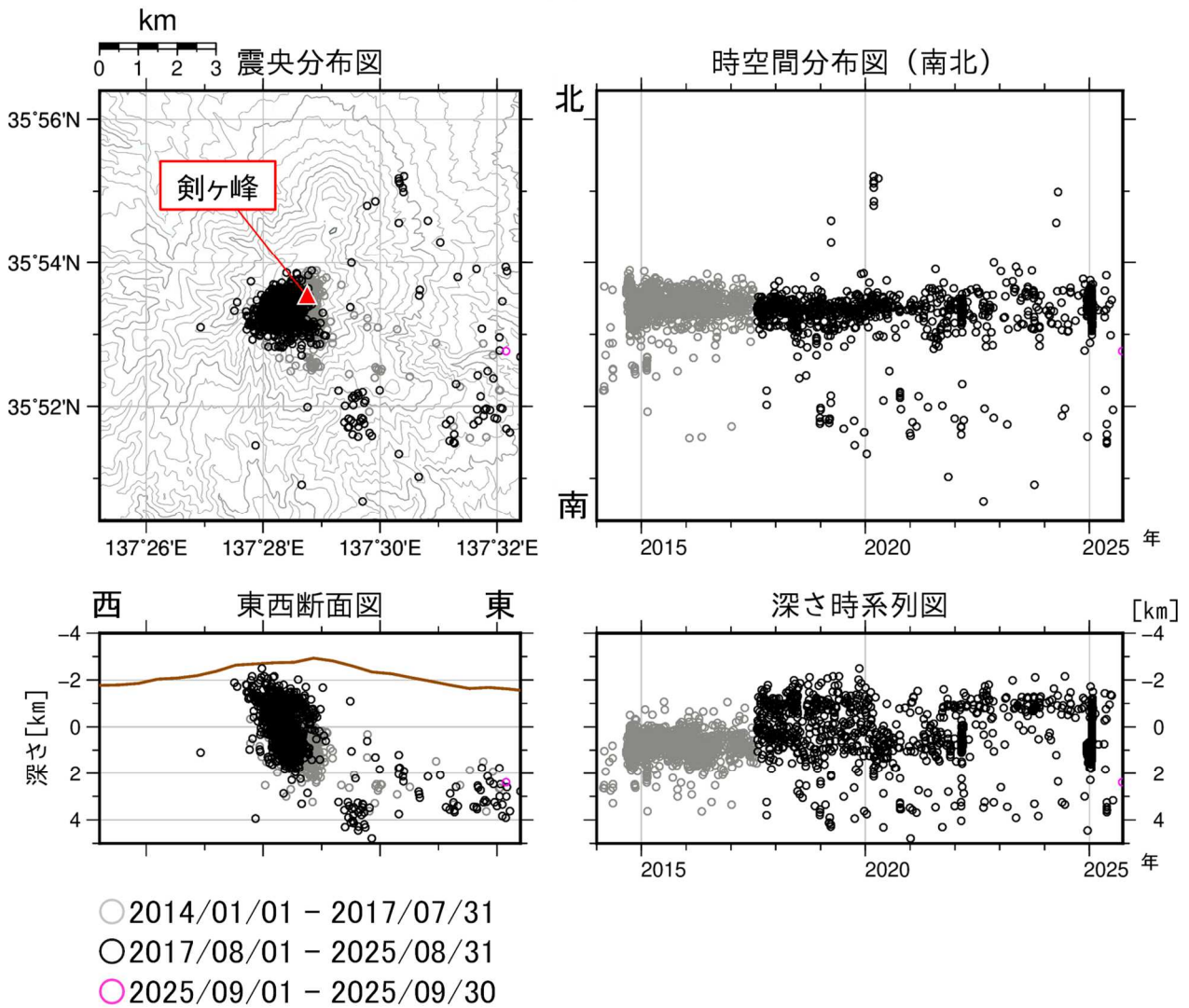
図4 御嶽山 震源分布図（2014年1月1日～2025年9月30日）
