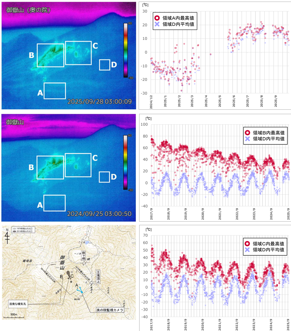
図3 御嶽山 奥の院赤外熱映像カメラによる地獄谷火口における最高温度の推移 (2017年9月13日～2025年9月30日)
