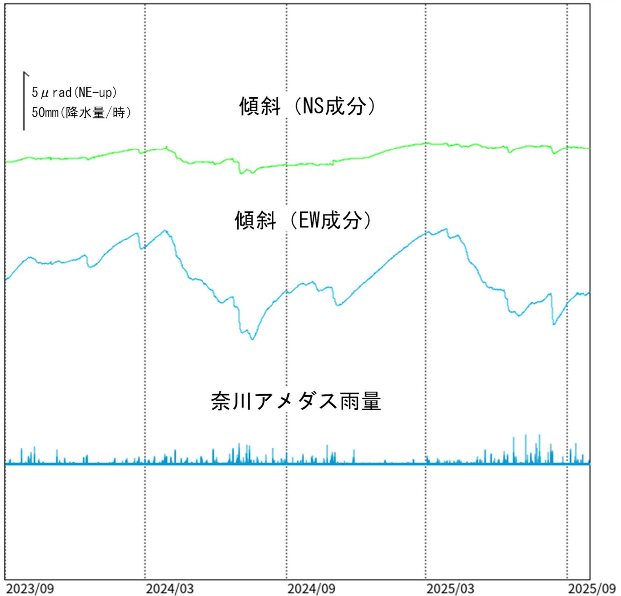
図4 乗鞍岳 三本滝観測点における傾斜データ（2023年9月1日～2025年9月30日） ・傾斜計による観測では、火山活動によるとみられる変動は認められません。
