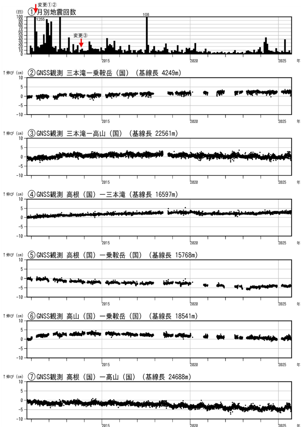
図2 乗鞍岳 火山活動経過図（2010年10月1日～2025年9月30日）
