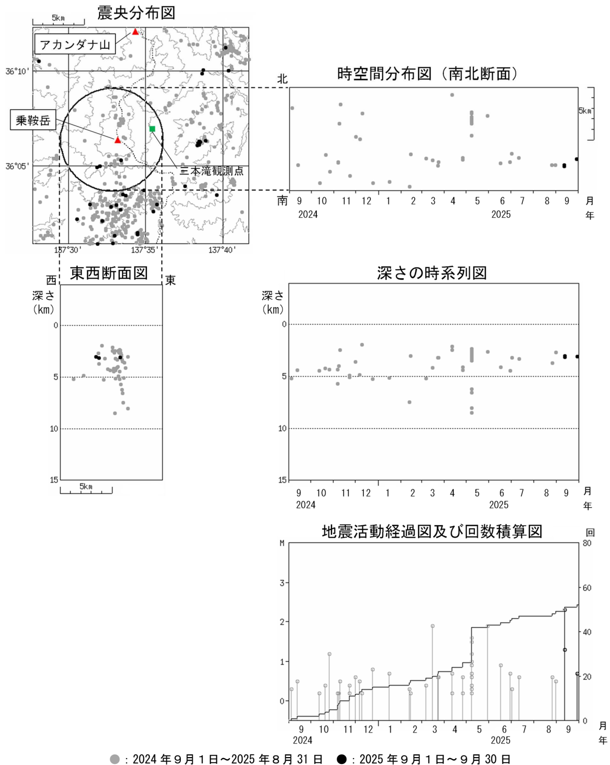
図3 乗鞍岳 広域地震観測網による山体・周辺の地震活動(2024年9月1日～2025年9月30日)
