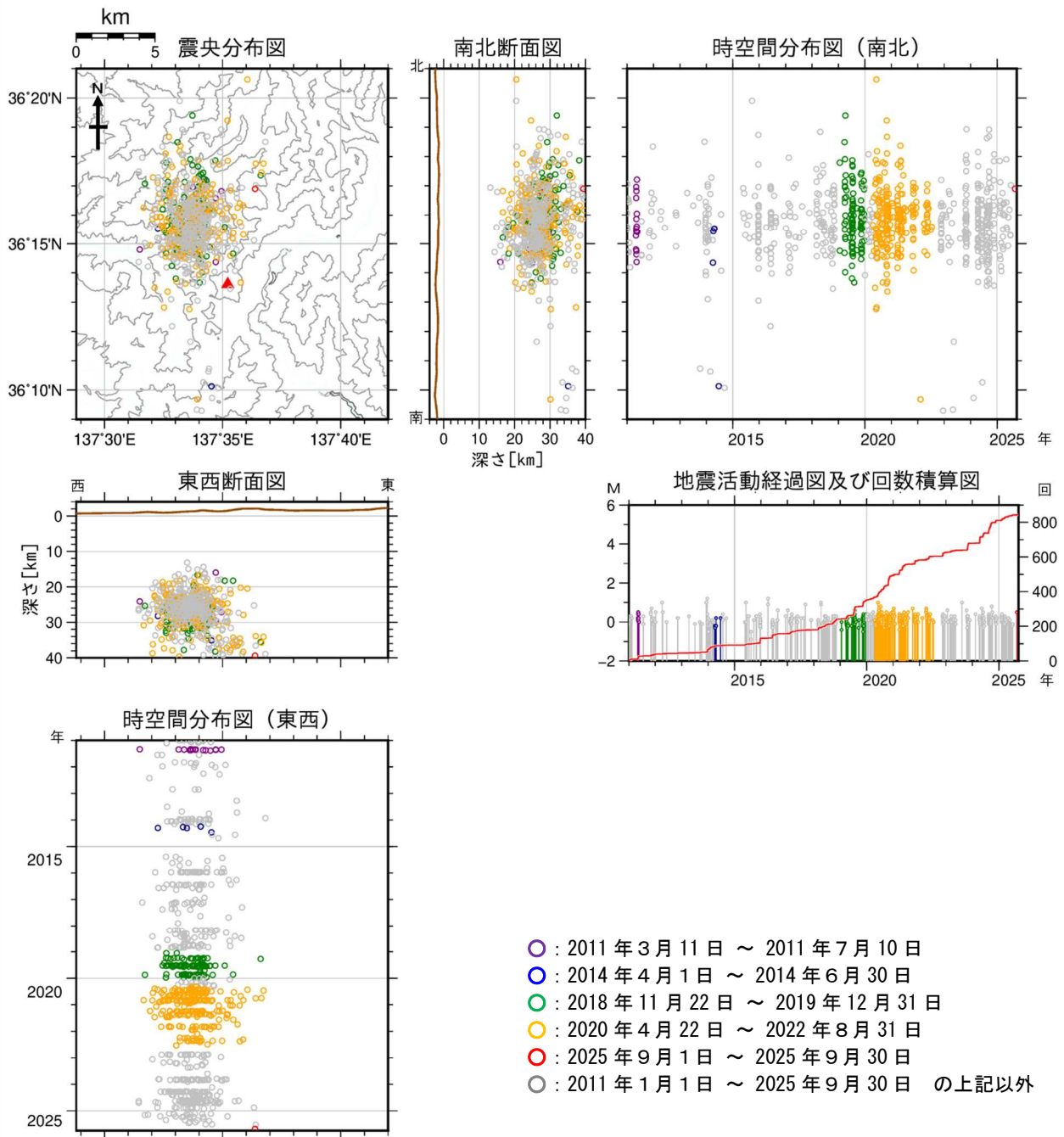
図10 焼岳 広域地震観測網による深部低周波地震の震源分布図（2011年1月1日～2025年9月30日）
