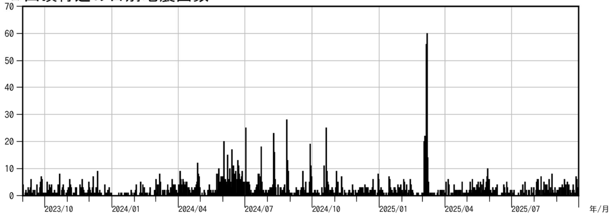
図8 焼岳 南峰南東観測点における傾斜データ（2023年9月1日～2025年9月30日）
