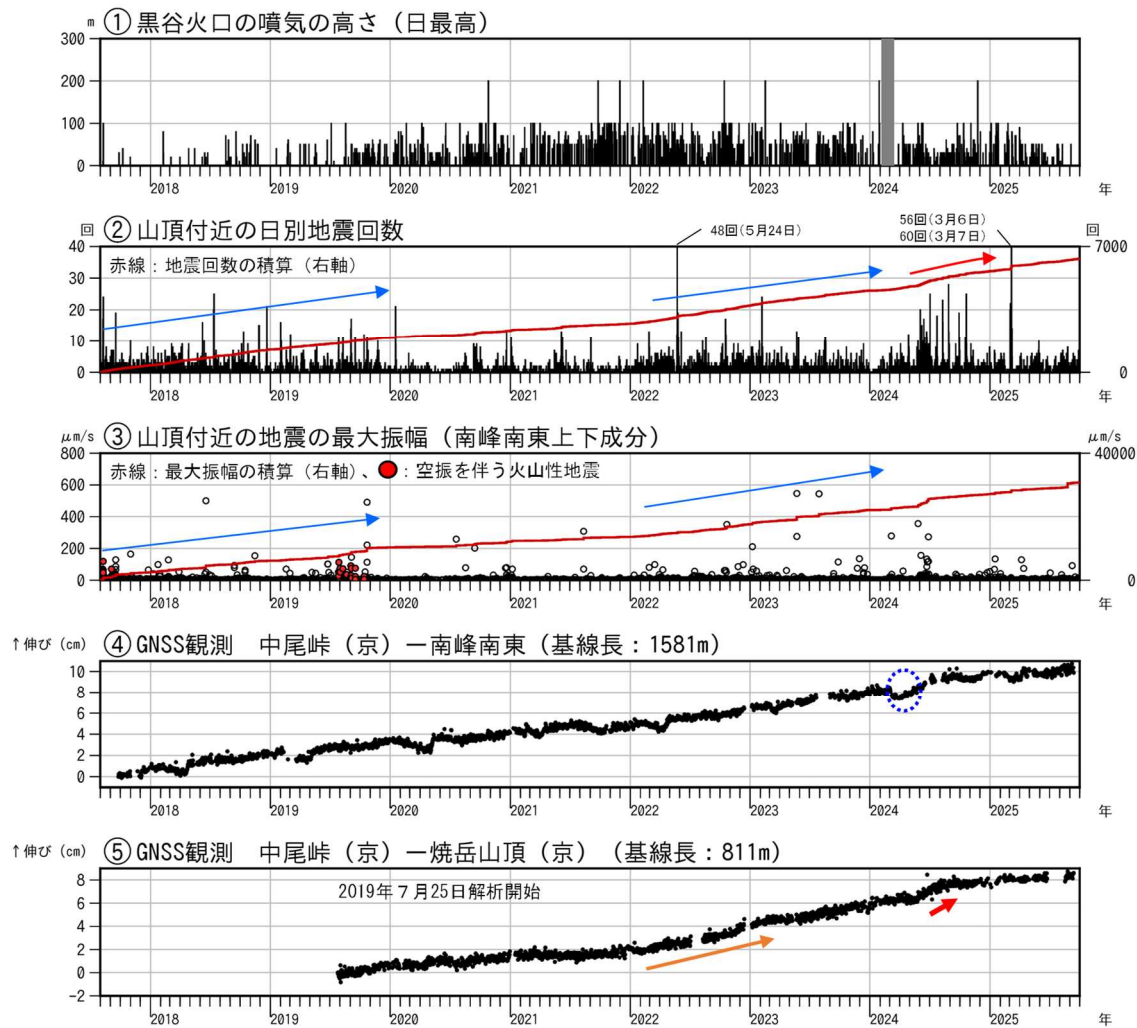
図1 焼岳 火山活動経過図（2017年8月1日～2025年9月30日）
