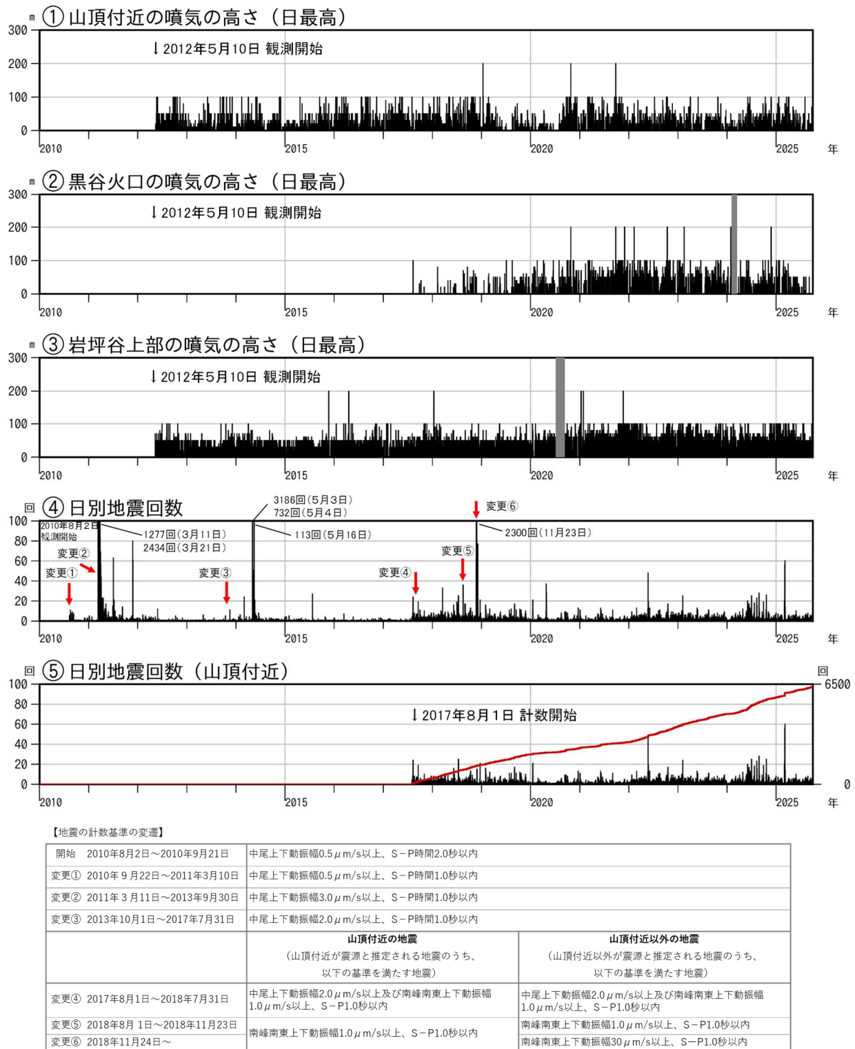
図5 焼岳 噴気の高さと地震回数の推移(2010年8月2日～2025年9月30日)
