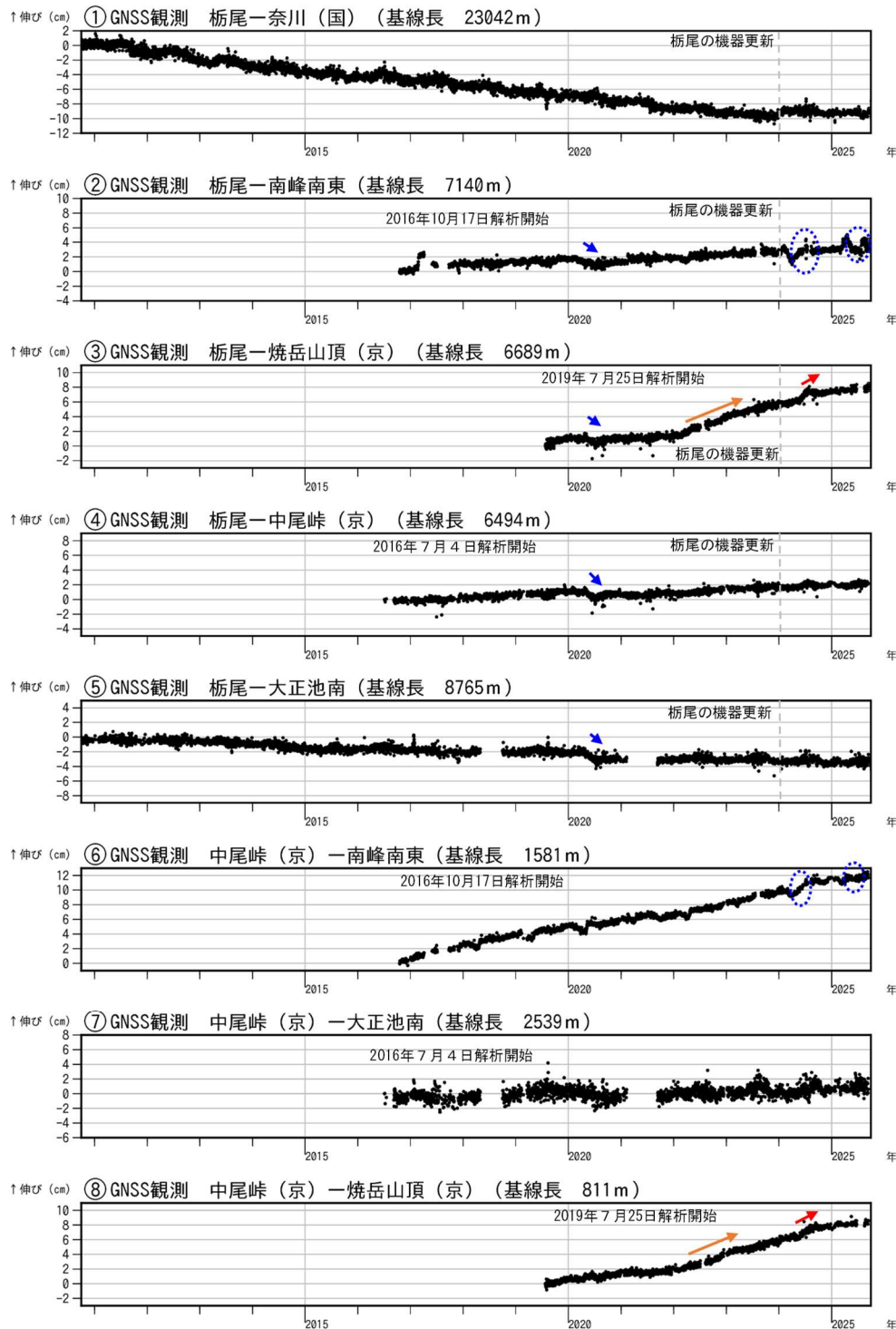
図6 焼岳 GNSS 連続観測による基線長変化（2010年10月1日～2025年9月30日）
