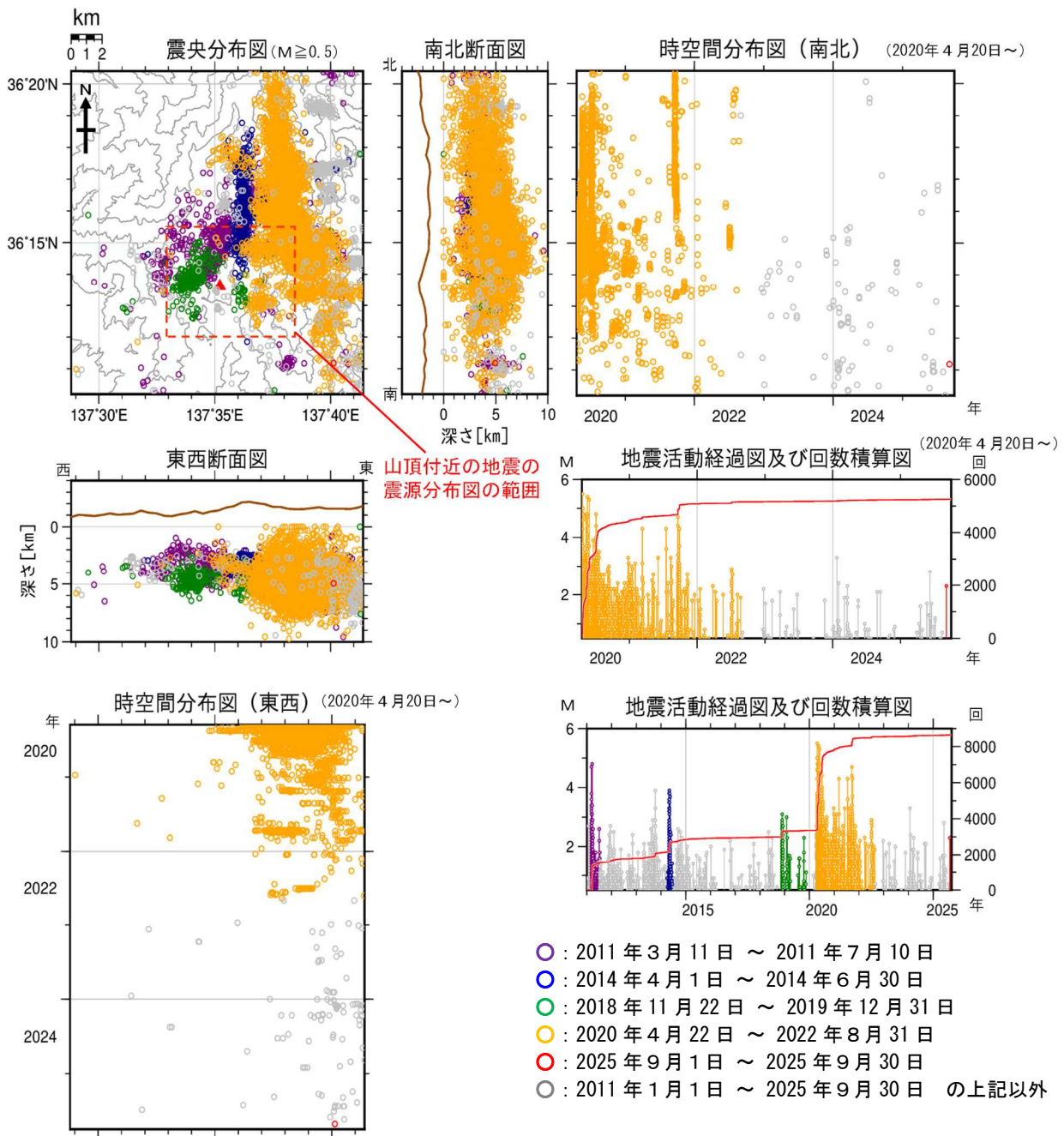
図9 焼岳 広域地震観測網による山体及び周辺の地震活動(2011年1月1日~2025年9月30日)
