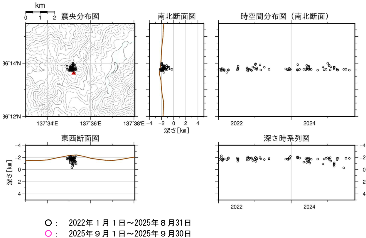
図2 焼岳 山頂付近の地震の震源分布図（2022年1月1日～2025年9月30日）
