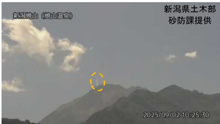
図 1 新潟焼山 山頂部の噴煙（橙色枠）の状況 （左：焼山温泉監視カメラ（9月2日）、右：宇棚監視カメラ（9月2日）による）
