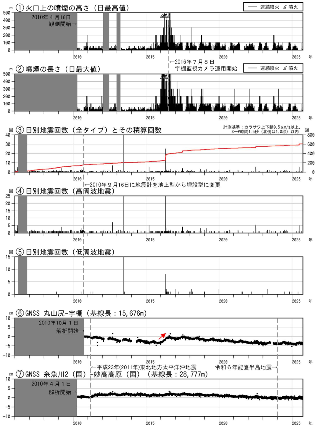
図2 新潟焼山 火山活動経過図（2006年1月1日～2025年9月30日）
