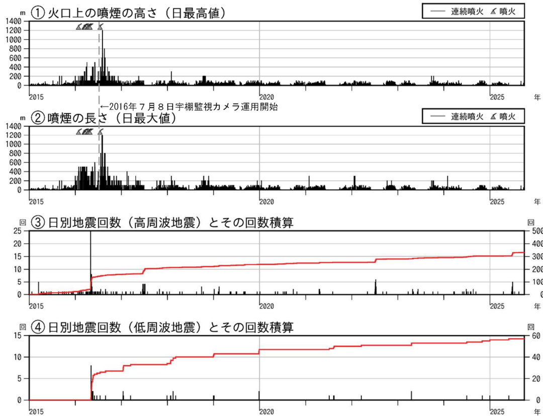
図3 新潟焼山 火山活動経過図（短期）（2015年1月1日～2025年9月30日）
