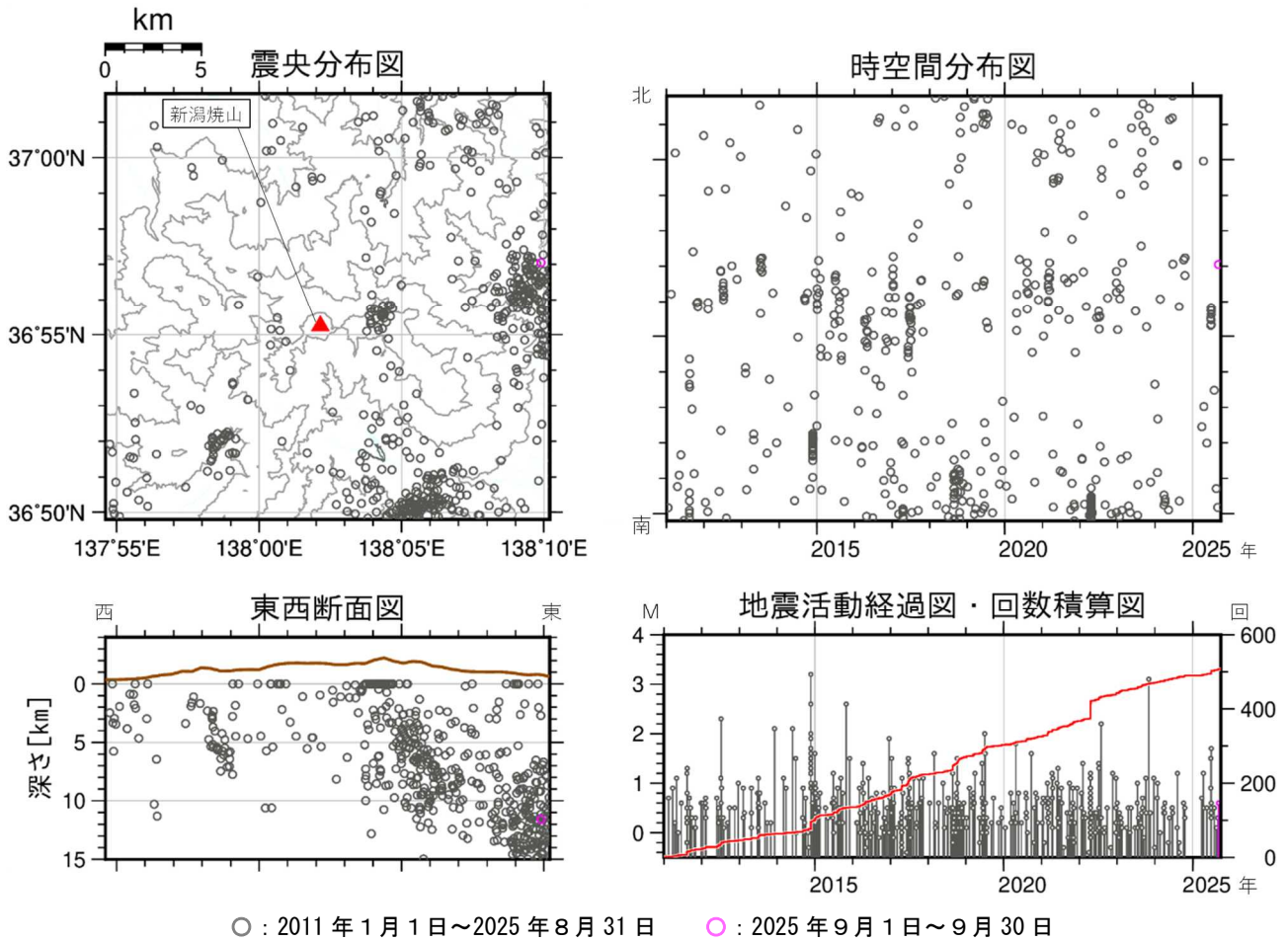
図4 新潟焼山 広域地震観測網による山体・周辺の地震活動（2011 年 1 月 1 日～2025 年 9 月 30 日）
