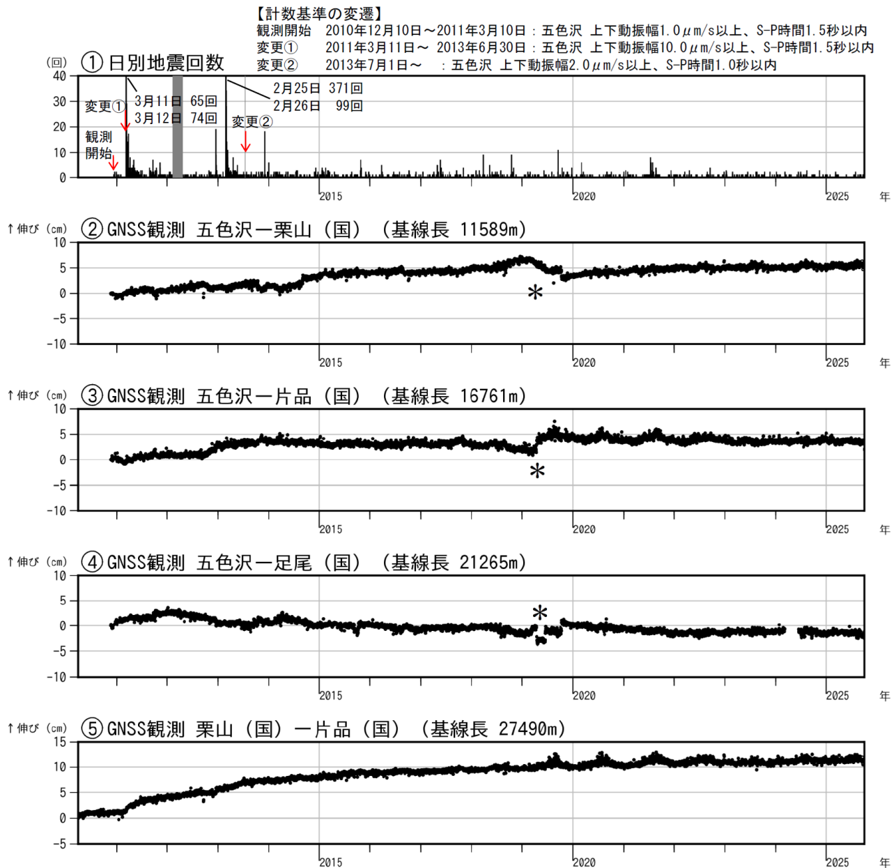
図2 日光白根山 火山活動経過図（2010年4月1日～2025年9月30日）
