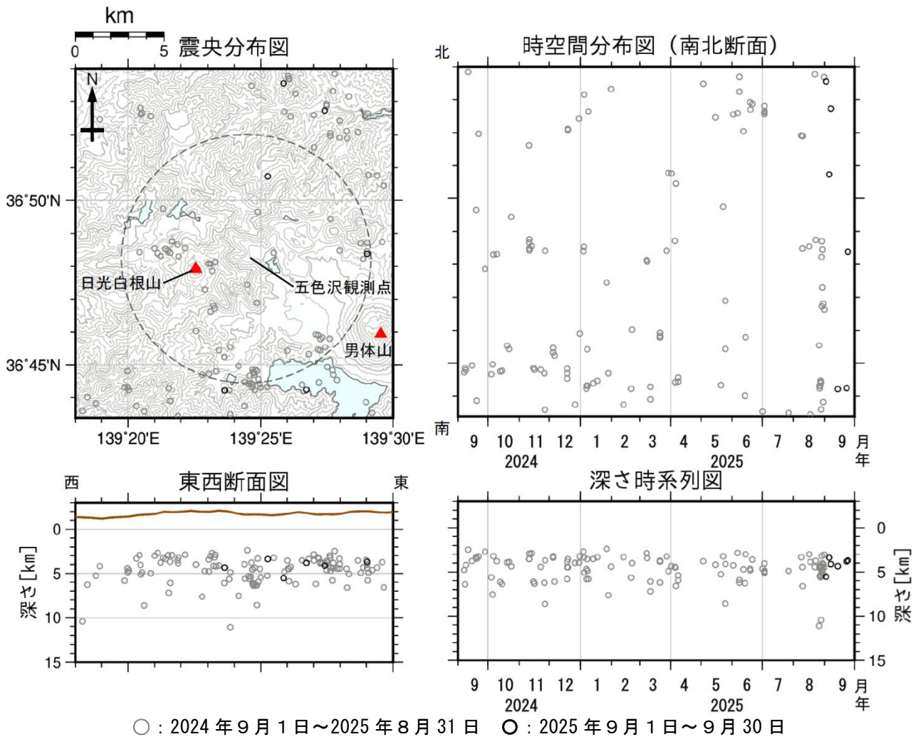
図3 日光白根山 広域地震観測網による山体周辺の地震活動 (2024年9月1日~2025年9月30日)
