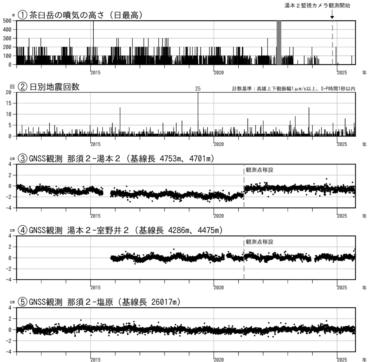
図4 那須岳 火山活動経過図（2012年1月1日～2025年9月30日）
