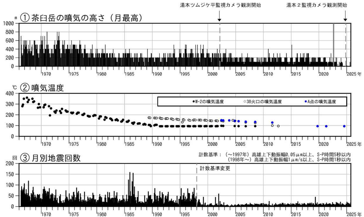
図3-1 那須岳 火山活動経過図（1966年6月～2025年9月）
