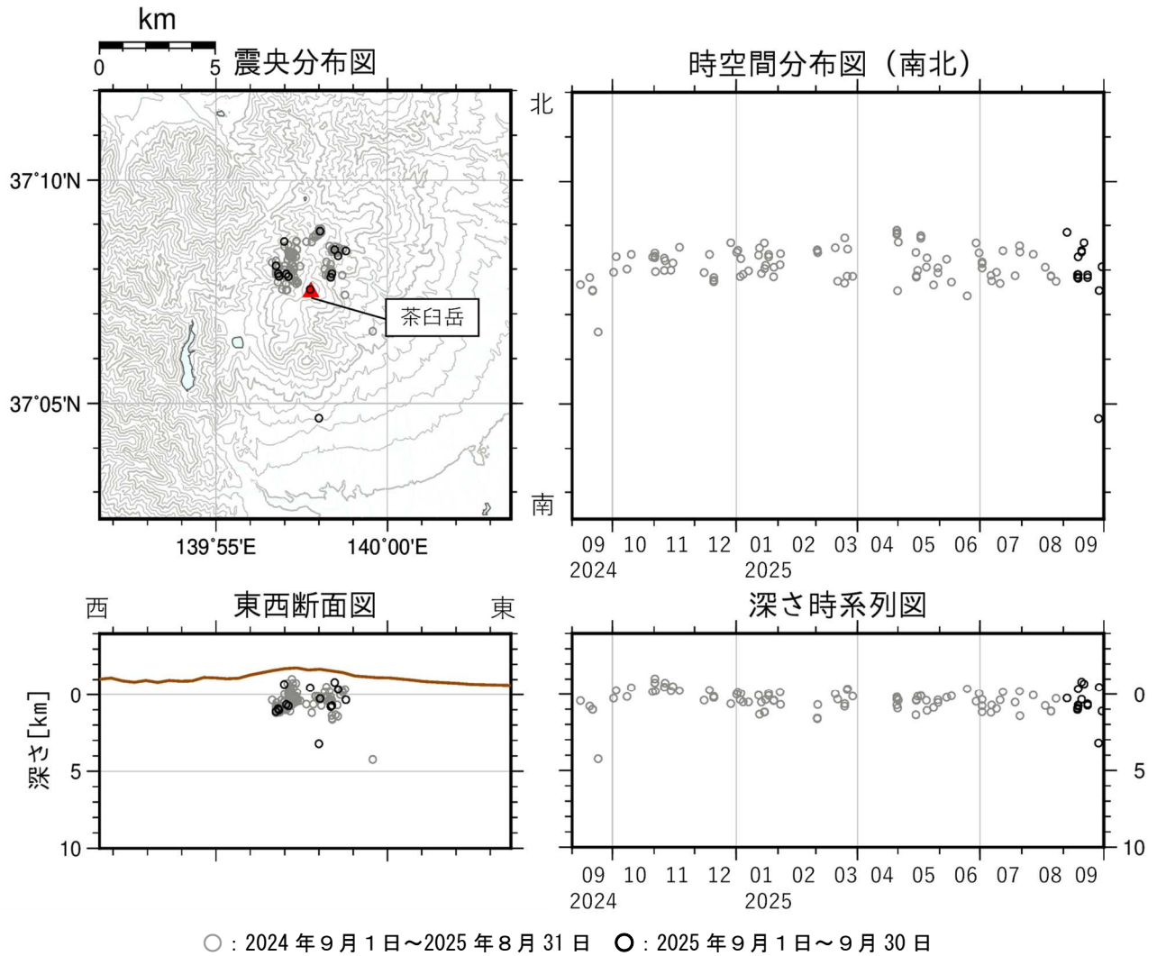
図5 那須岳 震源分布図（2024 年 9 月 1 日～2025 年 9 月 30 日）
