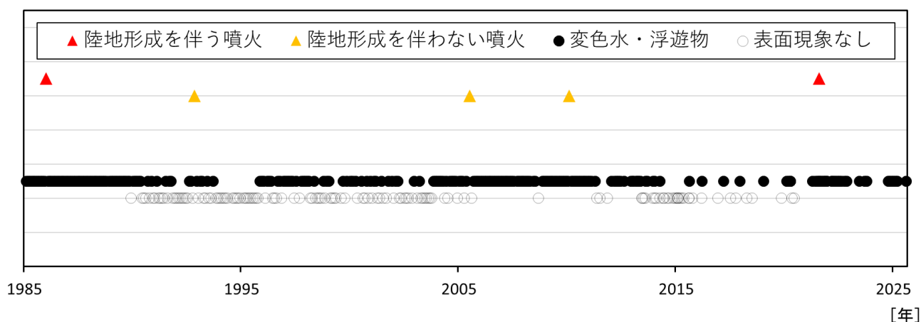
図3 福徳岡ノ場 1985年以降の活動状況
