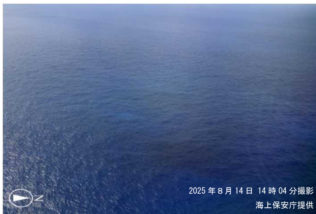
図2 福徳岡ノ場の変色水域
