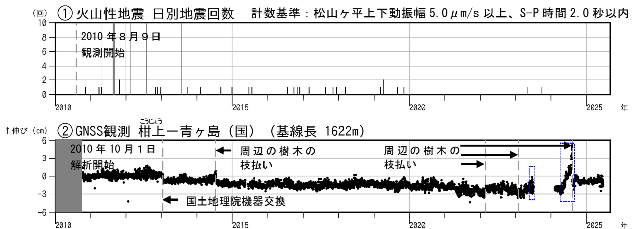
図3 青ヶ島 火山活動経過図（2010年8月9日～2025年8月31日） ① グラフの灰色部分は機器障害による欠測を示す。 ② （国）：国土地理院、図4のGNSS基線②に対応。グラフの空白部分は柑上の障害による欠測を示す。 ・青破線で囲んだ変化は柑上観測点周囲の樹木による影響と考えています。
