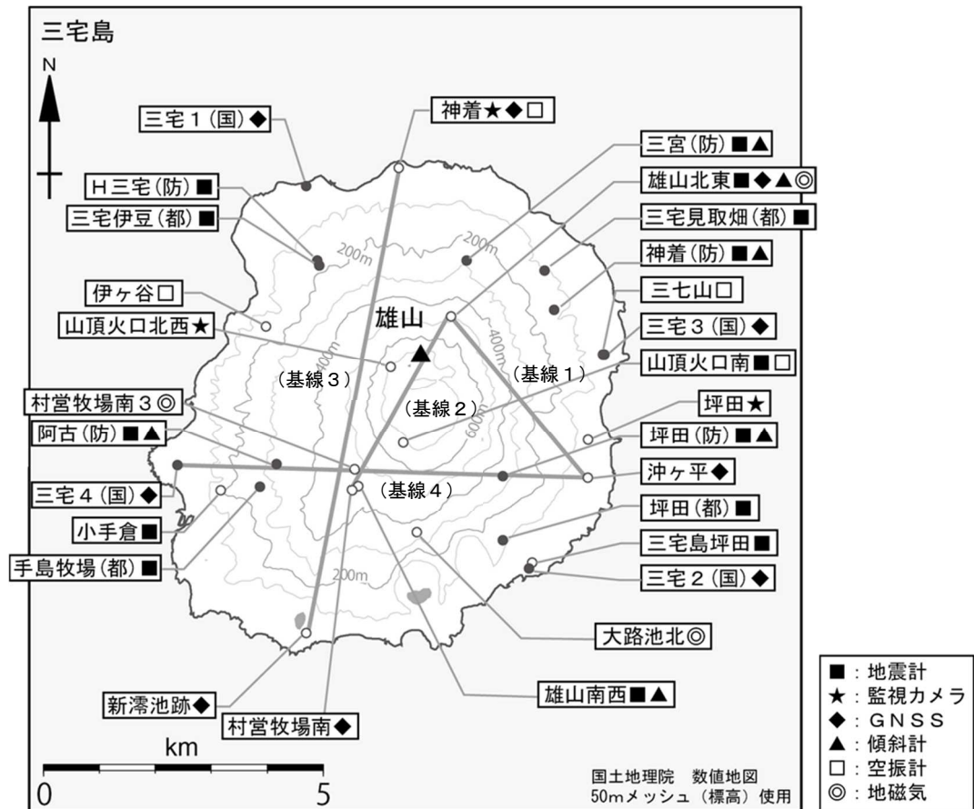
図 11 三宅島 観測点配置図
