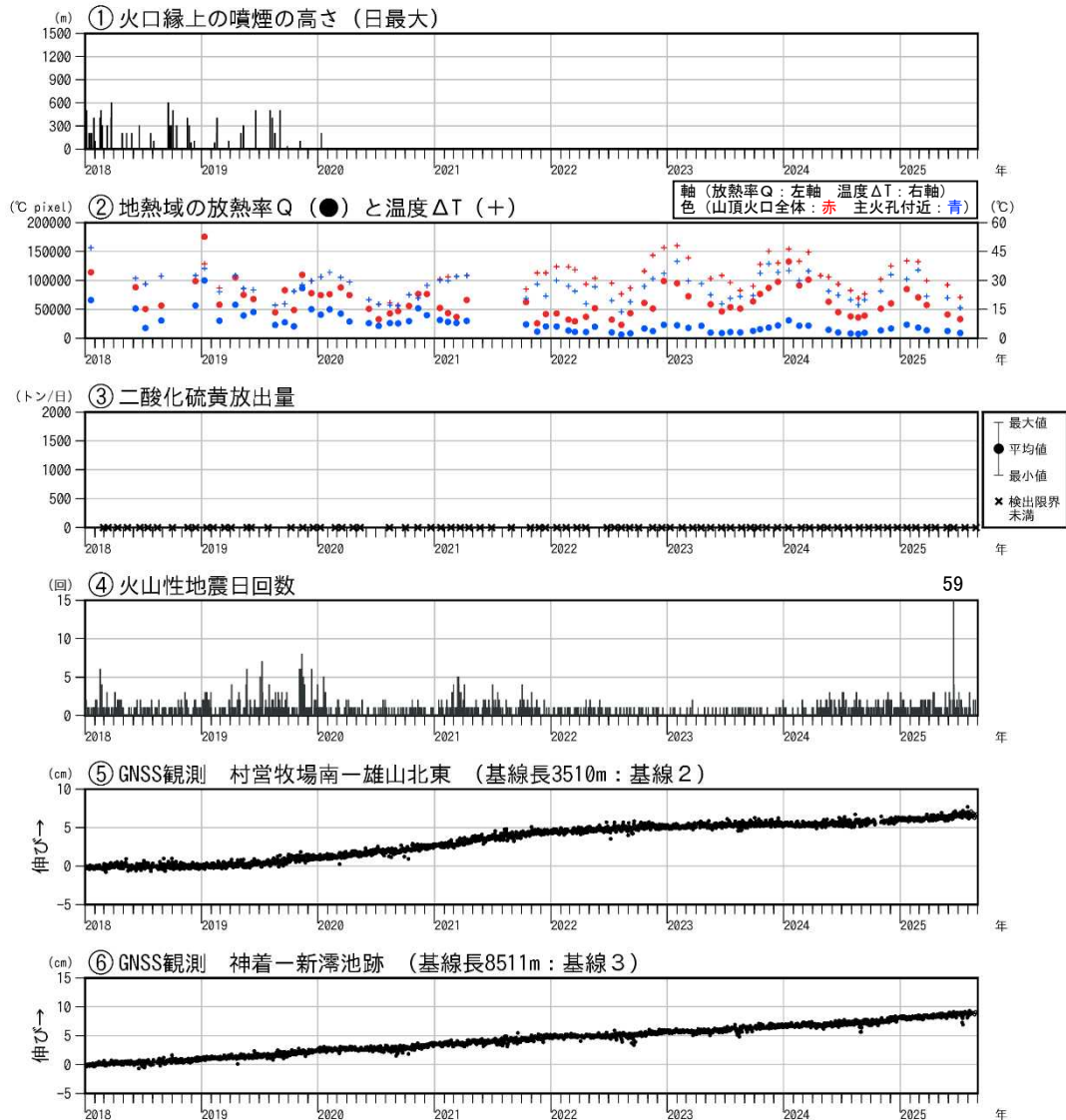
図5 三宅島 火山活動経過図（2018年1月1日～2025年8月31日）
