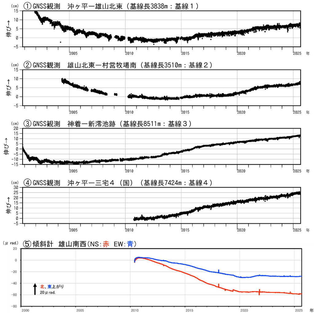
図7 三宅島 GNSS 連続観測及び傾斜計観測結果（2000年10月26日～2025年8月31日）
