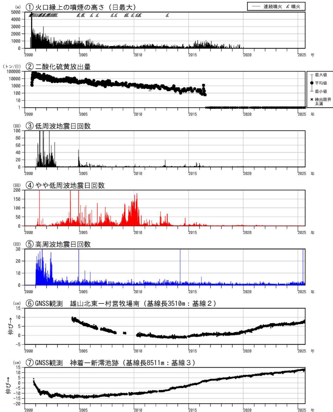
図6 三宅島 長期の火山活動経過図（2000年1月1日～2025年8月31日）
