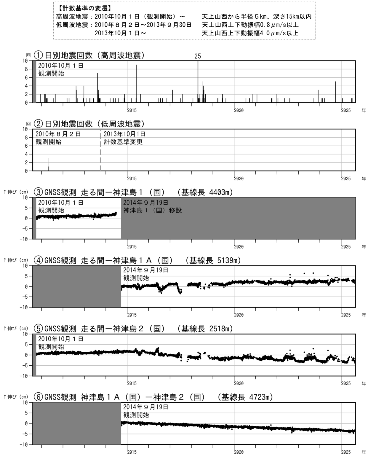
図2 神津島 火山活動経過図(2010年8月2日～2025年8月31日)
