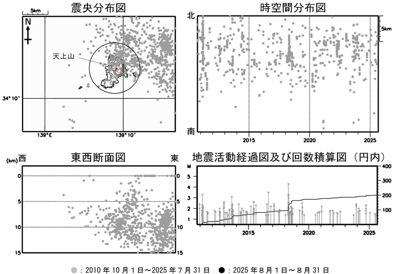
図 3 神津島 広域地震観測網による山体・周辺の地震活動（2010年10月1日～2025年8月31日） 広域地震観測網により震源決定したもので、深さは全て海面以下として決定しています。なお、2020年9月以降については、地震観測点の標高を考慮する等、震源決定の手法を変更しています。 M（マグニチュード）は地震の規模を表し、M1.4以上の地震を示しています。 図中の震源要素は一部暫定値が含まれており、後日変更することがあります。 計数対象（天上山西から半径約5km、深さ約15km以内）以外の地震が含まれるため、図2－①の日別地震回数（高周波地震）とは異なります。 震央分布図中の円は火山性地震の回数の計数対象（天上山西から半径5km、深さ15km以内）の範囲を示しています。 ・地震活動は低調に経過しました。
