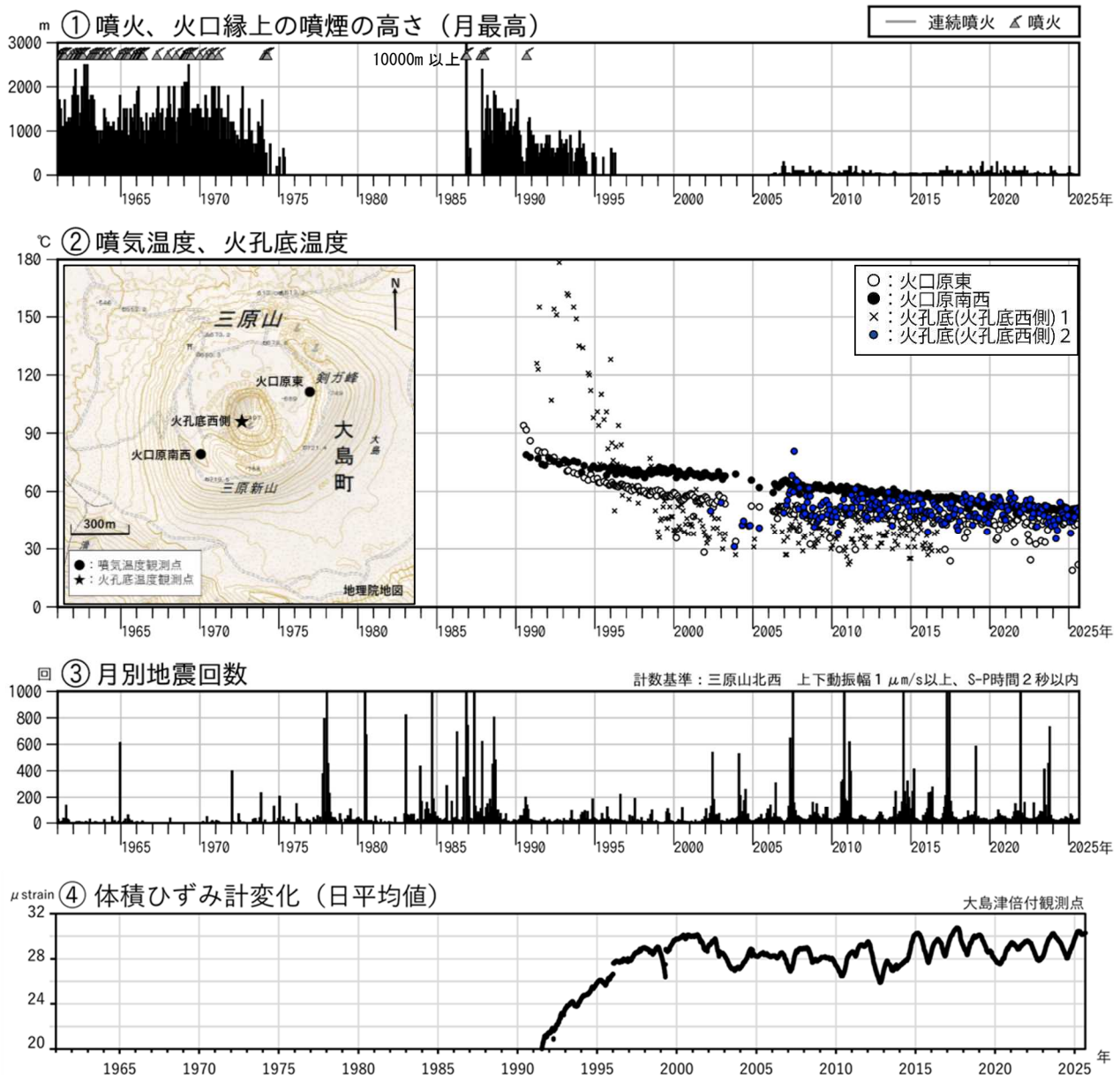
図1 伊豆大島 長期間の火山活動経過図（1961年1月～2025年8月）
