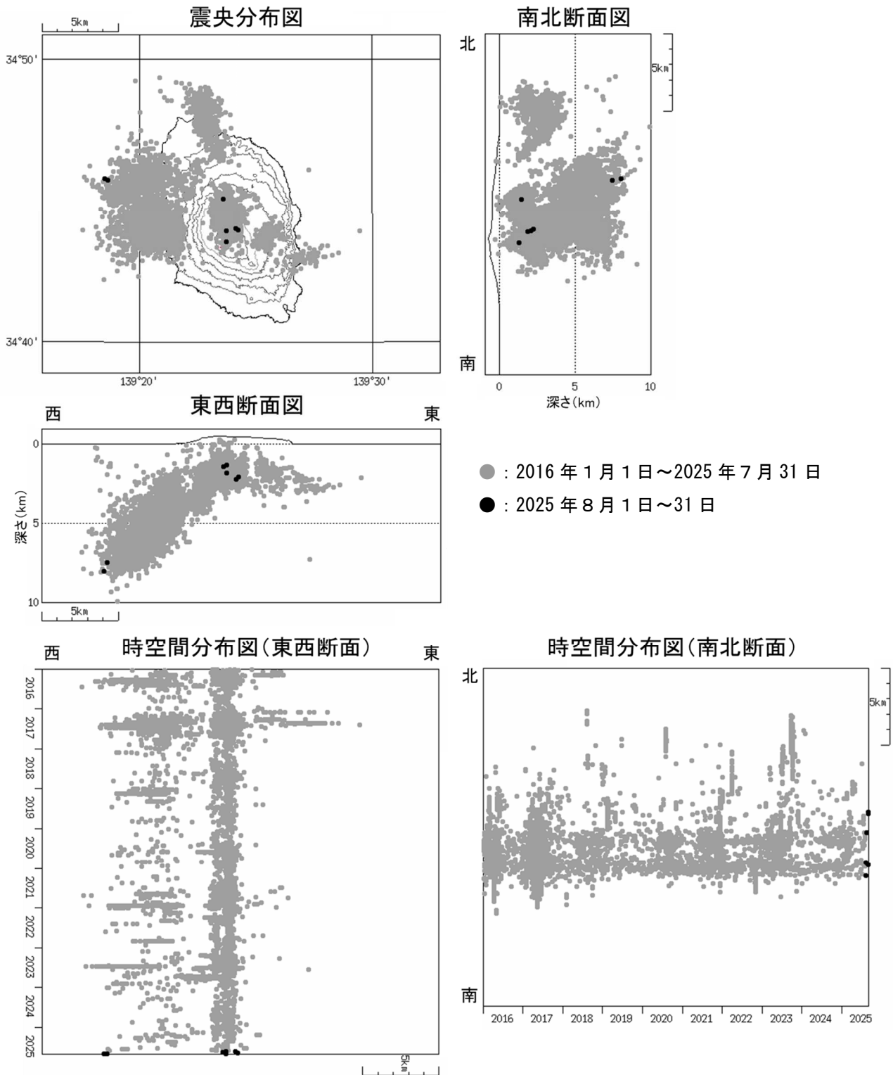
図 4 伊豆大島 震源分布図（2016 年 1 月 1 日～2025 年 8 月 31 日）
