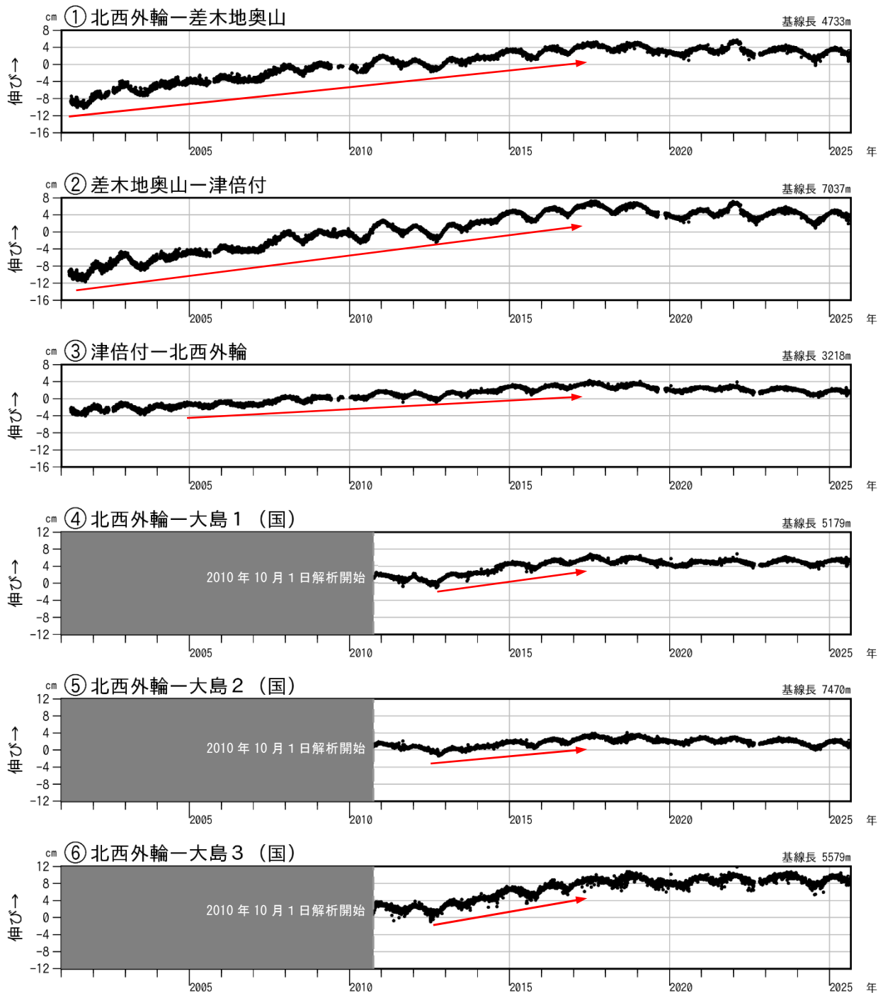
図3-1 伊豆大島 GNSS 連続観測による基線長変化(2001年1月～2025年8月)
