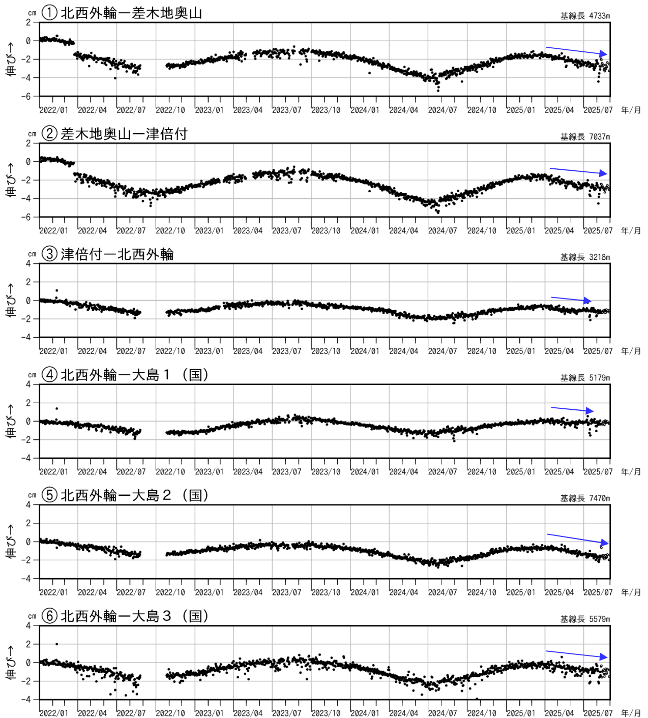
図 3-2 伊豆大島 GNSS 連続観測による基線長変化(2022 年 1 月～2025 年 8 月)
