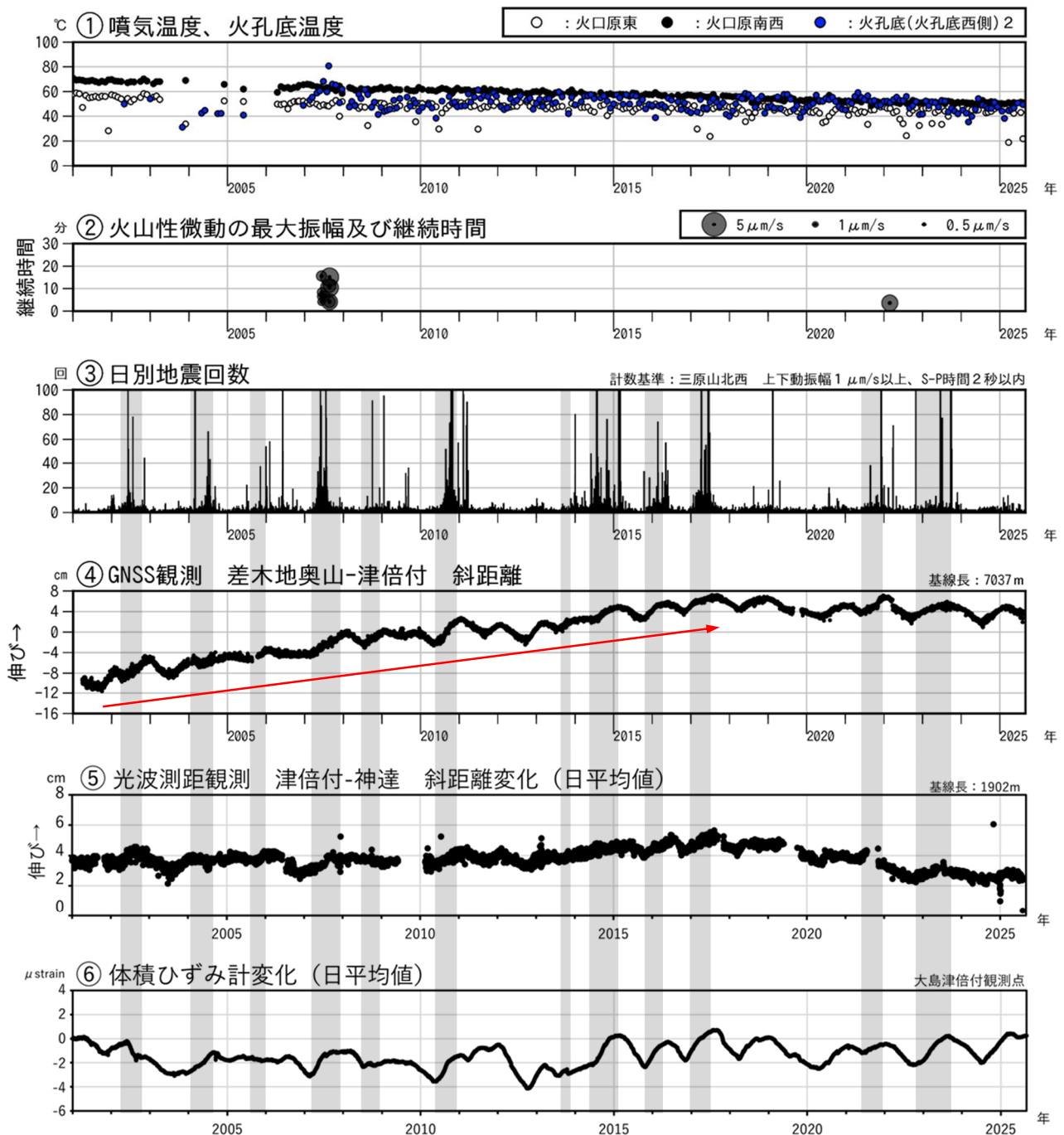
図2 伊豆大島 最近の火山活動経過図（2001年1月～2025年8月）
