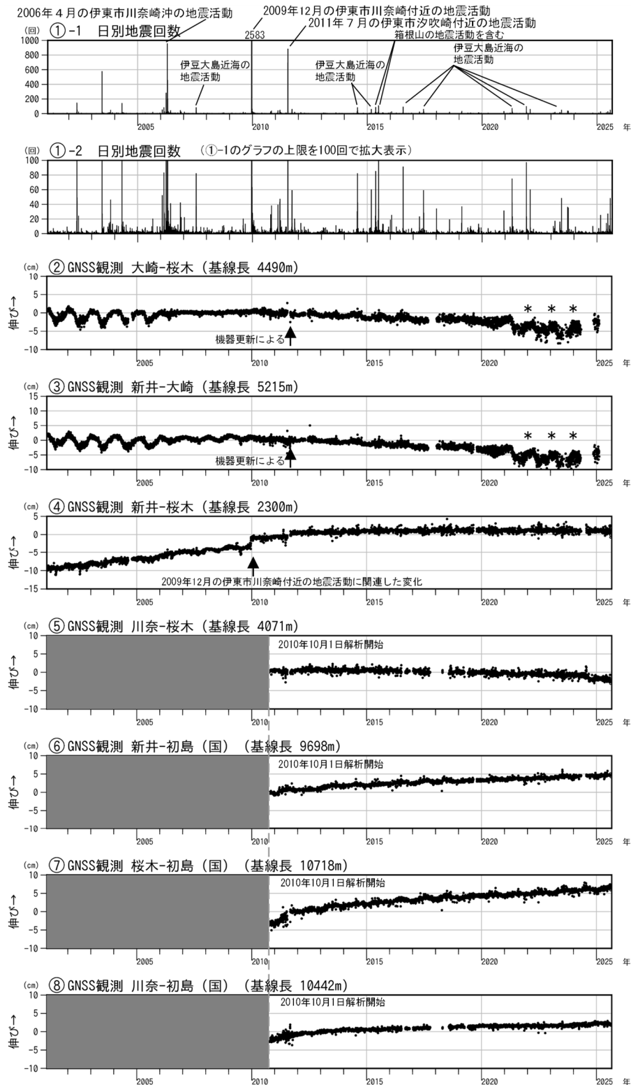
図3 伊豆東部火山群 火山活動経過図（2001年2月1日～2025年8月31日）
