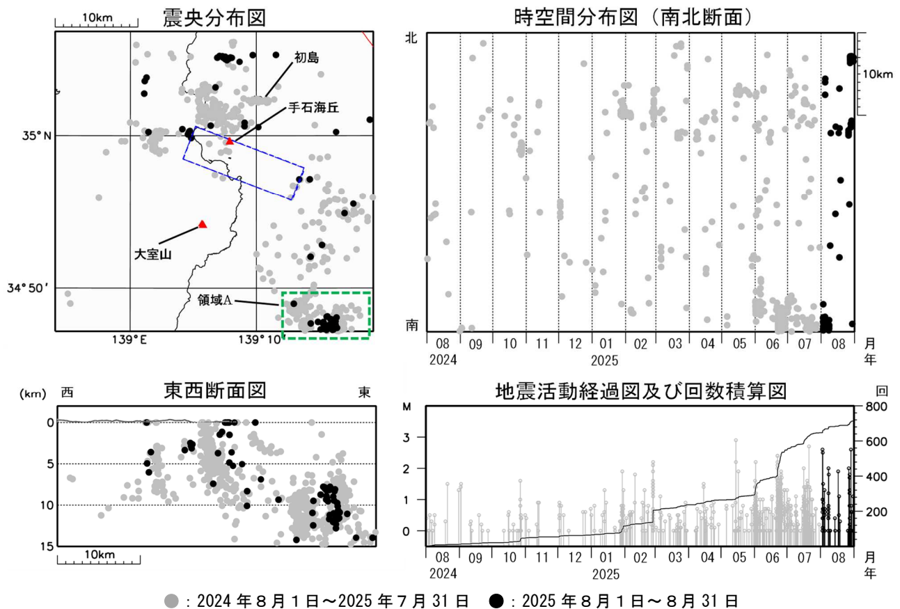
図2 伊豆東部火山群 広域地震観測網による震源分布図（2024 年 8 月 1 日～2025 年 8 月 31 日） 図中の領域は群発地震活動の発生する可能性がある範囲（火口が出現する可能性のある範囲）を示しています。 https://www.data.jma.go.jp/vois/data/filing/level/PDF/level_316.pdf 広域地震観測網により震源決定したもので、深さは全て海面以下として決定しています。 M（マグニチュード）は地震の規模を表し、M0.0 以上を表示しています。 図中の震源要素は一部暫定値が含まれており、後日変更することがあります。 この図では、関係機関の地震波形を一元的に処理し、地震観測点の標高を考慮する等した手法で得られた震源を用いています。
