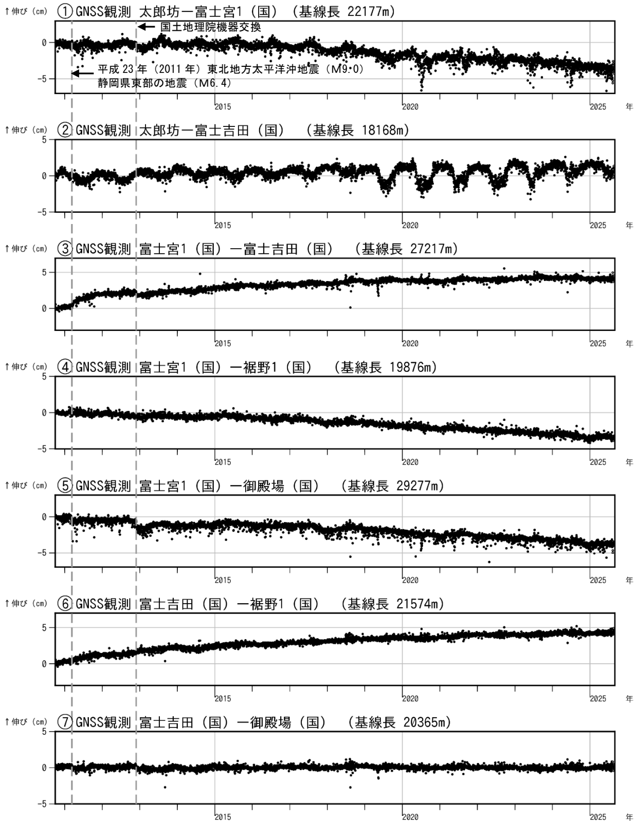
図4 富士山 GNSS 連続観測による基線長変化 (2010 年 10 月 1 日～2025 年 8 月 31 日) (国): 国土地理院 「平成 23 年 (2011 年) 東北地方太平洋沖地震」及び 2011 年 3 月 15 日に発生した静岡県東部の地震 (M 6.4) によるステップ状の変化を補正しています。 ①～⑦は図5の GNSS 基線①～⑦に対応しています。
