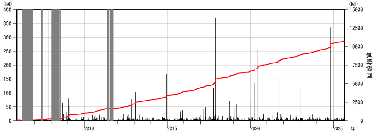
図3 白山 日別地震回数と積算回数（2005年12月1日～2025年8月31日） 図の灰色部分は機器障害による欠測期間。
