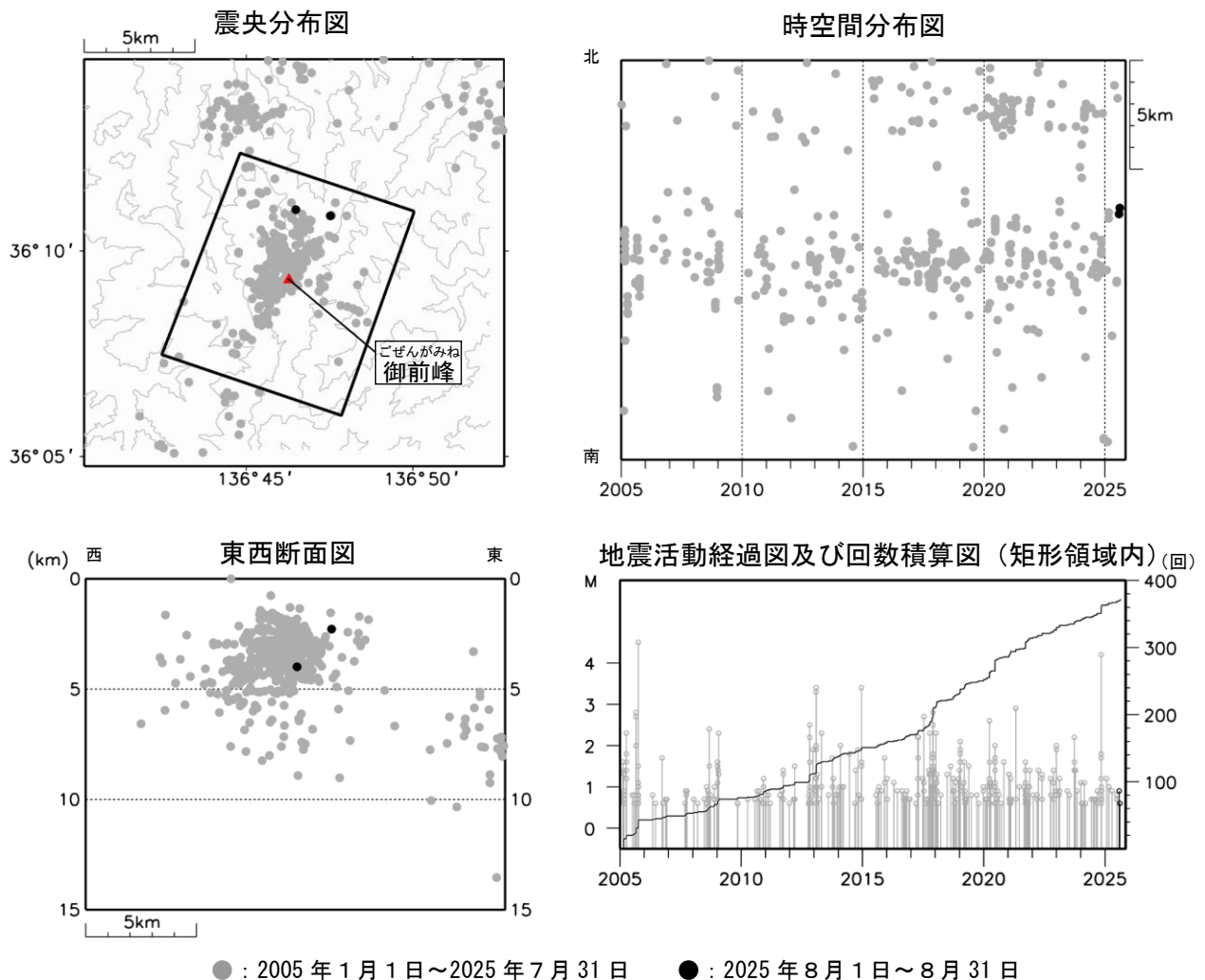
図4 白山 広域地震観測網による山体・周辺の地震活動（2005年1月1日～2025年8月31日） 広域地震観測網により震源決定したもので、深さは全て海面以下として決定しています。なお、2020年9月以降については、地震観測点の標高を考慮する等、震源決定の手法を変更しています。 M（マグニチュード）は地震の規模を表します。M0.6以上の地震を表示しています。 図中の震源要素は一部暫定値を含んでおり、後日変更することがあります。 ・今期間、白山付近の地震活動は低調に経過しました。
