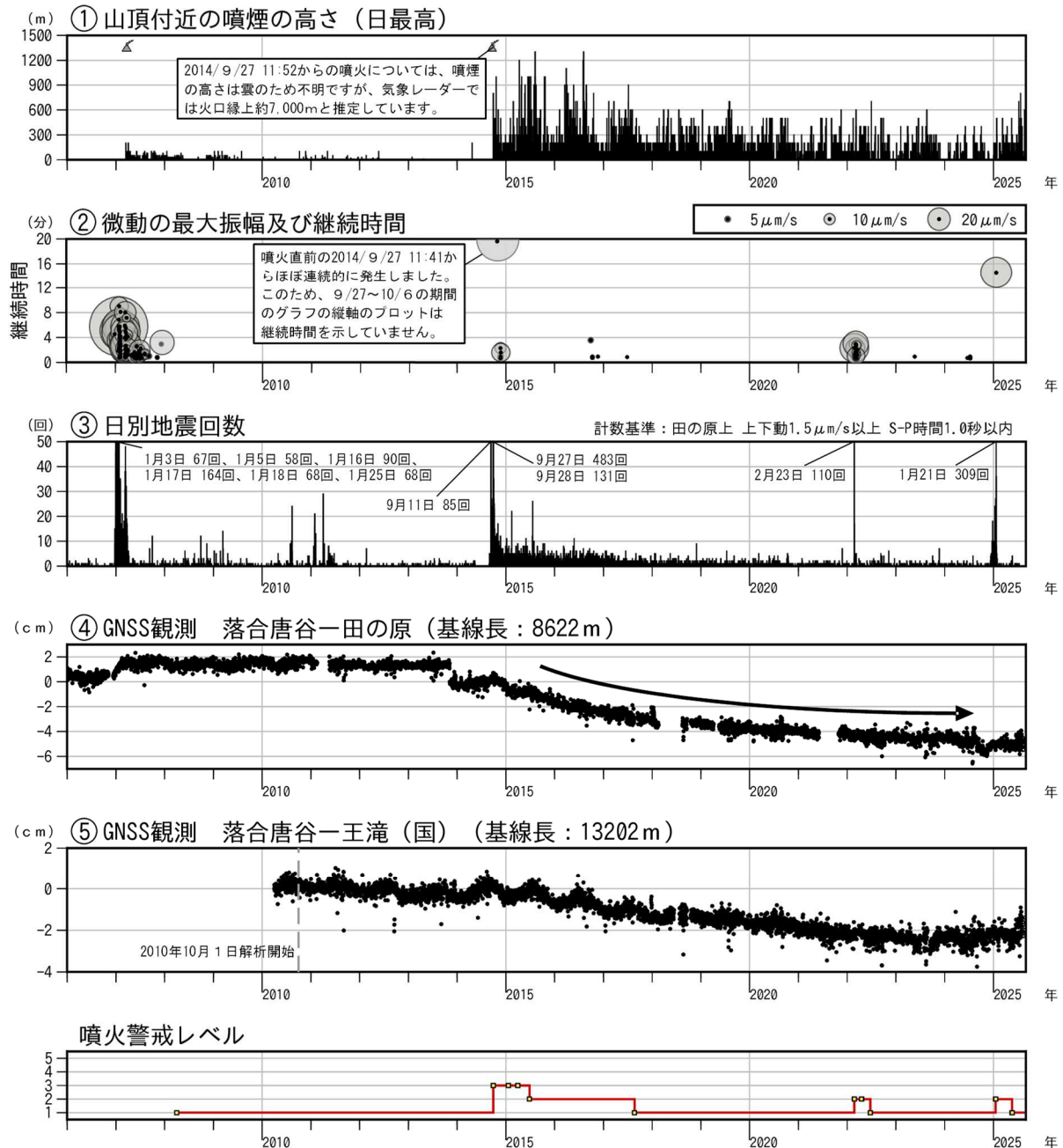
図1 御嶽山 長期間の火山活動経過図（2006年1月1日～2025年8月31日）
