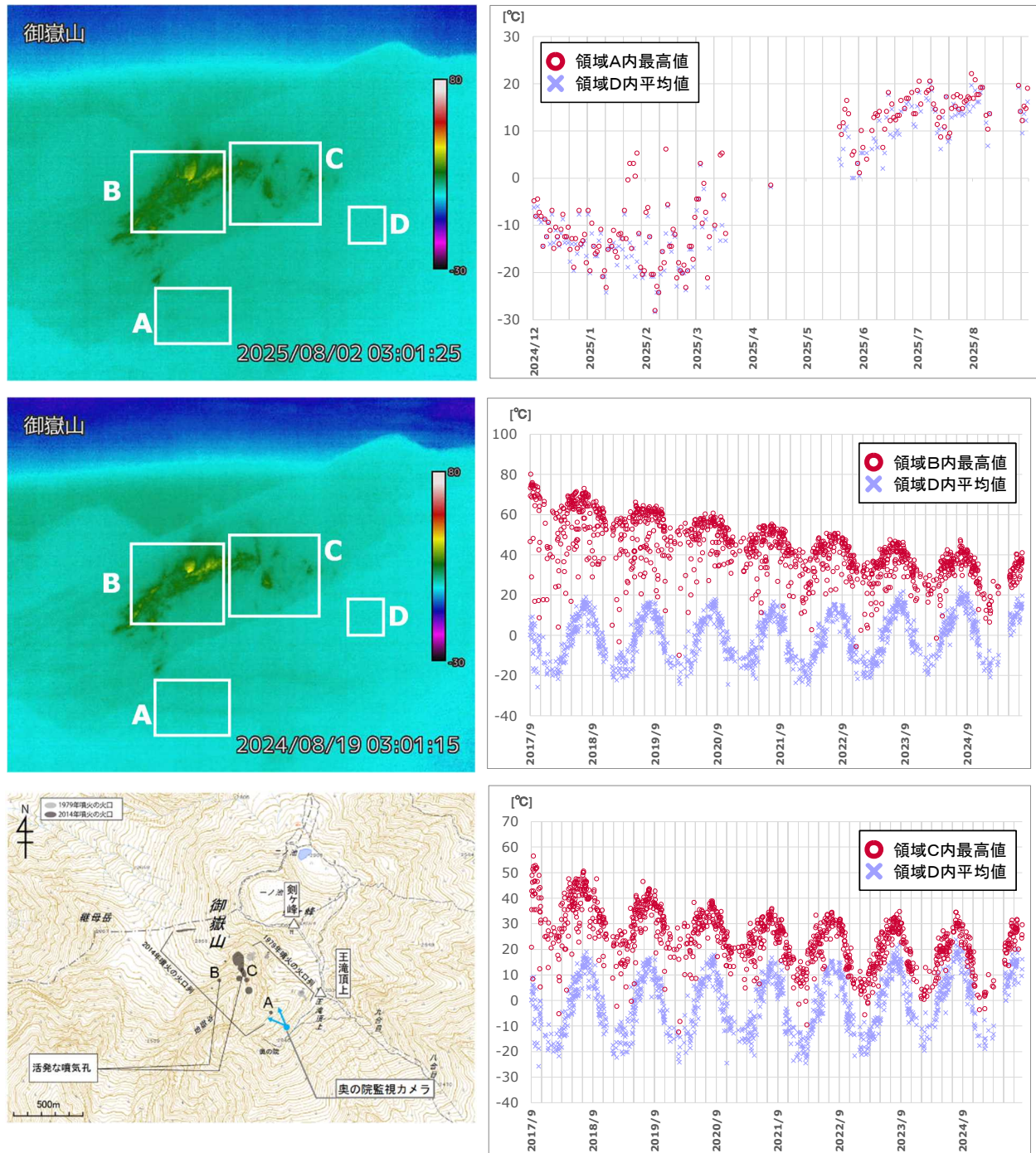
図3 御嶽山 奥の院赤外熱映像カメラによる地獄谷火口における最高温度の推移 (2017年9月13日～2025年8月31日)
