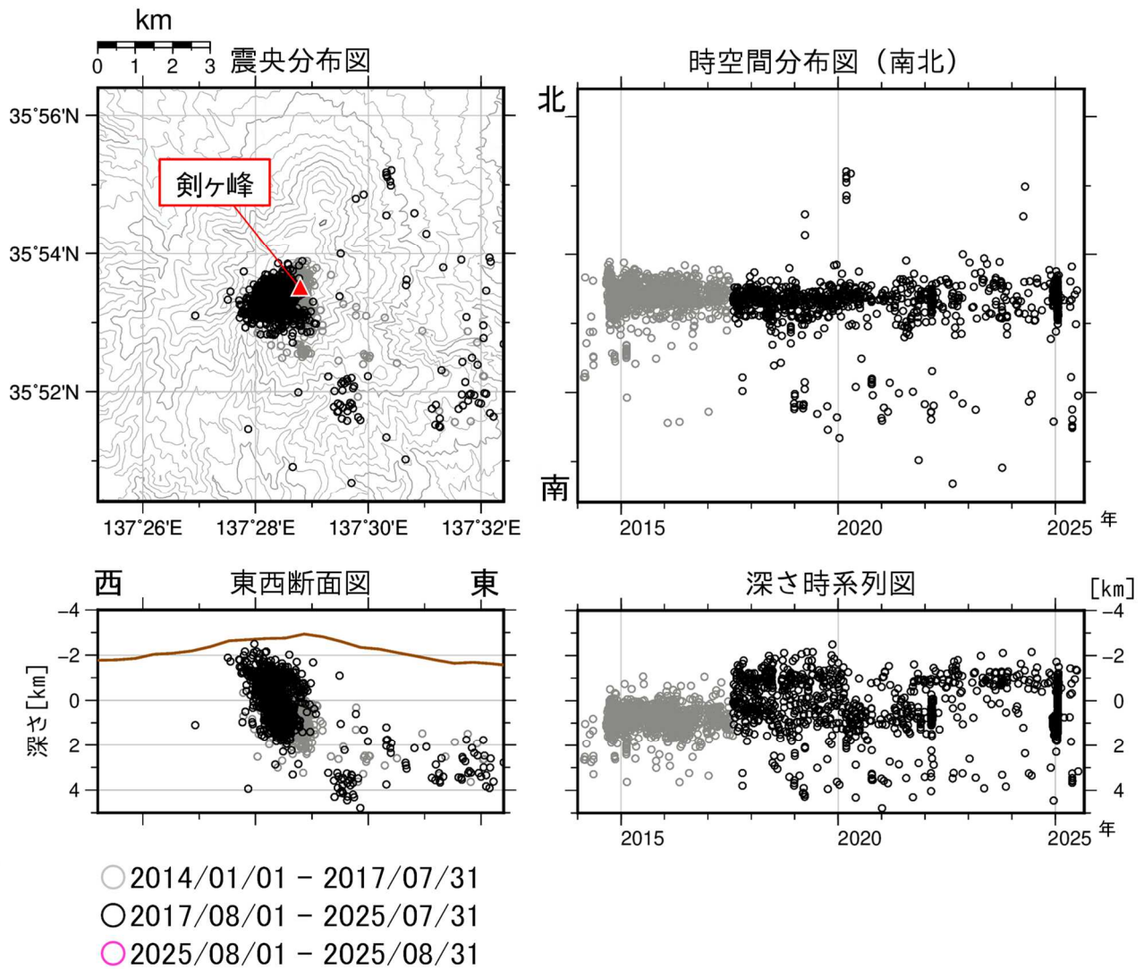
図5 御嶽山 震源分布図（2014年1月1日～2025年8月31日） 2017年8月1日以降の震源分布は、震源計算に使用する観測点を新たに追加して再計算したものを示しています。 観測点の移動状況により、求まる震源の数の減少や位置の精度低下が生じる場合があります。
