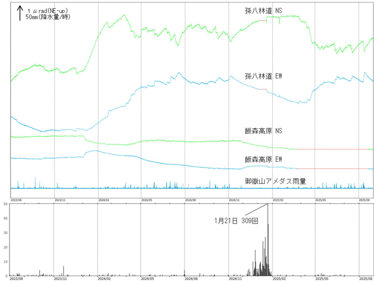
図8 御嶽山 傾斜変動と日別地震回数の推移（2023年8月1日～2025年8月31日）
