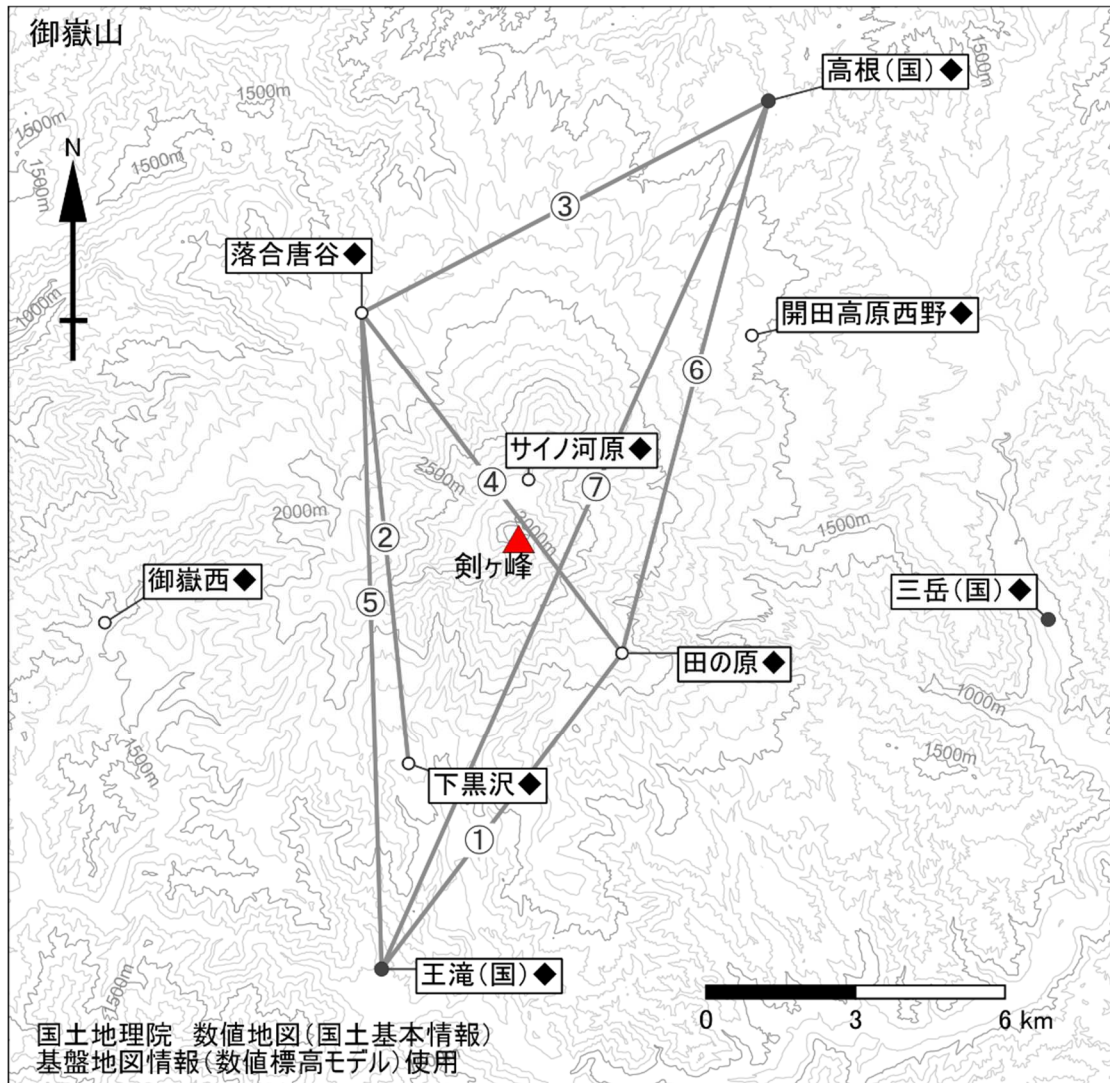
図7 御嶽山 GNSS 連続観測点と基線番号
