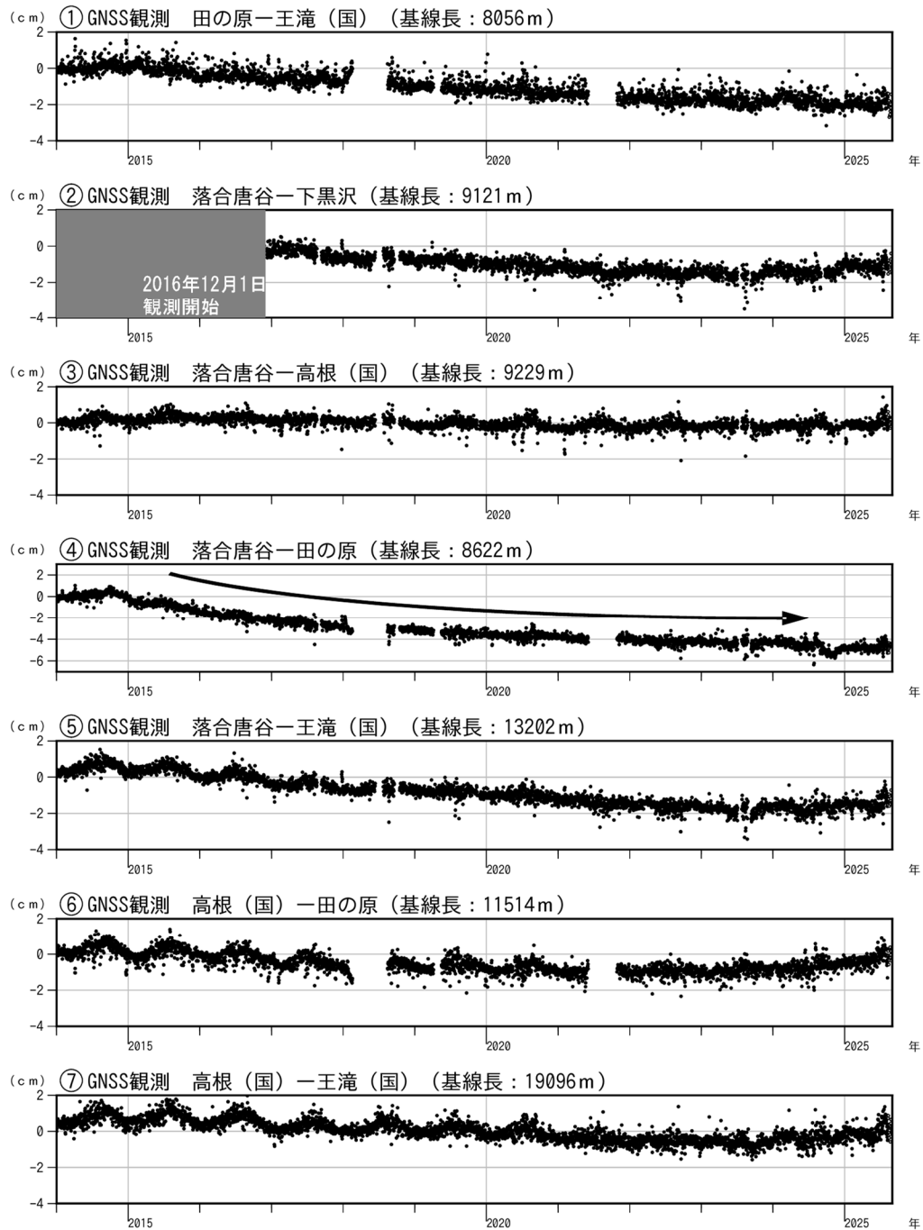
図6 御嶽山 GNSS 連続観測結果（2014 年 1 月 1 日～2025 年 8 月 31 日）
