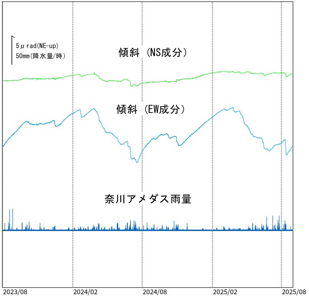
図4 乗鞍岳 三本滝観測点における傾斜データ（2023年8月1日～2025年8月31日） ・傾斜計による観測では、火山活動によるとみられる変動は認められません。
