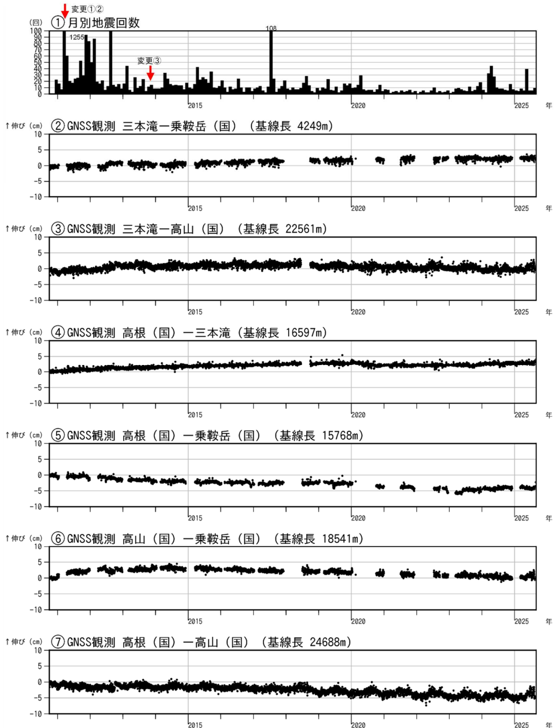
図2 乗鞍岳 火山活動経過図（2010年10月1日～2025年8月31日）
