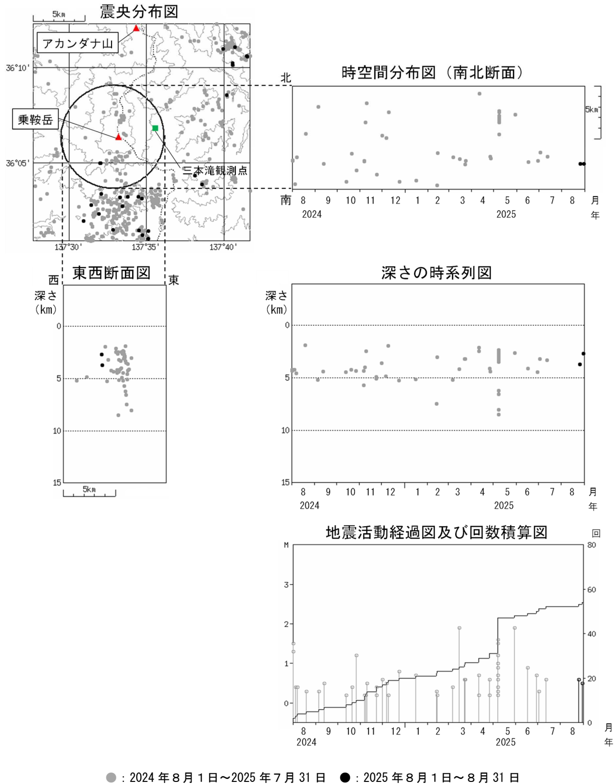
図3 乗鞍岳 広域地震観測網による山体・周辺の地震活動(2024年8月1日～2025年8月31日)
