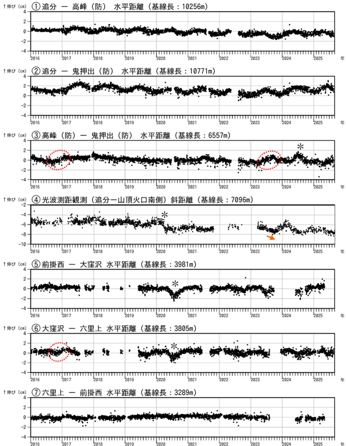
図7-1 浅間山 GNSS 連続観測及び光波測距観測結果(2016年1月1日～2025年8月31日)
