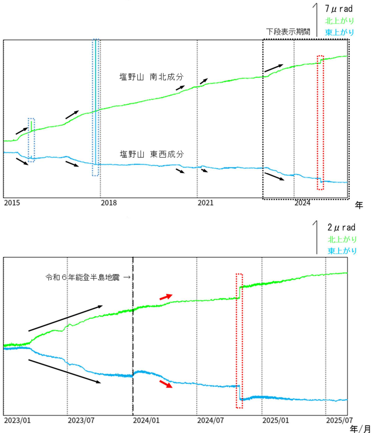
図 6 浅間山 塩野山観測点における傾斜データ（2015 年 1 月 1 日～2025 年 8 月 31 日）
