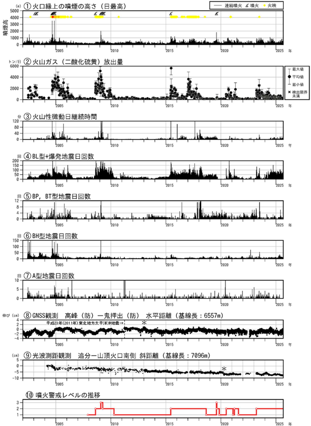
図3 浅間山 長期火山活動経過図（2002年1月1日～2025年8月31日）
