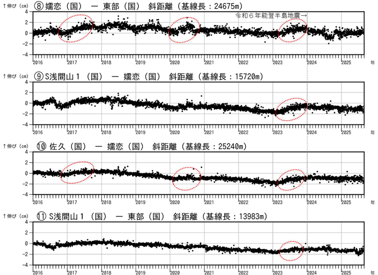
図7-2 浅間山 GNSS 連続観測結果(2016年1月1日～2025年8月31日)
