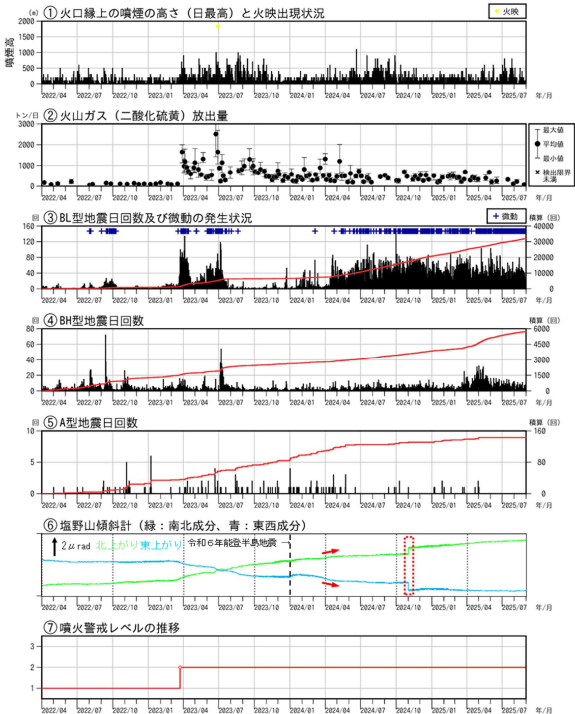
図2 浅間山 短期火山活動経過図（2022年4月1日～2025年8月31日）
