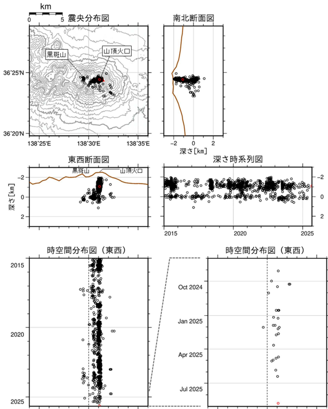
図5 浅間山 震源分布図（2015年1月1日～2025年8月31日）
