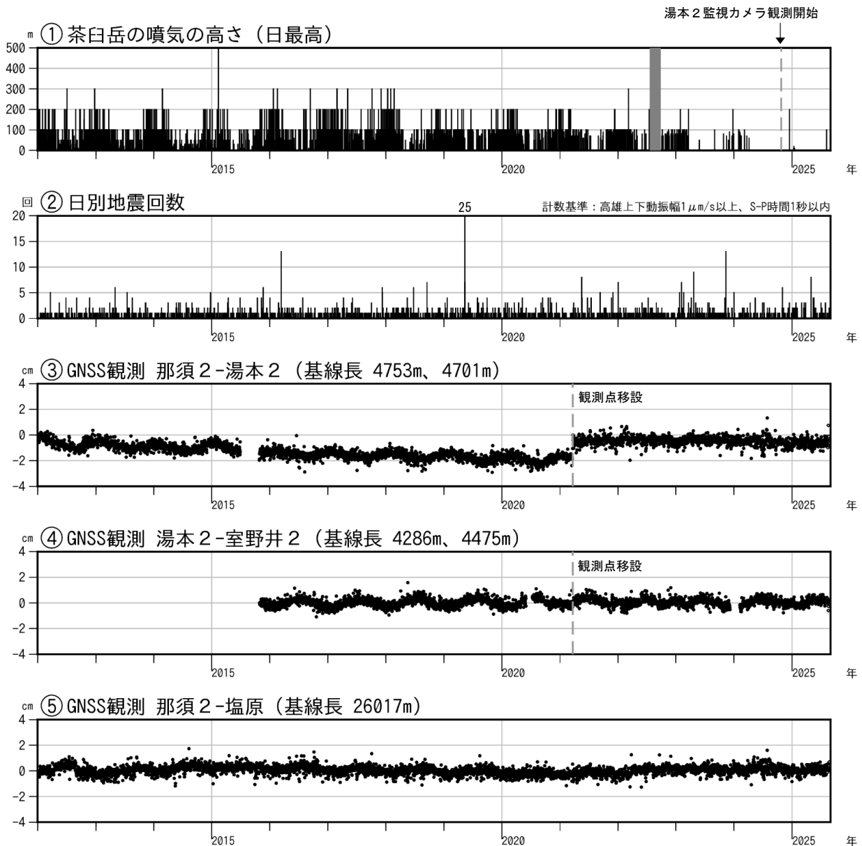
図4 那須岳 火山活動経過図（2012年1月1日～2025年8月31日）
