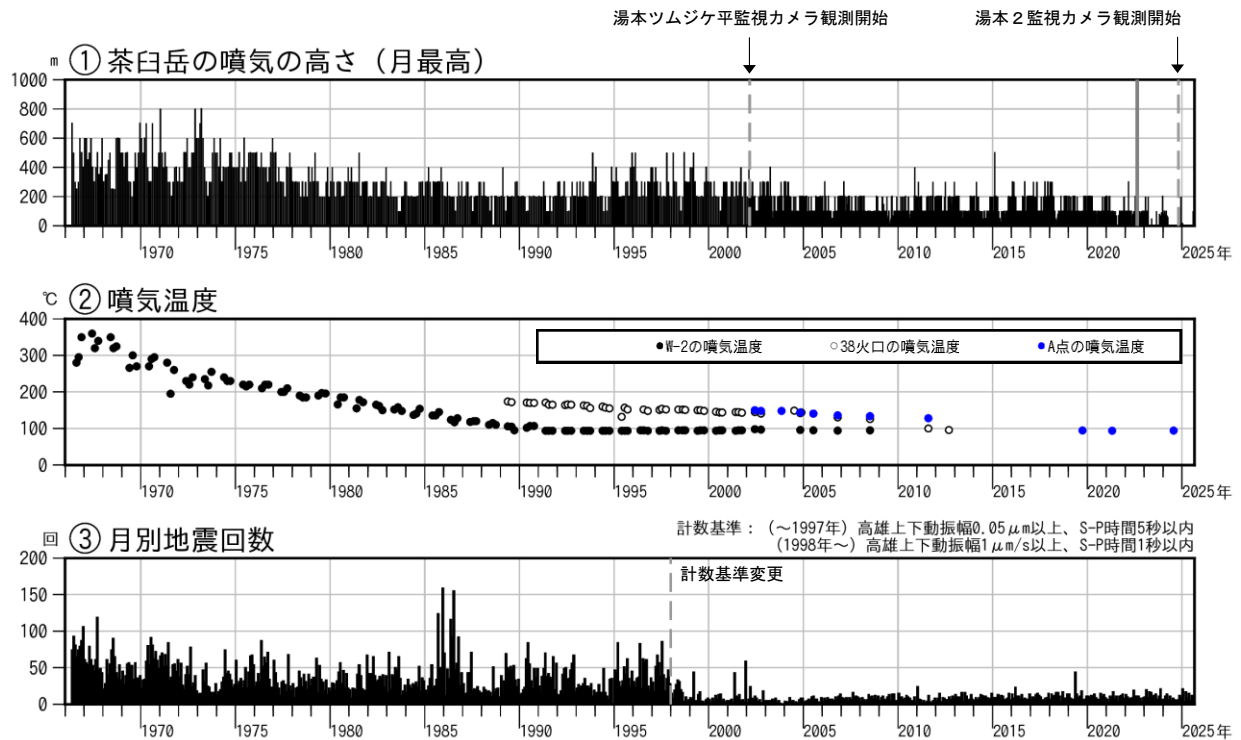
図3-1 那須岳 火山活動経過図（1966年6月～2025年8月）
