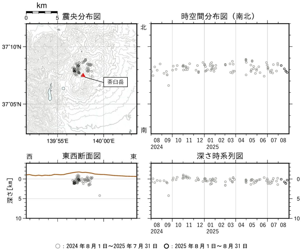
図5 那須岳 震源分布図（2024 年 8 月 1 日～2025 年 8 月 31 日）
