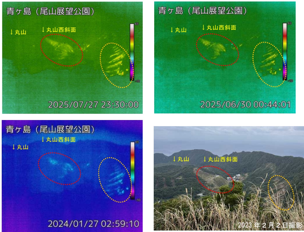
図2 青ヶ島 カルデラ内の地表面温度の状況（左上、右上、左下：尾山展望公園監視カメラによる、右下：2023年2月2日に撮影した同場所からの写真） ・地熱活動（赤点線及び黄色点線で示した範囲）に変化は認められません。
