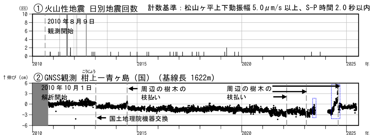
図3 青ヶ島 火山活動経過図（2010年8月9日～2025年7月31日） ① グラフの灰色部分は機器障害による欠測を示す。 ② （国）：国土地理院、図4のGNSS基線②に対応。グラフの空白部分は柑上の障害による欠測を示す。 ・青破線で囲んだ変化は柑上観測点周囲の樹木による影響と考えています。
