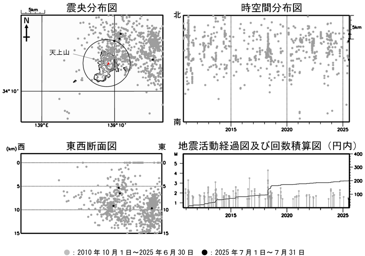
図 3 神津島 広域地震観測網による山体・周辺の地震活動（2010年10月1日～2025年7月31日） 広域地震観測網により震源決定したもので、深さは全て海面以下として決定しています。なお、2020 年 9 月以降については、地震観測点の標高を考慮する等、震源決定の手法を変更しています。 M（マグニチュード）は地震の規模を表し、M1.4 以上の地震を示しています。 図中の震源要素は一部暫定値が含まれており、後日変更することがあります。 計数対象（天上山西から半径約 5 km、深さ約 15km 以内）以外の地震が含まれるため、図 2－①の日別地震回数（高周波地震）とは異なります。 震央分布図中の円は火山性地震の回数の計数対象（天上山西から半径 5 km、深さ 15km 以内）の範囲を示しています。 ・地震活動は低調に経過しました。
