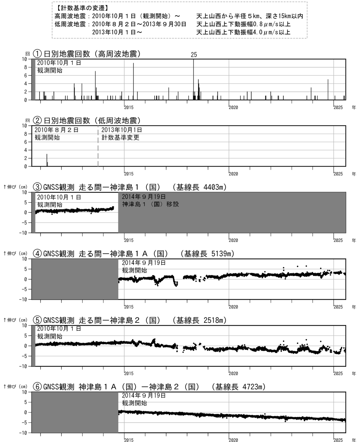
図2 神津島 火山活動経過図(2010年8月2日～2025年7月31日)
