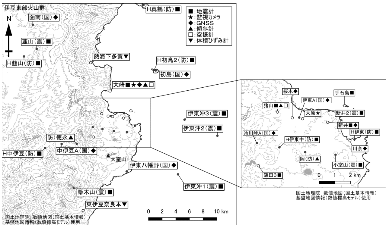
図5 伊豆東部火山群 観測点配置図
