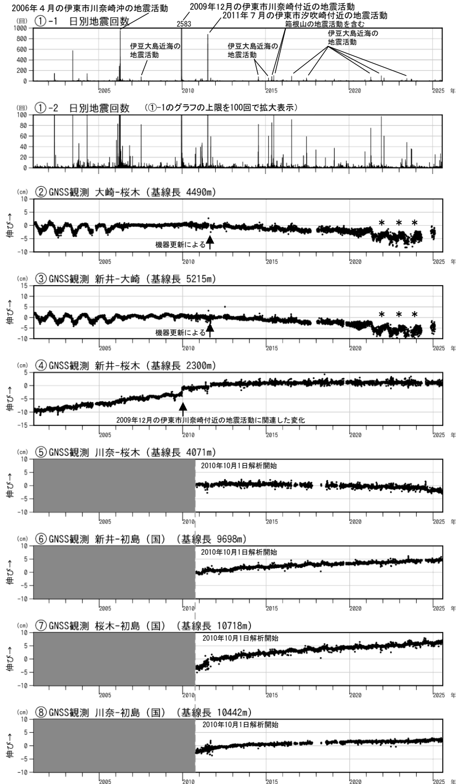
図3 伊豆東部火山群 火山活動経過図（2001年2月1日～2025年7月31日）
