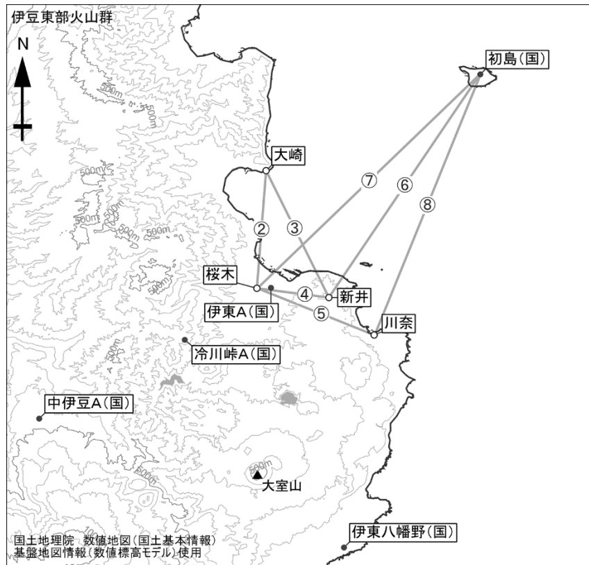
図4 伊豆東部火山群 GNSS 連続観測点配置図 図中の GNSS 基線②～⑧は図3の②～⑧に対応しています。
