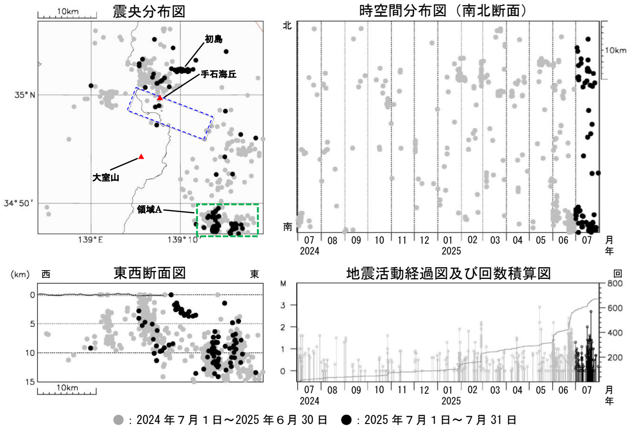
図2 伊豆東部火山群 広域地震観測網による震源分布図（2024年7月1日～2025年7月31日） □の領域は群発地震活動の発生する可能性がある範囲（火口が出現する可能性のある範囲）を示しています。 https://www.data.jma.go.jp/vois/data/filing/level/PDF/level_316.pdf 広域地震観測網により震源決定したもので、深さは全て海面以下として決定しています。 M（マグニチュード）は地震の規模を表し、M0.0以上を表示しています。 図中の震源要素は一部暫定値が含まれており、後日変更することがあります。 この図では、関係機関の地震波形を一元的に処理し、地震観測点の標高を考慮する等した手法で得られた震源を用いています。
