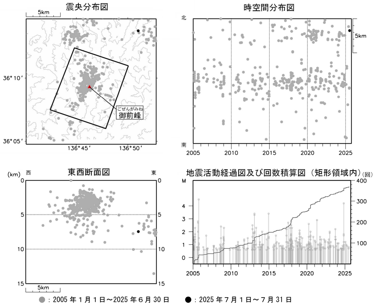
図4 白山 広域地震観測網による山体・周辺の地震活動（2005年1月1日～2025年7月31日） 広域地震観測網により震源決定したもので、深さは全て海面以下として決定しています。なお、2020年9月以降については、地震観測点の標高を考慮する等、震源決定の手法を変更しています。 M（マグニチュード）は地震の規模を表します。M0.6以上の地震を表示しています。 図中の震源要素は一部暫定値を含んでおり、後日変更することがあります。 ・今期間、白山付近の地震活動は低調に経過し、矩形領域内に震源が求まる地震はありませんでした。
