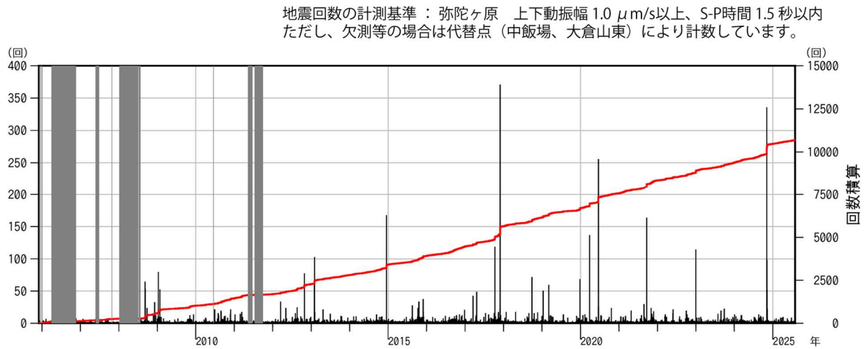
図3 白山 日別地震回数と積算回数（2005年12月1日～2025年7月31日） 図の灰色部分は機器障害による欠測期間。
