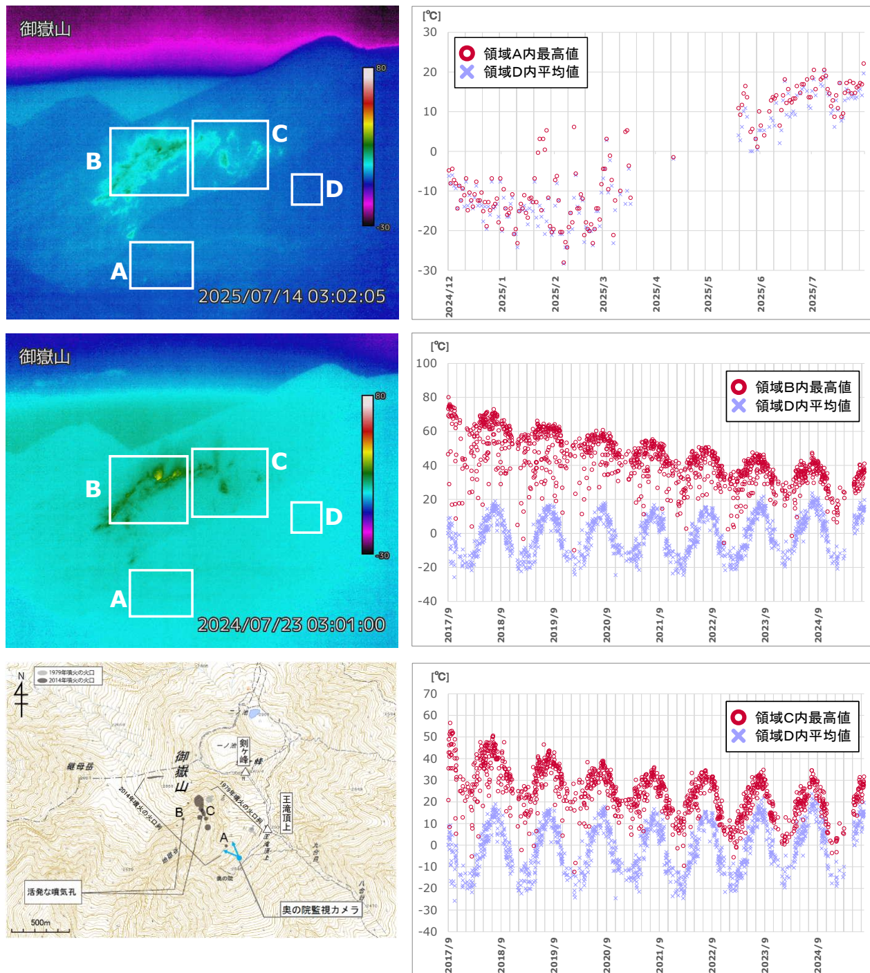
図3 御嶽山 奥の院赤外熱映像カメラによる地獄谷火口における最高温度の推移 (2017年9月13日～2025年7月31日)
