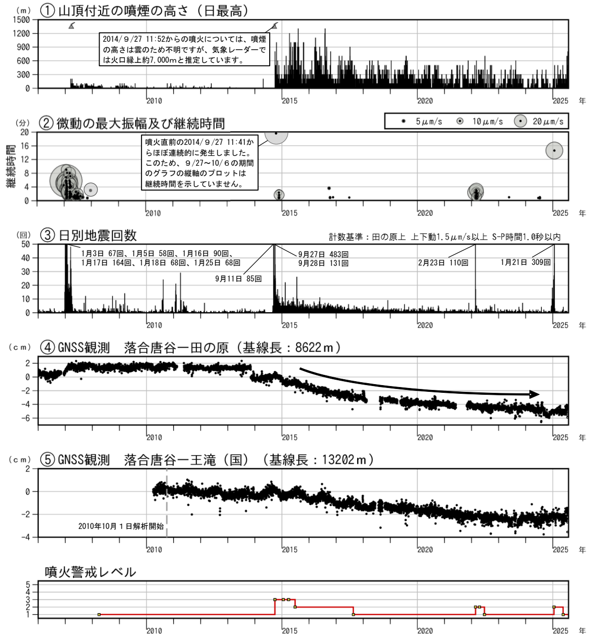
図1 御嶽山 長期間の火山活動経過図（2006年1月1日～2025年7月31日）
