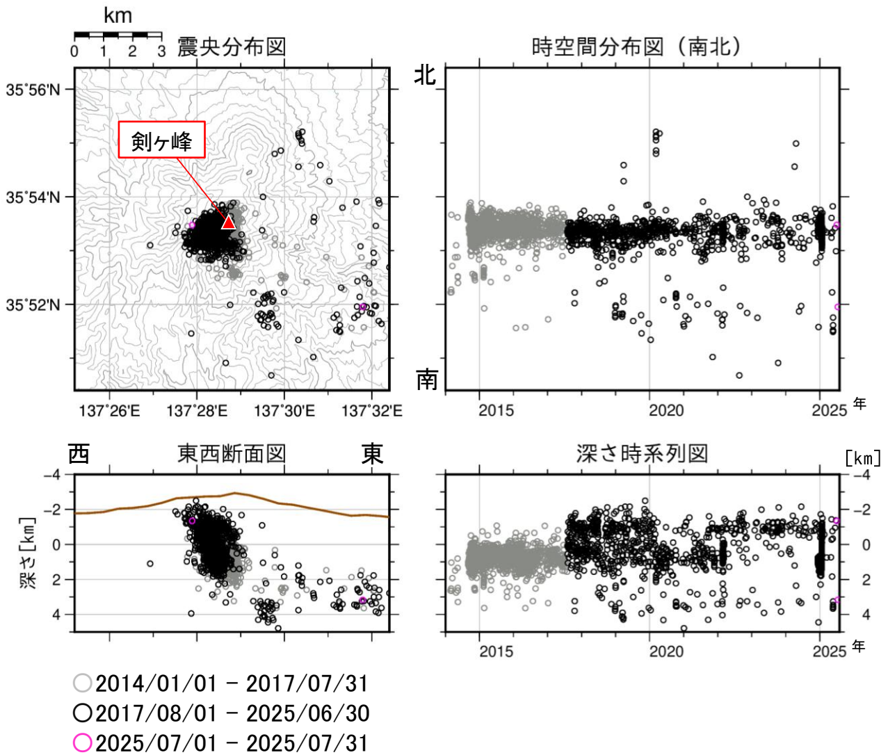
図 4 御嶽山 震源分布図（2014 年 1 月 1 日～2025 年 7 月 31 日）
