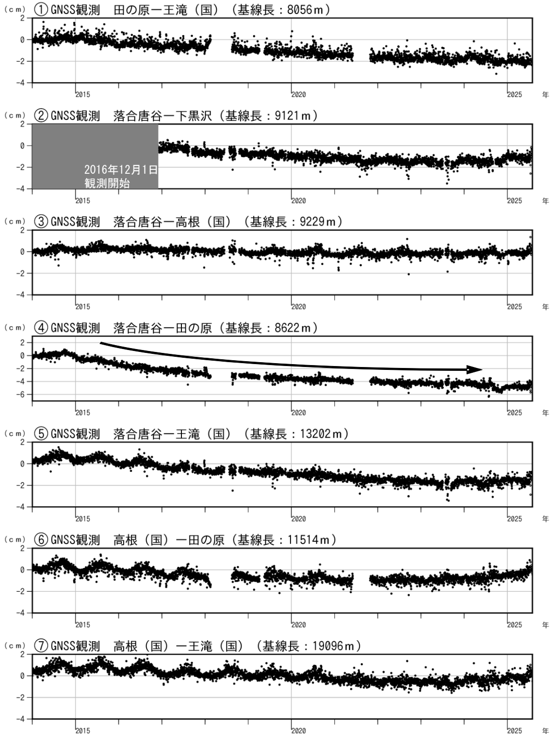
図5 御嶽山 GNSS 連続観測結果（2014 年 1 月 1 日～2025 年 7 月 31 日）
