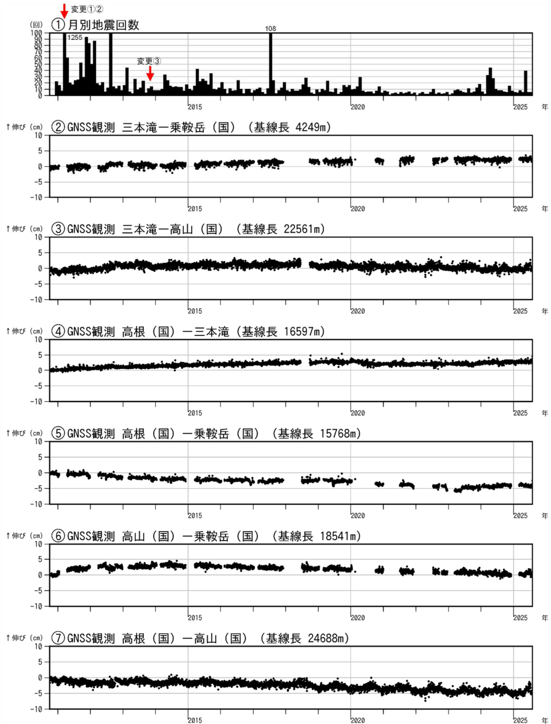
図2 乗鞍岳 火山活動経過図（2010年10月1日～2025年7月31日）
