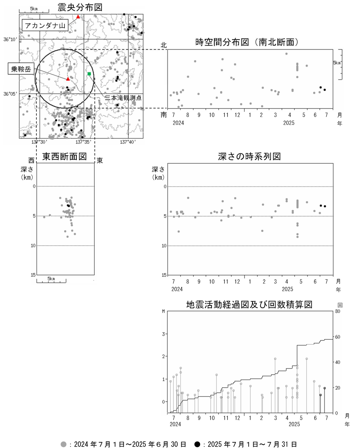
図3 乗鞍岳 広域地震観測網による山体・周辺の地震活動(2024 年 7 月 1 日～2025 年 7 月 31 日)
