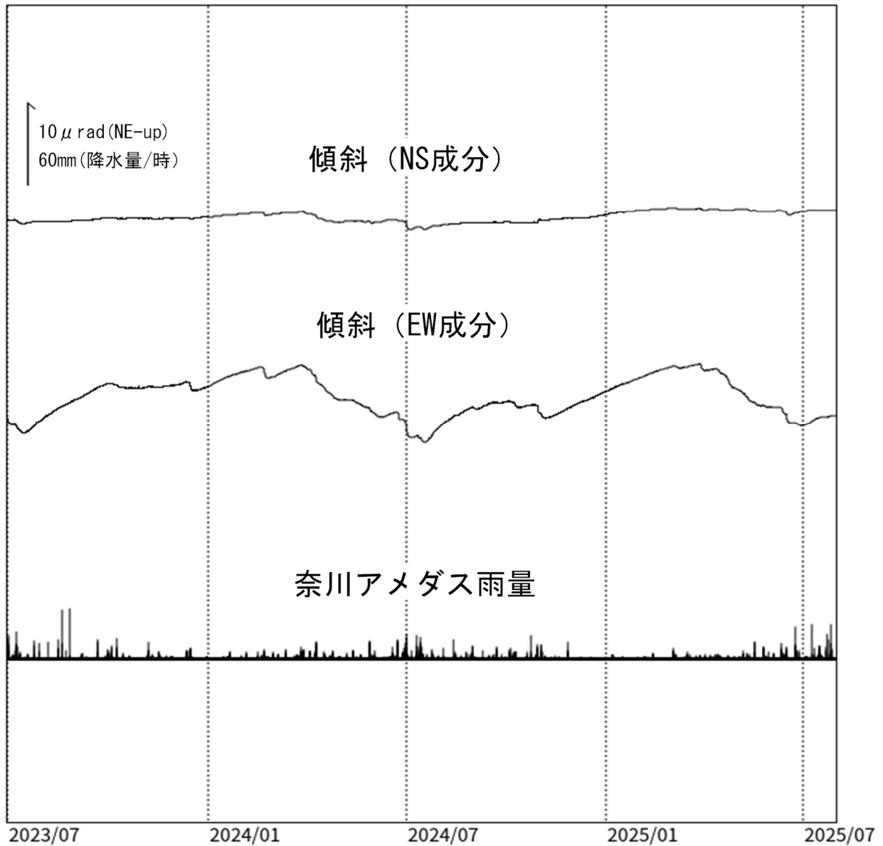
図4 乗鞍岳 三本滝観測点における傾斜データ（2023年7月1日～2025年7月31日） ・傾斜計による観測では、火山活動によるとみられる変動は認められません。
