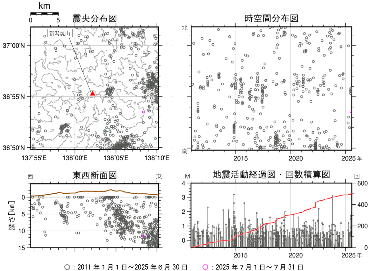
図 4 新潟焼山 広域地震観測網による山体・周辺の地震活動（2011 年 1 月 1 日～2025 年 7 月 31 日）
