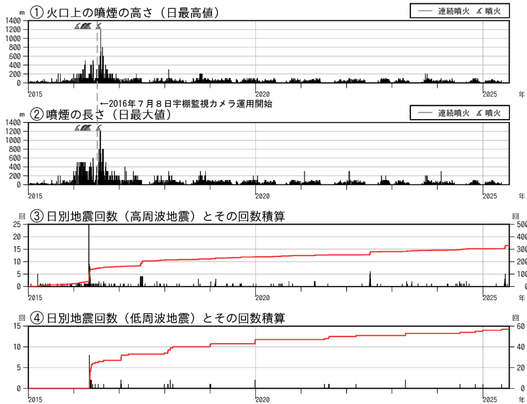
図 3 新潟焼山 火山活動経過図（短期）（2015 年 1 月 1 日～2025 年 7 月 31 日）
