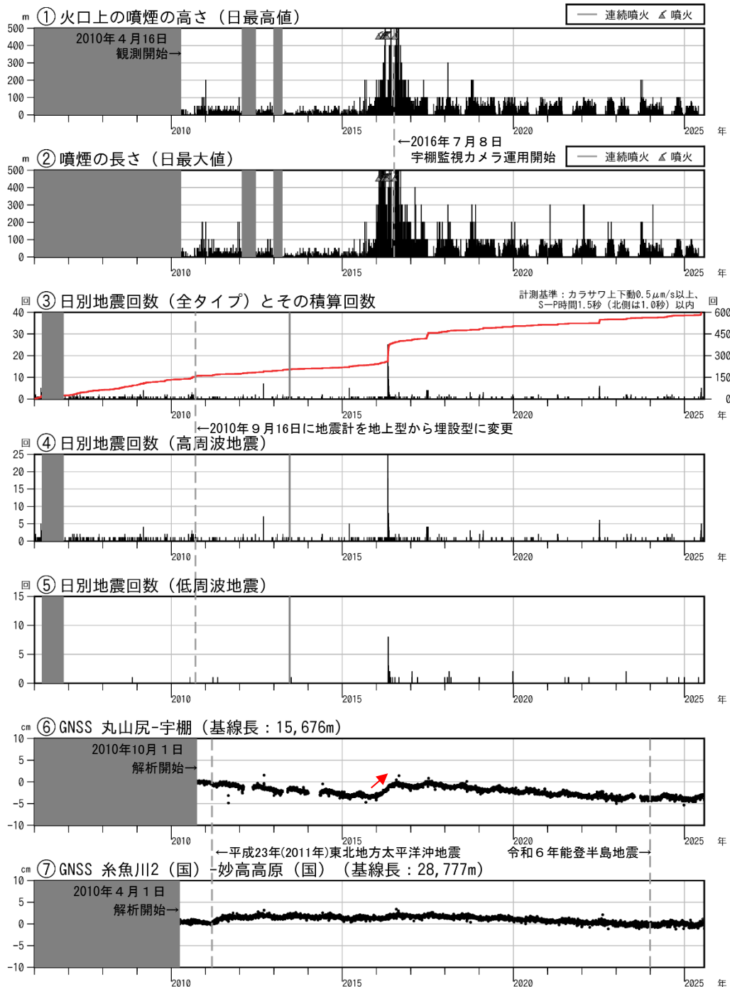
図 2 新潟焼山 火山活動経過図（2006 年 1 月 1 日～2025 年 7 月 31 日）
