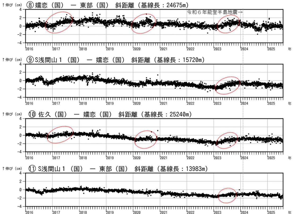
図7-2 浅間山 GNSS 連続観測結果(2016年1月1日～2025年7月31日)
