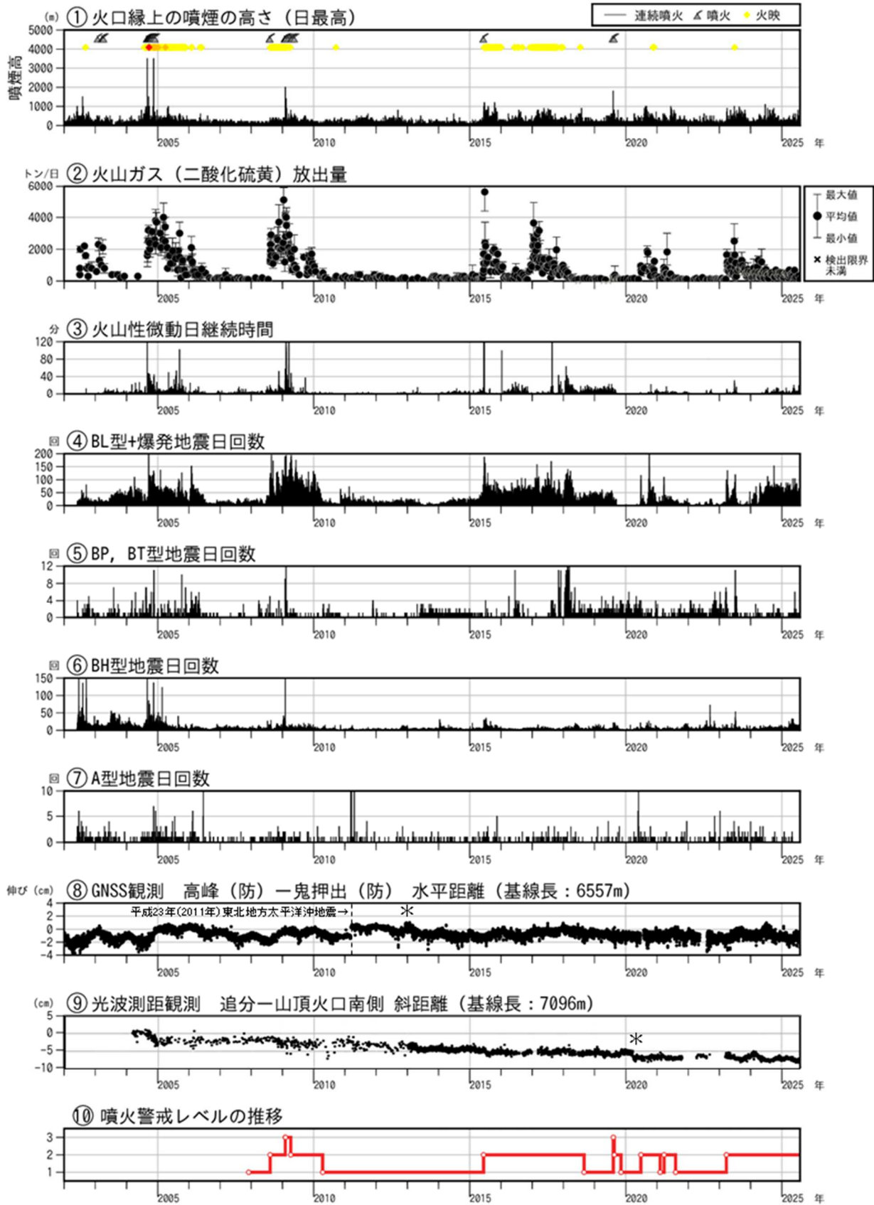
図3 浅間山 長期火山活動経過図（2002年1月1日～2025年7月31日）
