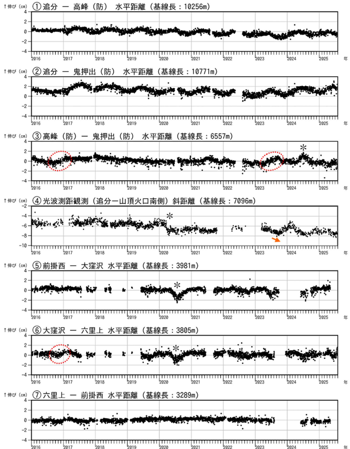
図 7 - 1 浅間山 GNSS 連続観測及び光波測距観測結果 (2016 年 1 月 1 日 ~ 2025 年 7 月 31 日)
