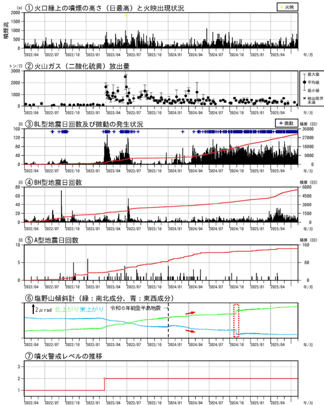
図2 浅間山 短期火山活動経過図（2022年4月1日～2025年7月31日）
