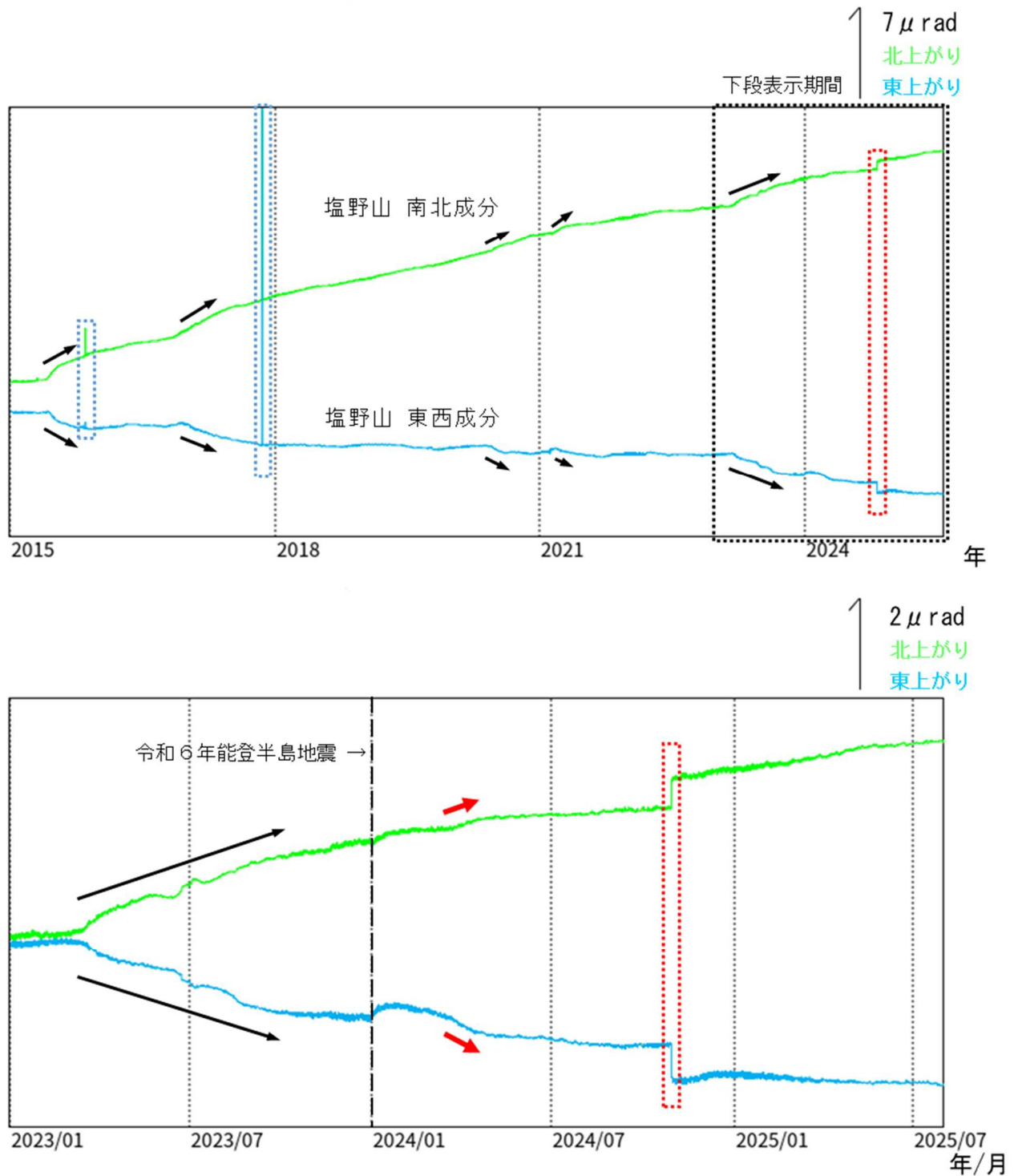
図6 浅間山 塩野山観測点における傾斜データ（2015年1月1日～2025年7月31日）
