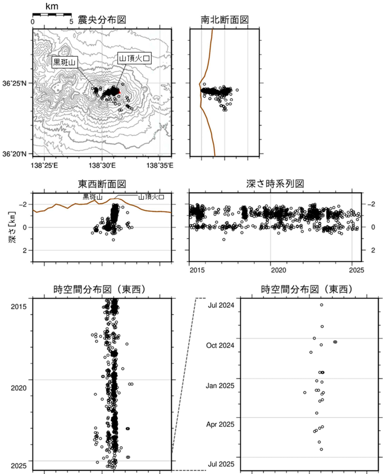
図5 浅間山 震源分布図（2015年1月1日～2025年7月31日）
