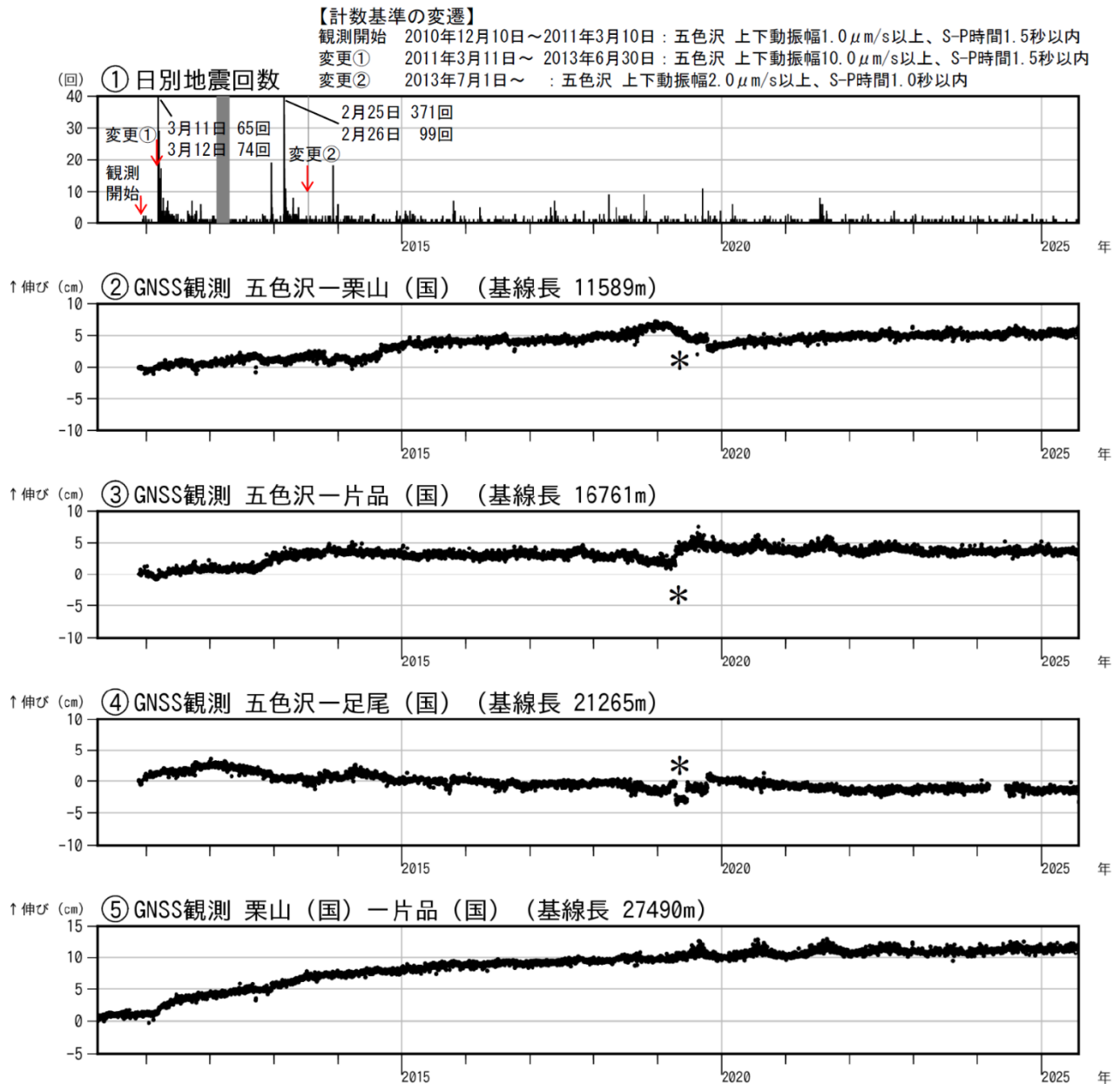
図2 日光白根山 火山活動経過図（2010年4月1日～2025年7月31日）
