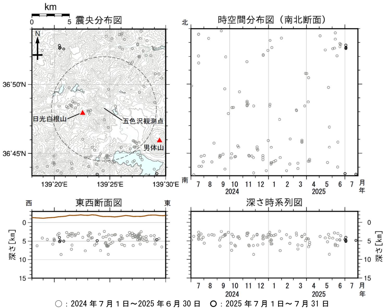
図3 日光白根山 広域地震観測網による山体周辺の地震活動 (2024 年 7 月 1 日～2025 年 7 月 31 日)
