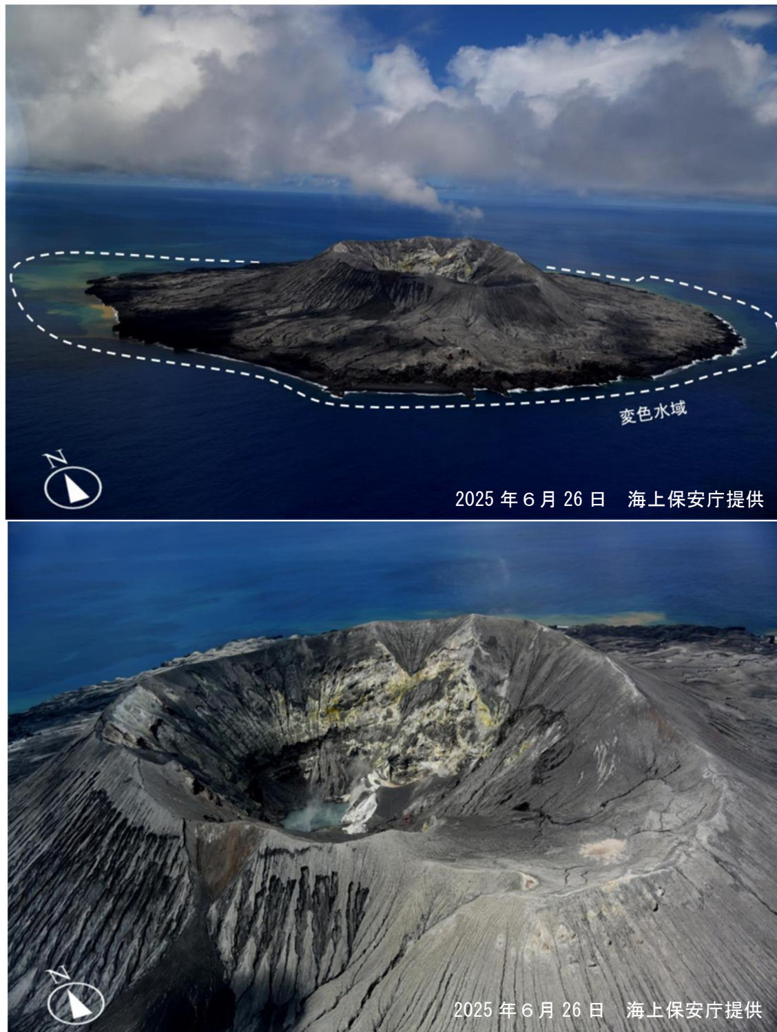
図2 西之島 上空からの観測による西之島の状況（6月26日）
