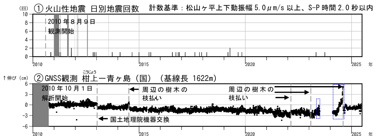
図3 青ヶ島 火山活動経過図（2010年8月9日～2025年6月30日） ① グラフの灰色部分は機器障害による欠測を示す。 ② （国）：国土地理院、図4のGNSS基線②に対応。グラフの空白部分は柑上の障害による欠測を示す。 ・青破線で囲んだ変化は柑上観測点周囲の樹木による影響と考えています。
