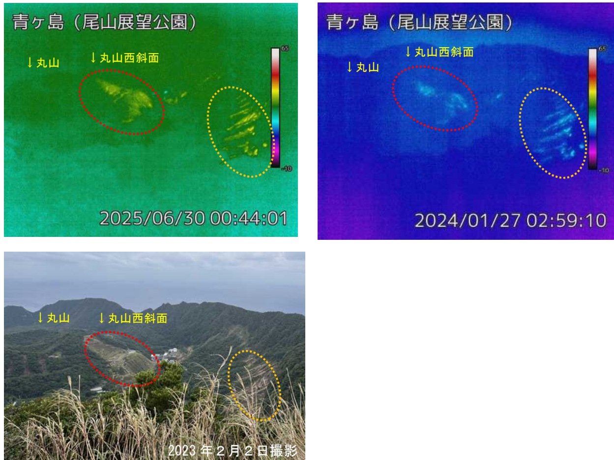
図2 青ヶ島 カルデラ内の地表面温度の状況（左上, 右上：尾山展望公園監視カメラによる、 下：2023年2月2日に撮影した同場所からの写真） ・地熱活動（赤点線及び黄色点線で示した範囲）に変化は認められません。
