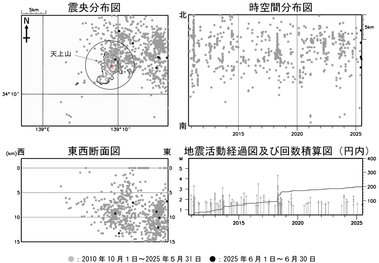
図3 神津島 広域地震観測網による山体・周辺の地震活動（2010年10月1日～2025年6月30日） 広域地震観測網により震源決定したもので、深さは全て海面以下として決定しています。なお、2020年9月以降については、地震観測点の標高を考慮する等、震源決定の手法を変更しています。 M（マグニチュード）は地震の規模を表し、M1.4以上の地震を示しています。 図中の震源要素は一部暫定値が含まれており、後日変更することがあります。 計数対象（天上山西から半径約5km、深さ約15km以内）以外の地震が含まれるため、図2-①の日別地震回数（高周波地震）とは異なります。 震央分布図中の円は火山性地震の回数の計数対象（天上山西から半径5km、深さ15km以内）の範囲を示しています。 ・地震活動は低調に経過しました。
