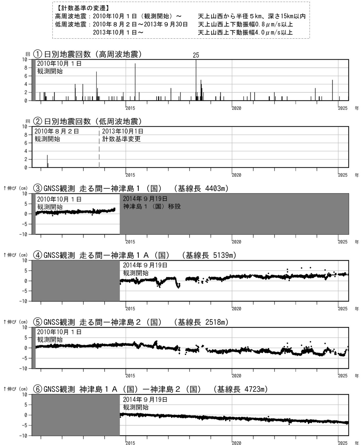
図2 神津島 火山活動経過図(2010年8月2日～2025年6月30日)
