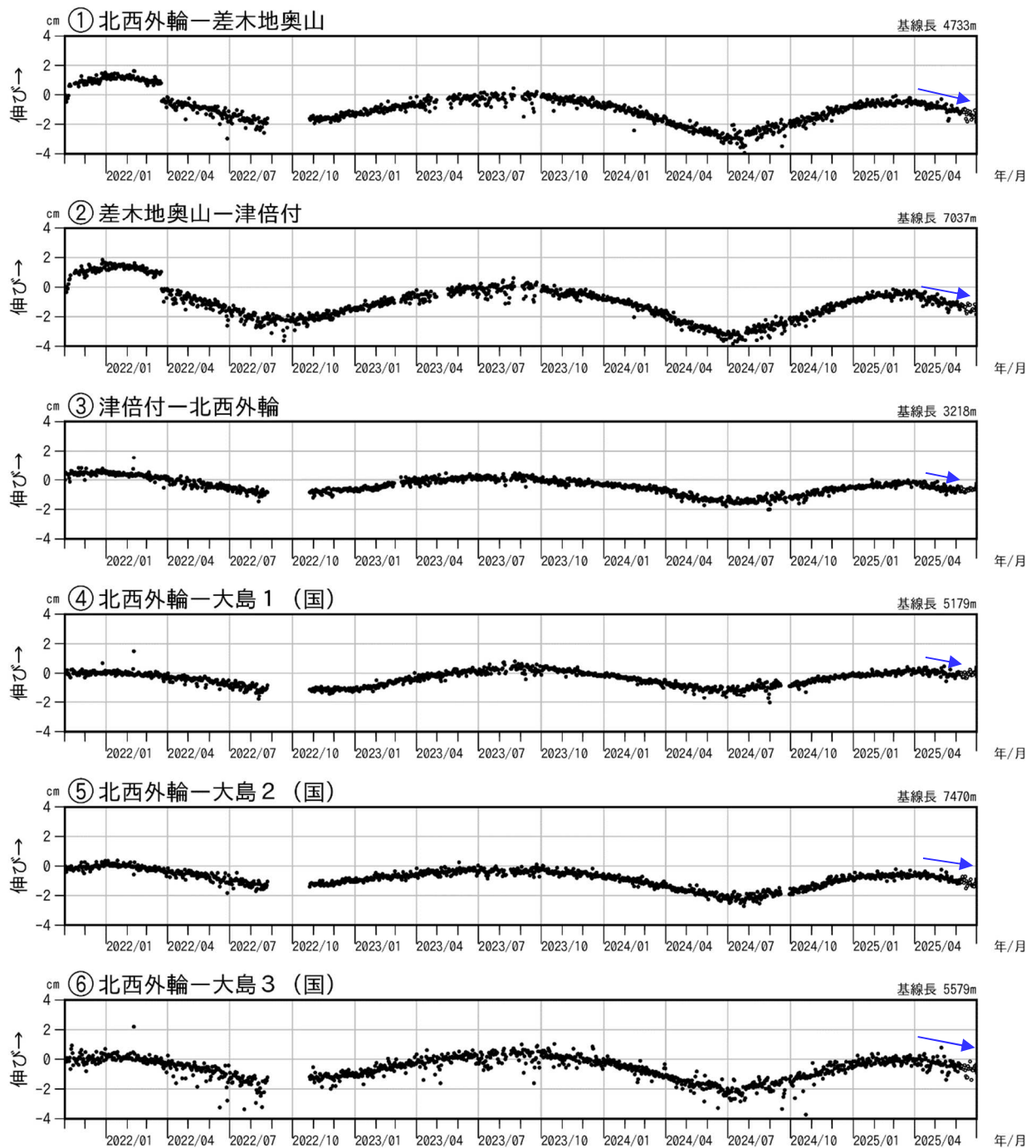
図3-2 伊豆大島 GNSS 連続観測による基線長変化(2021年10月～2025年6月30日)
