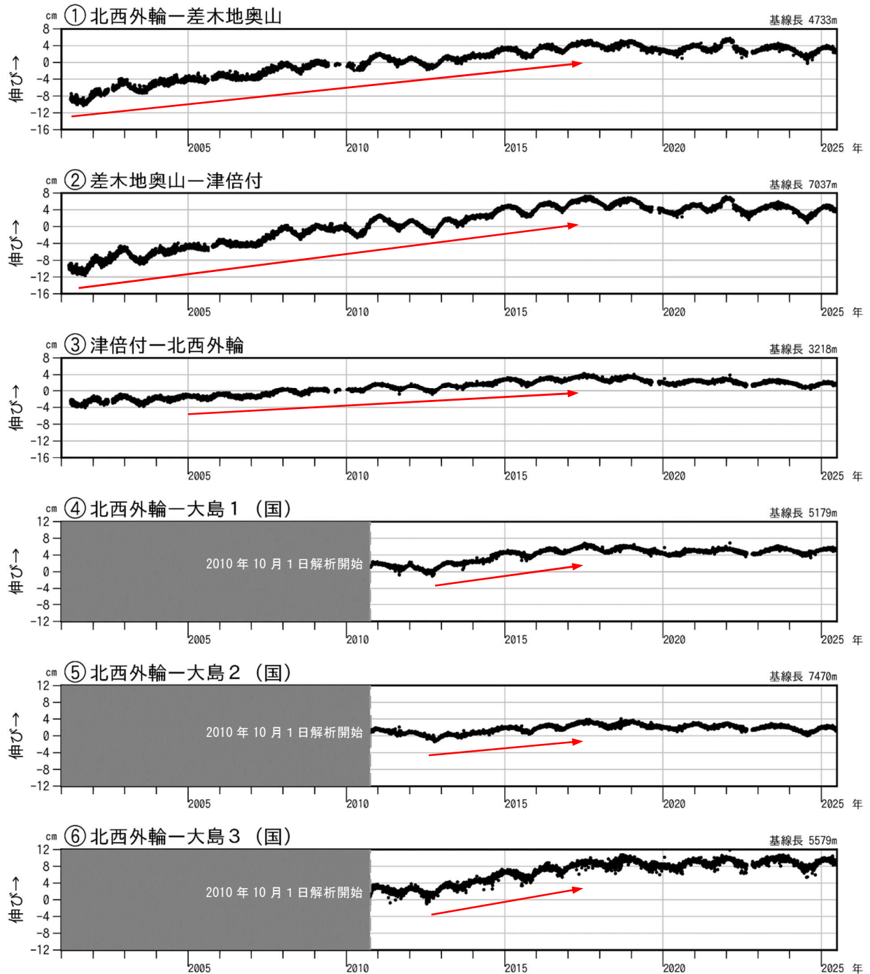
図3-1 伊豆大島 GNSS連続観測による基線長変化(2001年1月～2025年6月30日)
