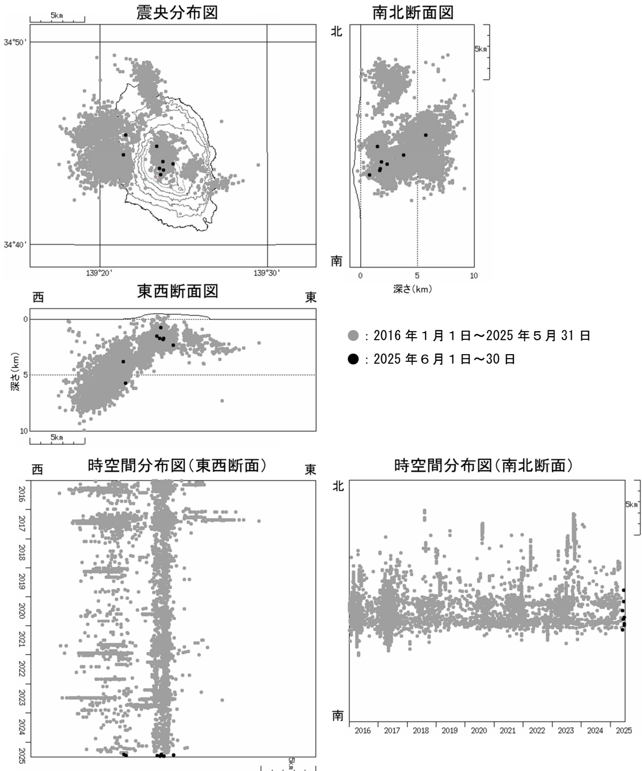
図4 伊豆大島 震源分布図（2016 年 1 月 1 日～2025 年 6 月 30 日）
