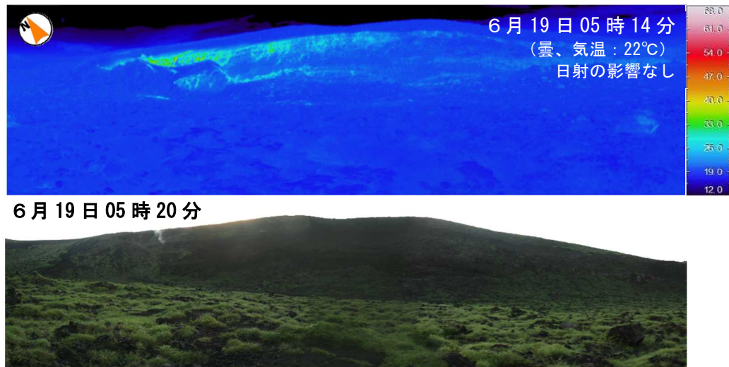
図7-2 伊豆大島 剣ガ峰の状況（撮影方向は図8参照）
