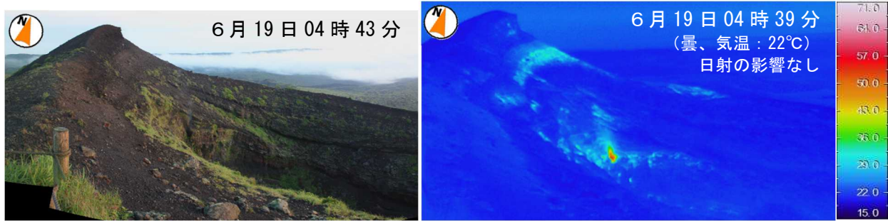
図7-1 伊豆大島 B2 火孔周辺の状況（撮影方向は図8参照）
