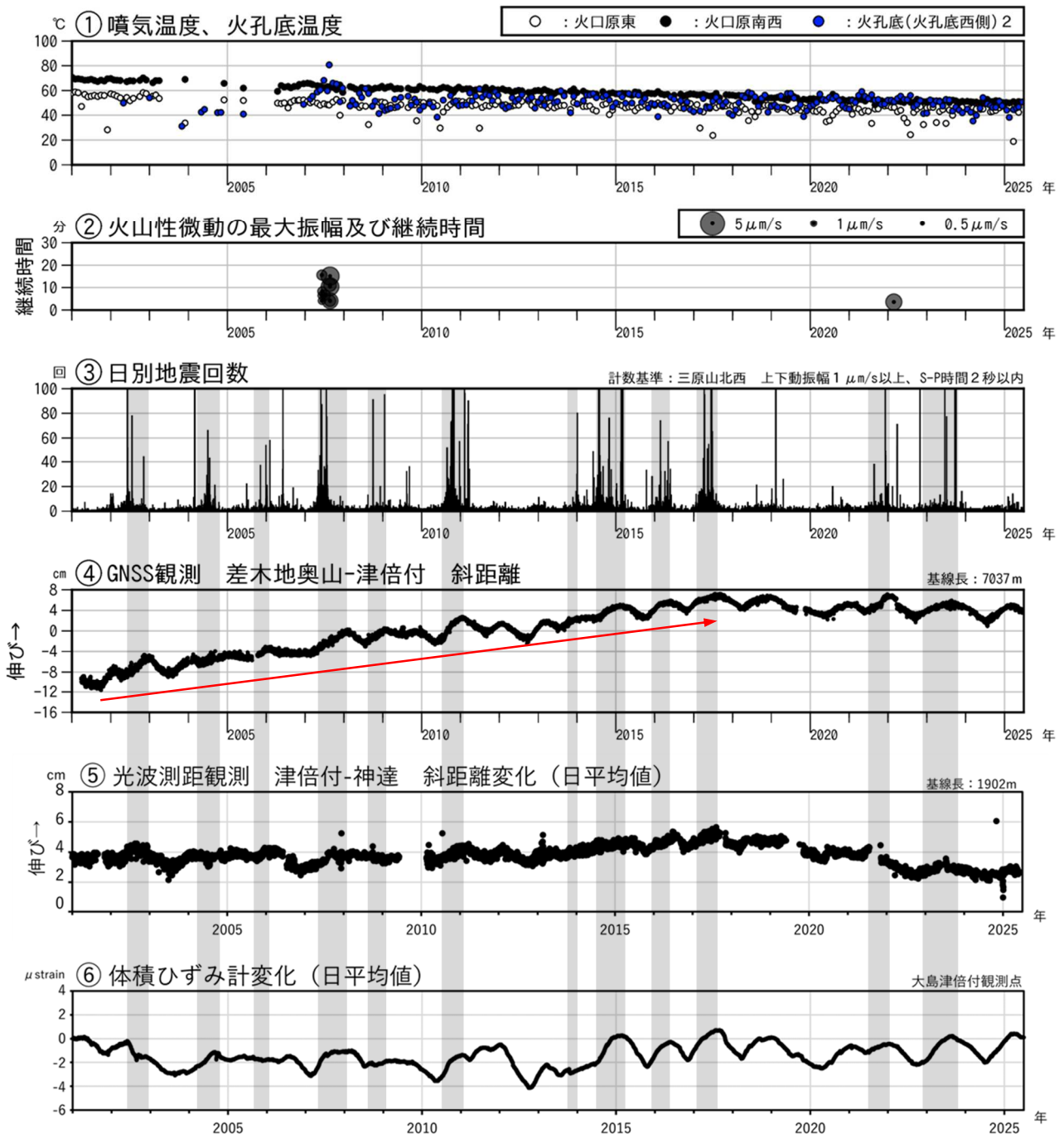
図2 伊豆大島 最近の火山活動経過図(2001年1月～2025年6月30日)
