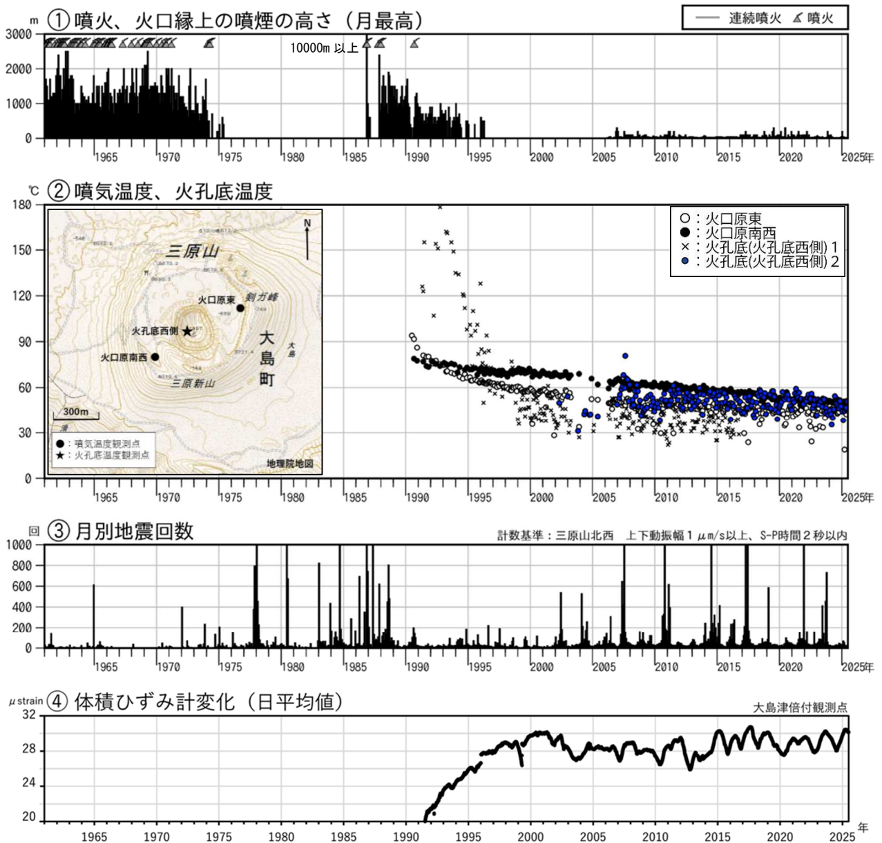
図1 伊豆大島 長期間の火山活動経過図（1961年1月～2025年6月30日）
