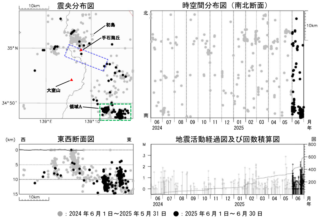
図2 伊豆東部火山群 広域地震観測網による震源分布図（2024 年 6 月 1 日～2025 年 6 月 30 日） □ の領域は群発地震活動の発生する可能性がある範囲（火口が出現する可能性のある範囲）を示しています。 https://www.data.jma.go.jp/vois/data/filing/level/PDF/level_316.pdf 広域地震観測網により震源決定したもので、深さは全て海面以下として決定しています。 M（マグニチュード）は地震の規模を表し、M0.0 以上を表示しています。 図中の震源要素は一部暫定値が含まれており、後日変更することがあります。 この図では、関係機関の地震波形を一元的に処理し、地震観測点の標高を考慮する等した手法で得られた震源を用いています。
