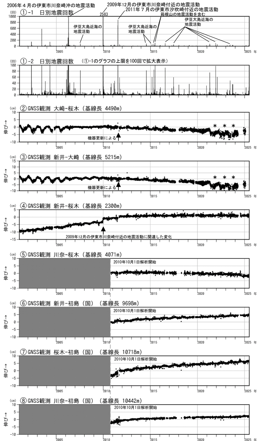
図3 伊豆東部火山群 火山活動経過図（2001年2月1日～2025年6月30日）
