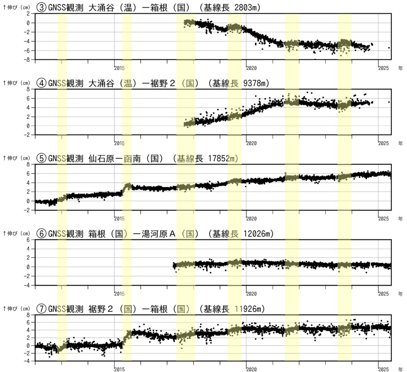
図3－2 箱根山 GNSS連続観測による 基線長変化及び観測点配置図 (2012年1月1日～2025年6月30日) (国)：国土地理院 (温)：神奈川県温泉地学研究所 空白部分は欠測を示します。 システム更新に伴う調整中のため、一部の過去データにステップ状の変化がみられています。
