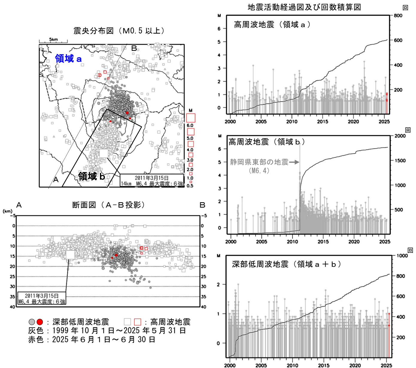
図3 富士山 広域地震観測網による山体及び周辺の地震活動（1999年10月1日～2025年6月30日）
