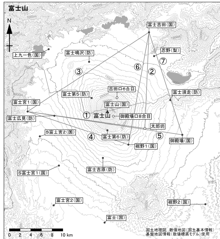
図5 富士山 GNSS 観測点配置図
