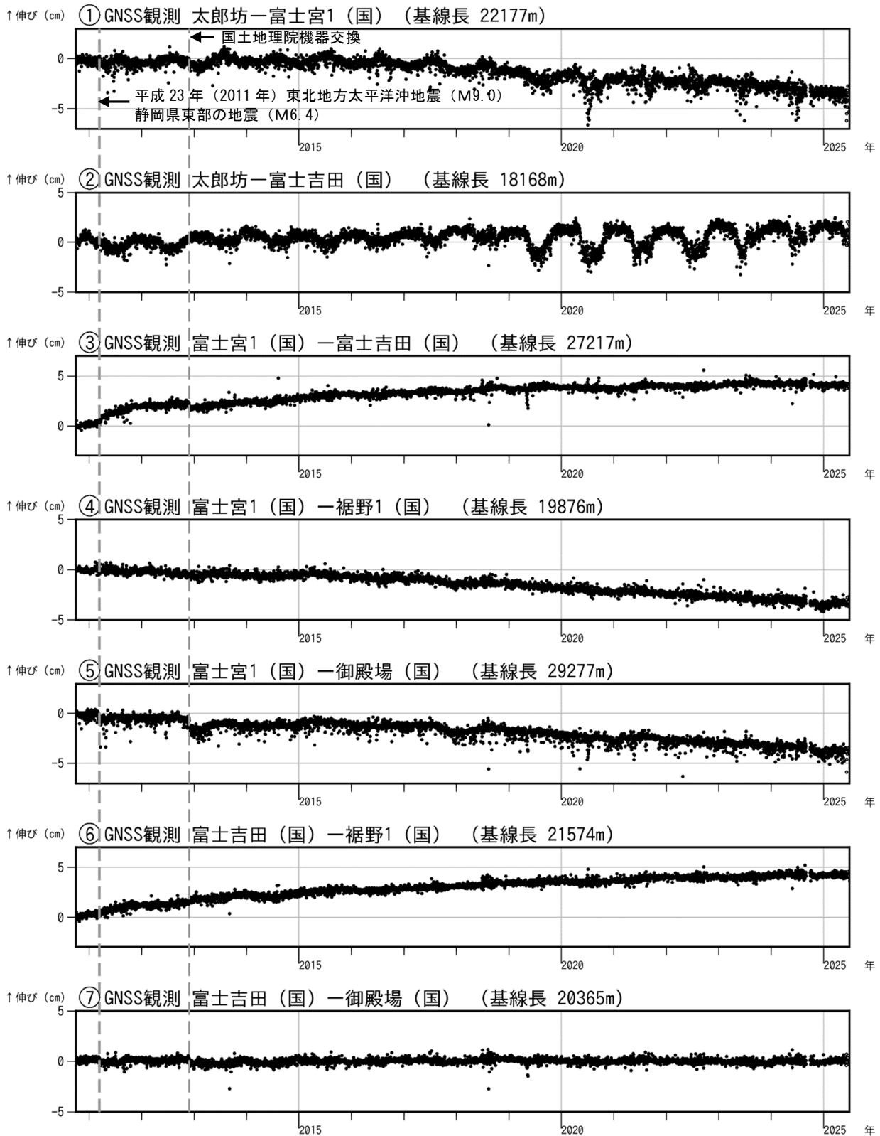
図4 富士山 GNSS 連続観測による基線長変化 (2010 年 10 月 1 日～2025 年 6 月 30 日)
