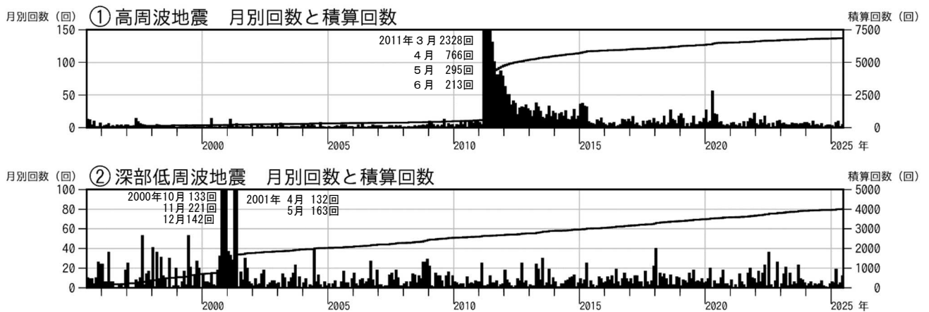
図2 富士山 月別地震回数（1995年6月1日～2025年6月30日）
